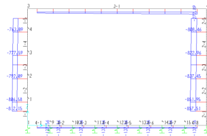
Fig. 6 – Involuppo azioni assiali SLU
