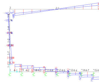
Fig. 5 – Involuppo sforzi taglienti SLU
