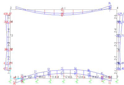
Fig. 4 – Involuppo momenti flettenti SLU
