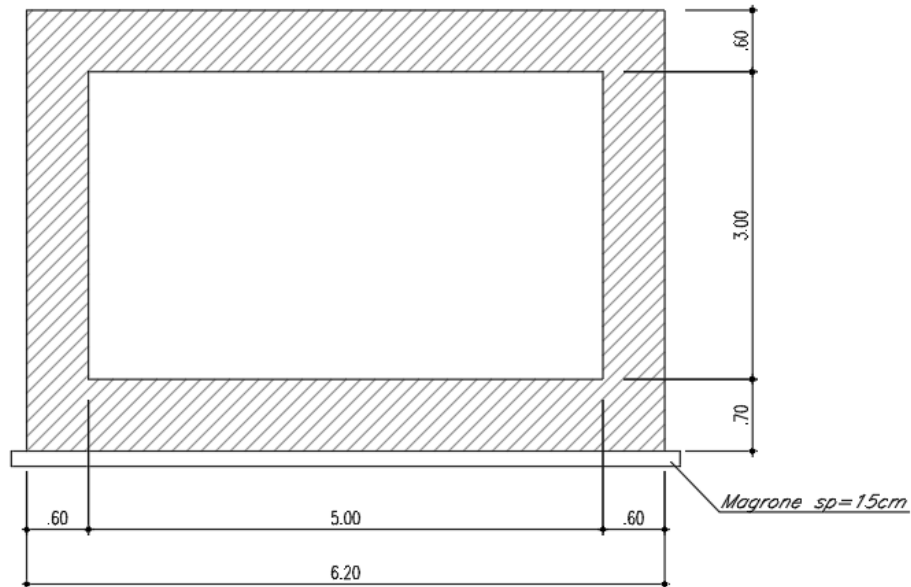
Fig. 1 – Sezione trasversale dell'opera
