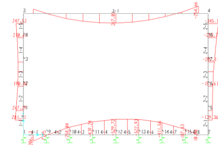
Fig. 10 – Inviluppo momenti flettenti SLE rara
