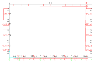
Fig. 11 – Inviluppo azioni assiali SLE rara
