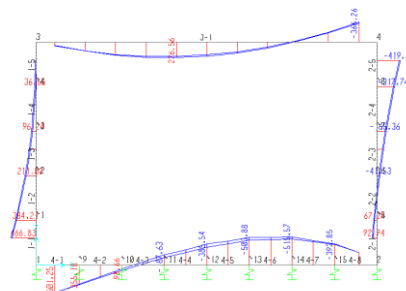
Fig. 7 –Involuppo momenti flettenti SLV
