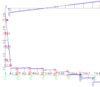
Fig. 8 – Inviluppo sforzi taglienti SLV
