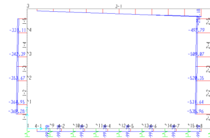
Fig. 9 – Inviluppo azioni assiali SLV
