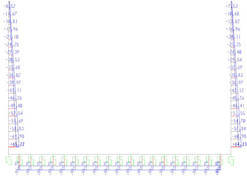
Fig. 5 – Involuppo azioni assiali SLU
