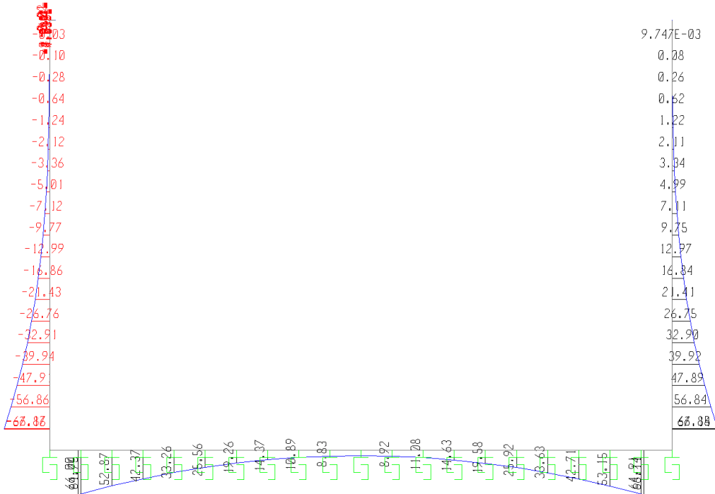
Fig. 9 – Involuppo momenti flettenti SLE rara
