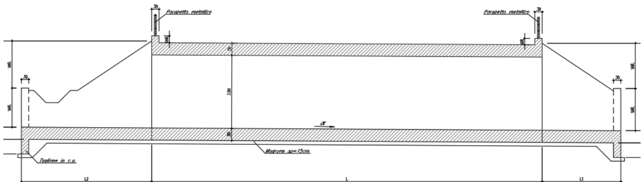
Fig. 2 –Sezione longitudinale
