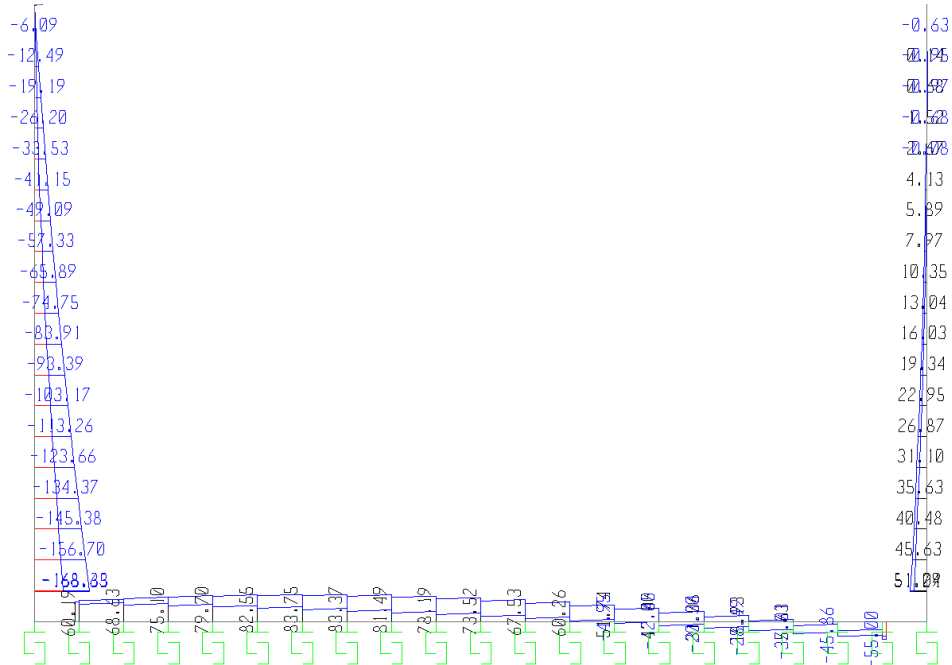
Fig. 7 – Involuppo sforzi taglienti SLV
