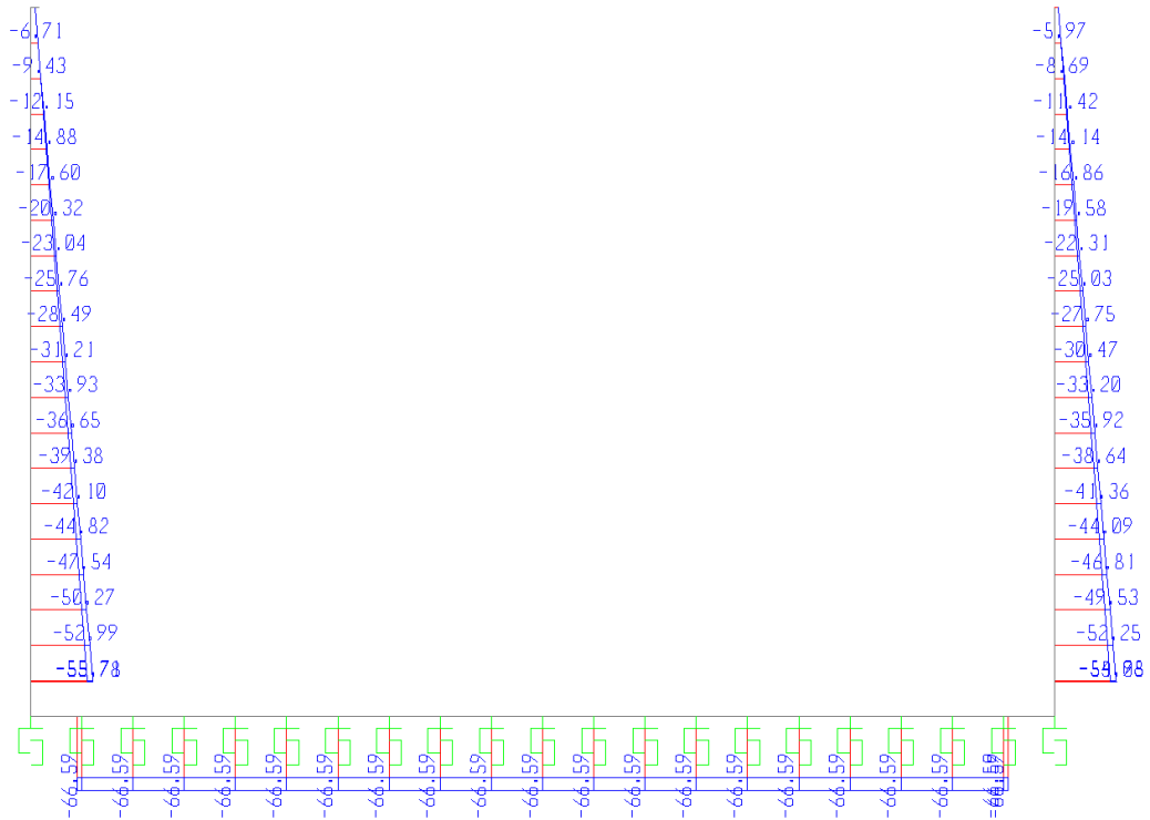
Fig. 8 – Involuppo azioni assiali SLV
