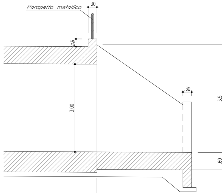
Fig. 1 –Sezione longitudinale
