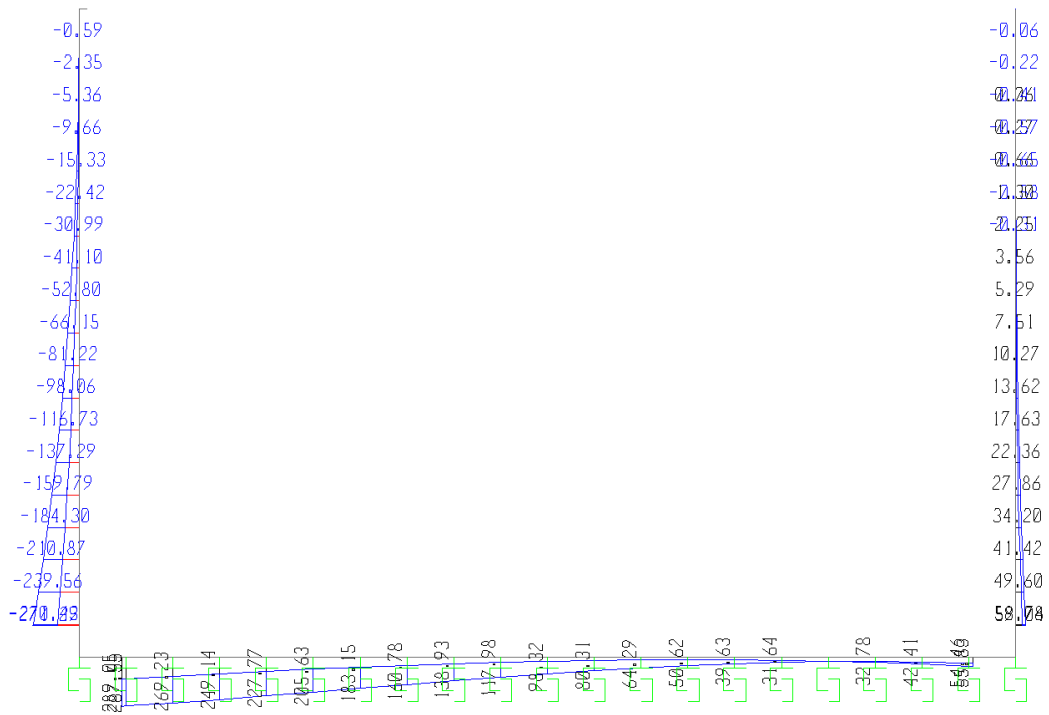
Fig. 6 – Involuppo momenti flettenti SLV
