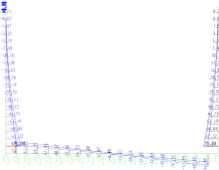
Fig. 4 – Involuppo sforzi taglienti SLU
