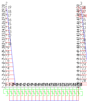
Fig. 11 – Involuppo azioni assiali SLE rara
