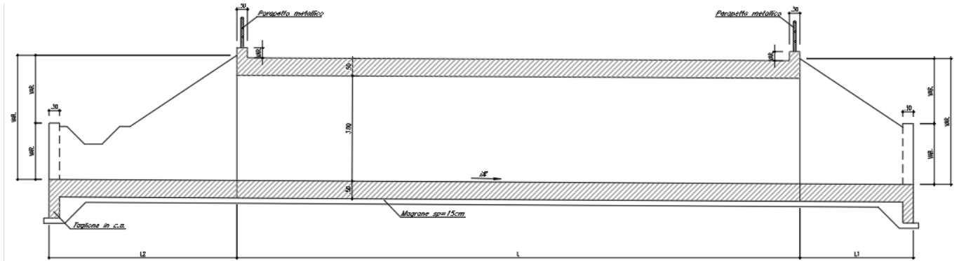
Fig. 2 –Sezione longitudinale
