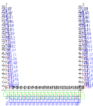
Fig. 6 – Involuppo azioni assiali SLU
