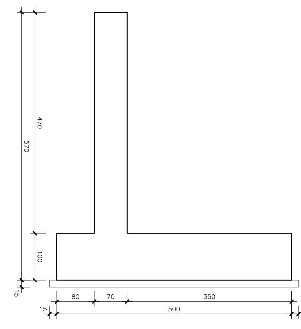
SEZIONE MURO TIPO "D" - Scala 1:50
