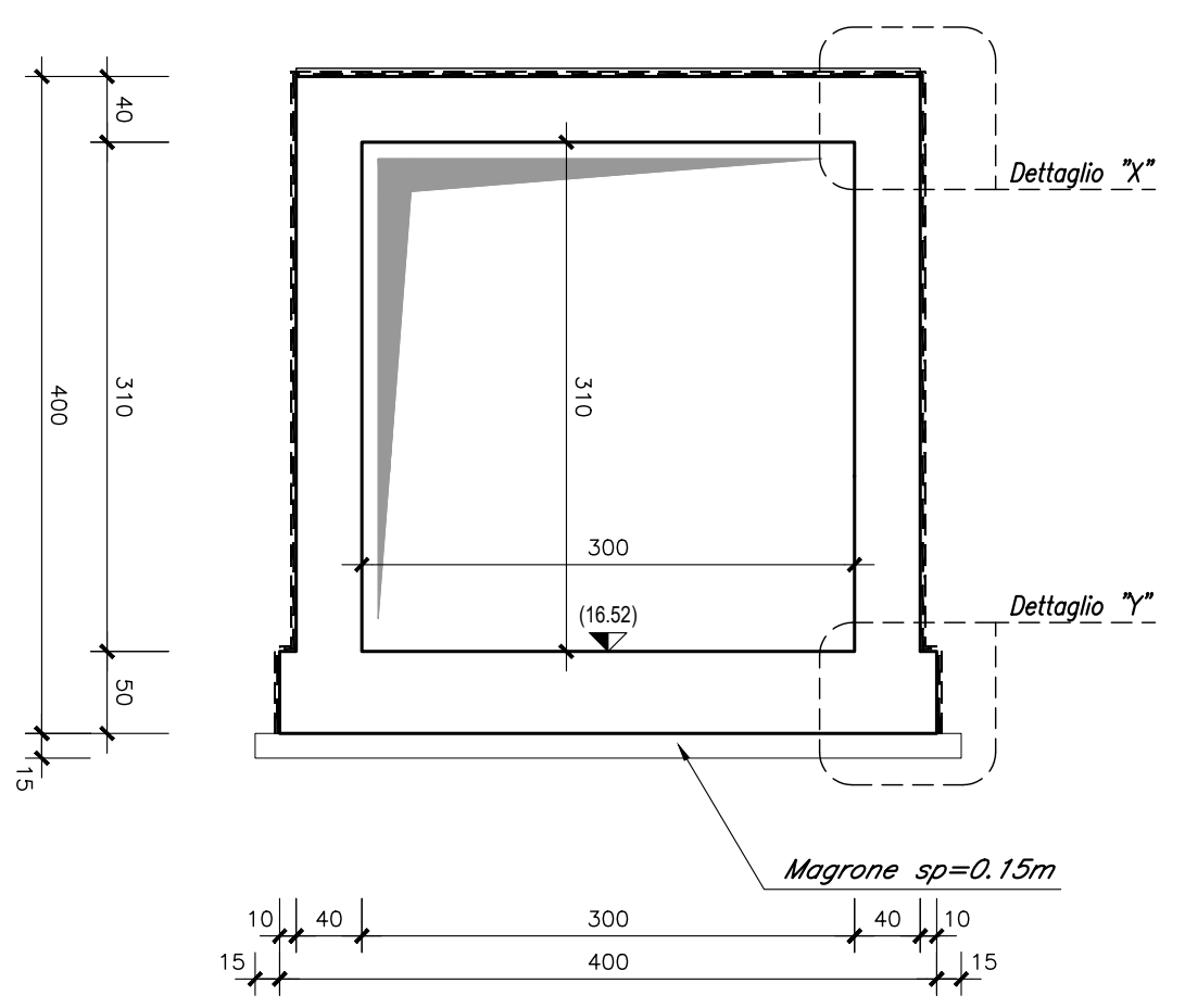
SEZIONE B-B-Scala 1:50
