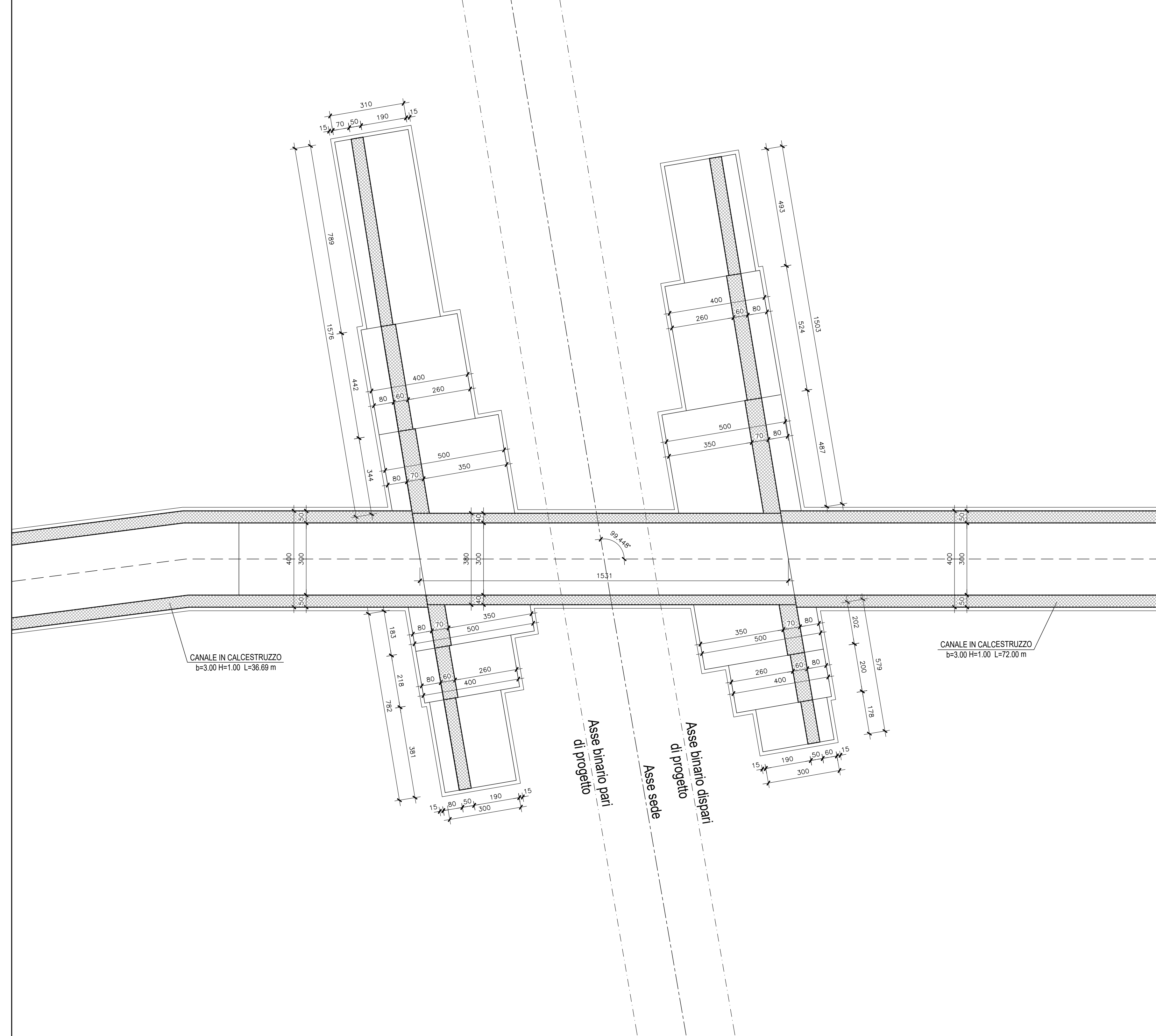
PIANTA ALLO SPICCATO-Scala 1:100
