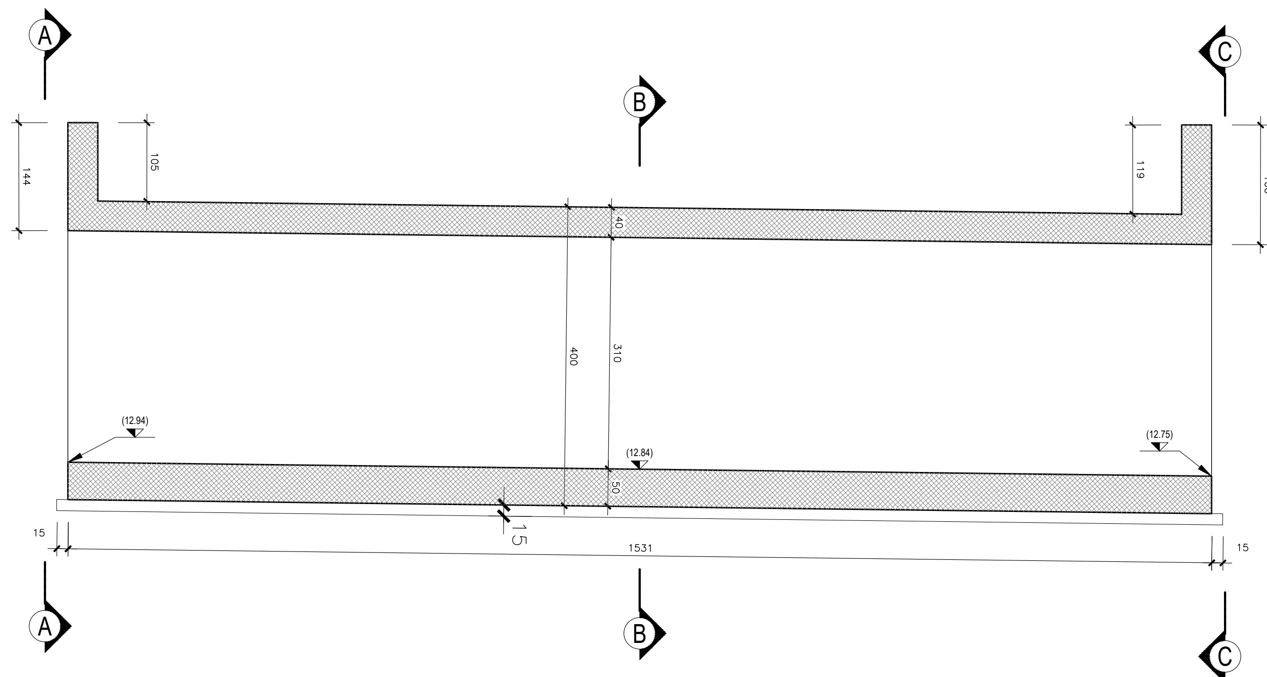
SEZIONE LONGITUDINALE-Scala 1:50
