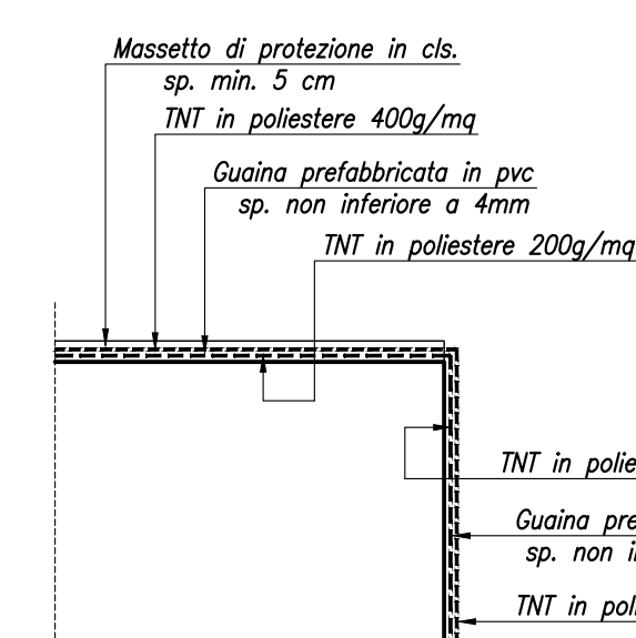
DETTAGLIO "X"-Scala 1:20
