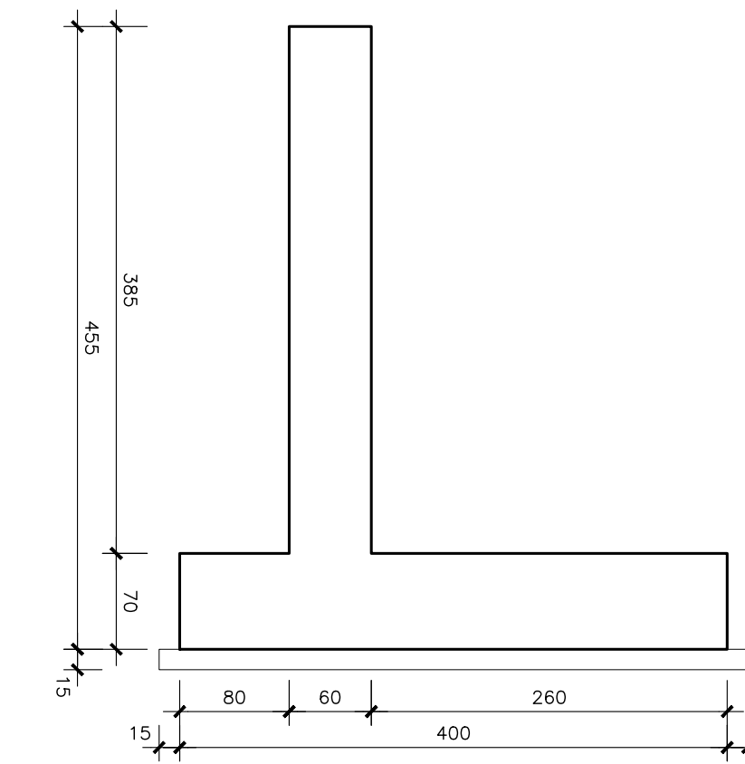
SEZIONE MURO TIPO "B" - Scala 1:50
