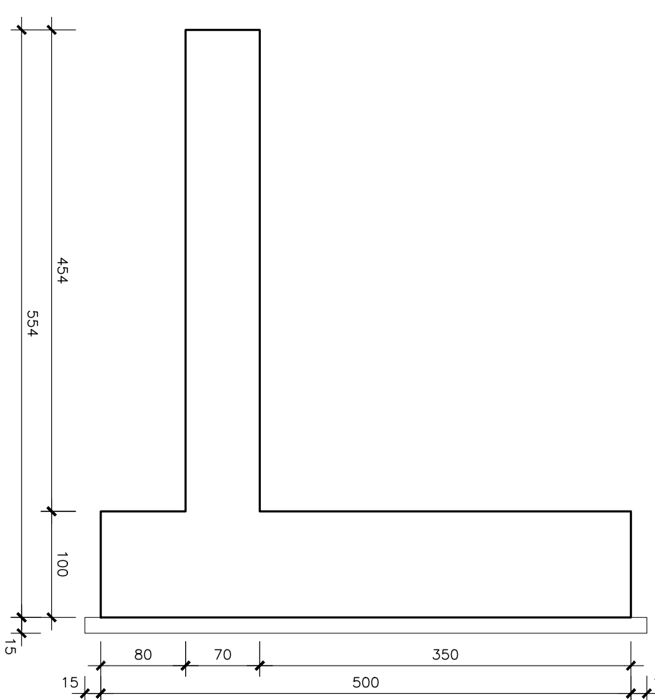
SEZIONE MURO TIPO "C" - Scala 1:50
