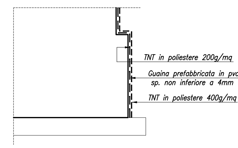
DETTAGLIO "Y"-Scala 1:20
