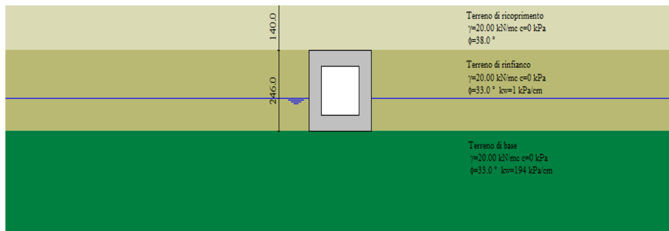
Modello Geometrico Geotecnico di Riferimento – 1/2
