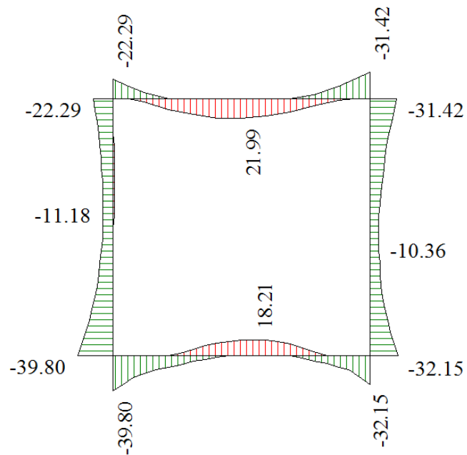
Inviluppo diagrammi del momento flettente – SLE
