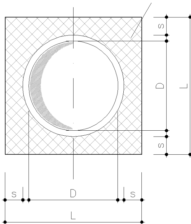
Figura 2 – Sezione trasversale tipo
