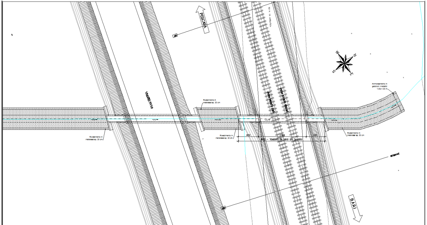
Figura 1 – Inquadramento planimetrico
