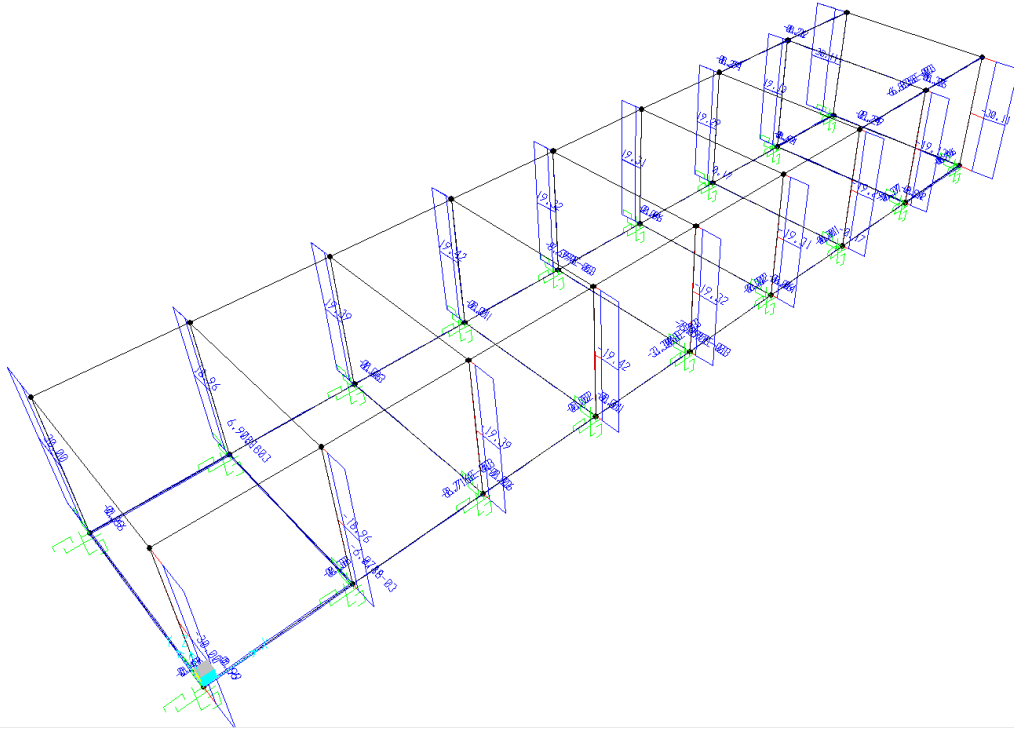
Taglio V3 - Involuppo SLV
