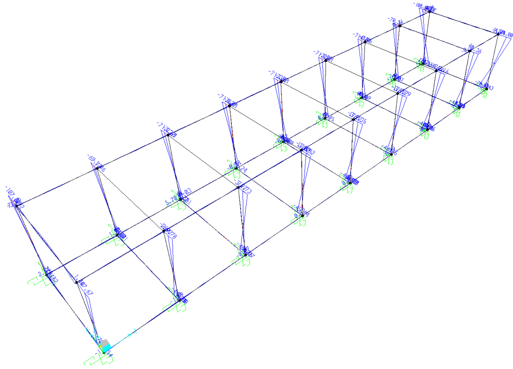
Momento M2 - Involuppo SLU
