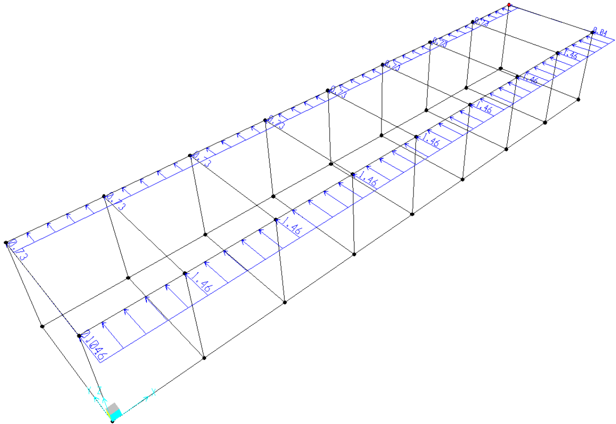
Vy+ – Vento Y+
