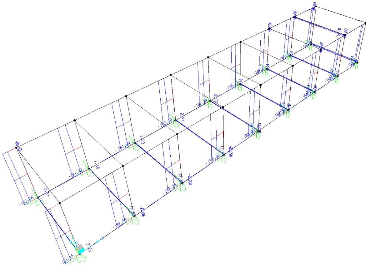
Sforzo Normale N - Involuppo SLER
