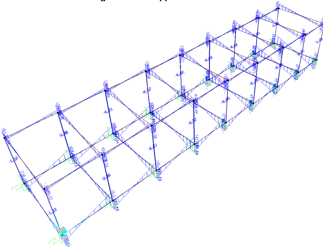
Taglio V2 - Involuppo SLV
