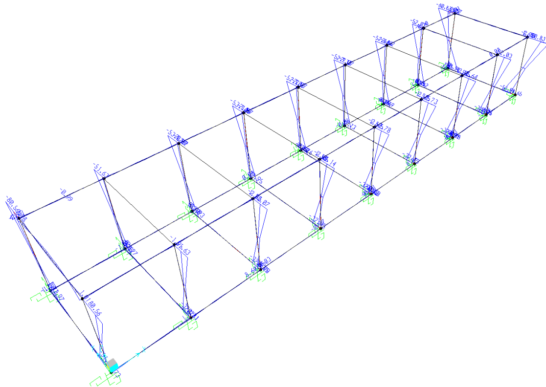
Momento M2 - Involuppo SLER
