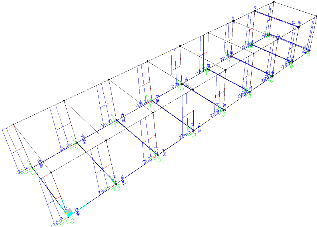
Sforzo Normale N - Involuppo SLV
