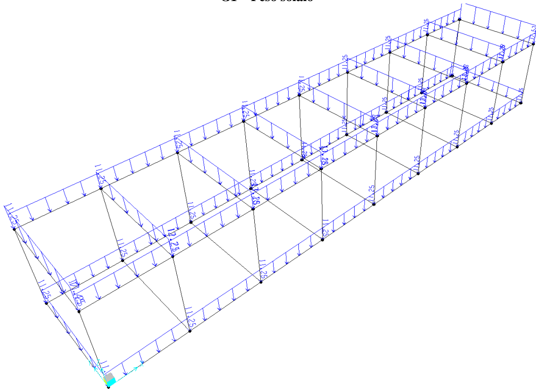
G2 – Permanenti non strutturali
