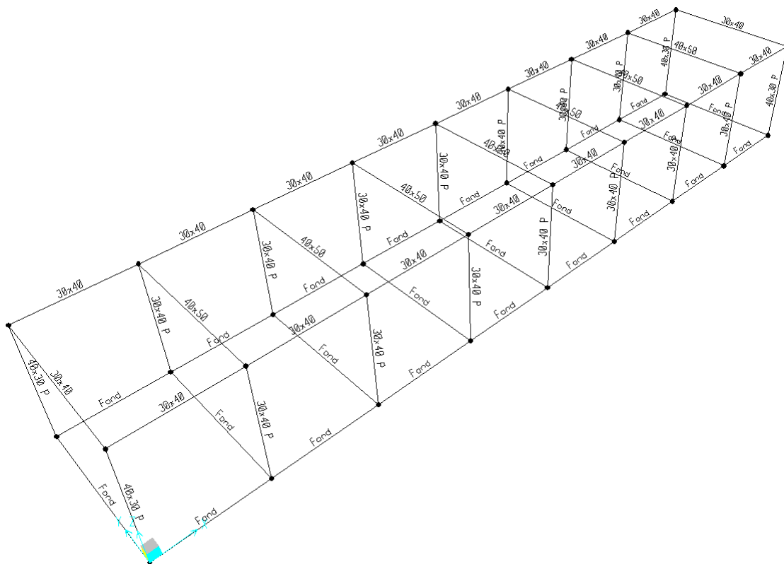
Figura 2: tipologia aste
