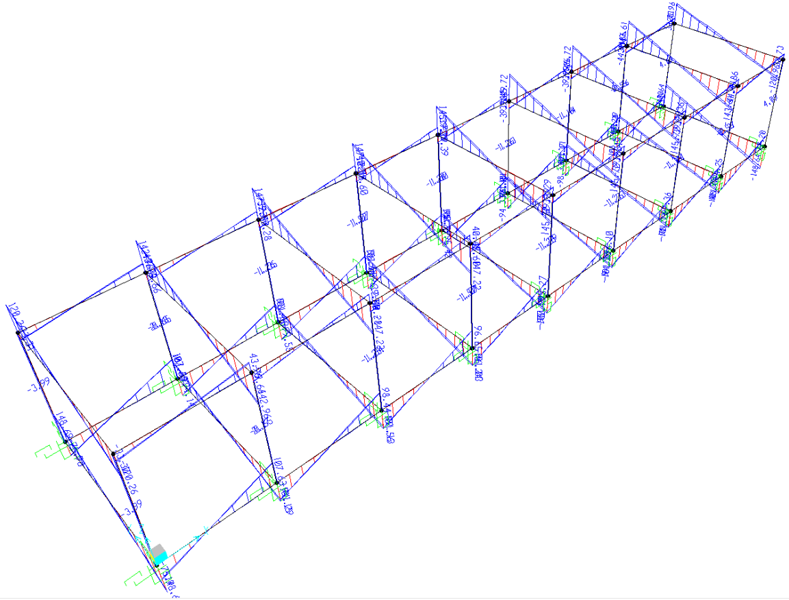
Taglio V2 - Involuppo SLU
