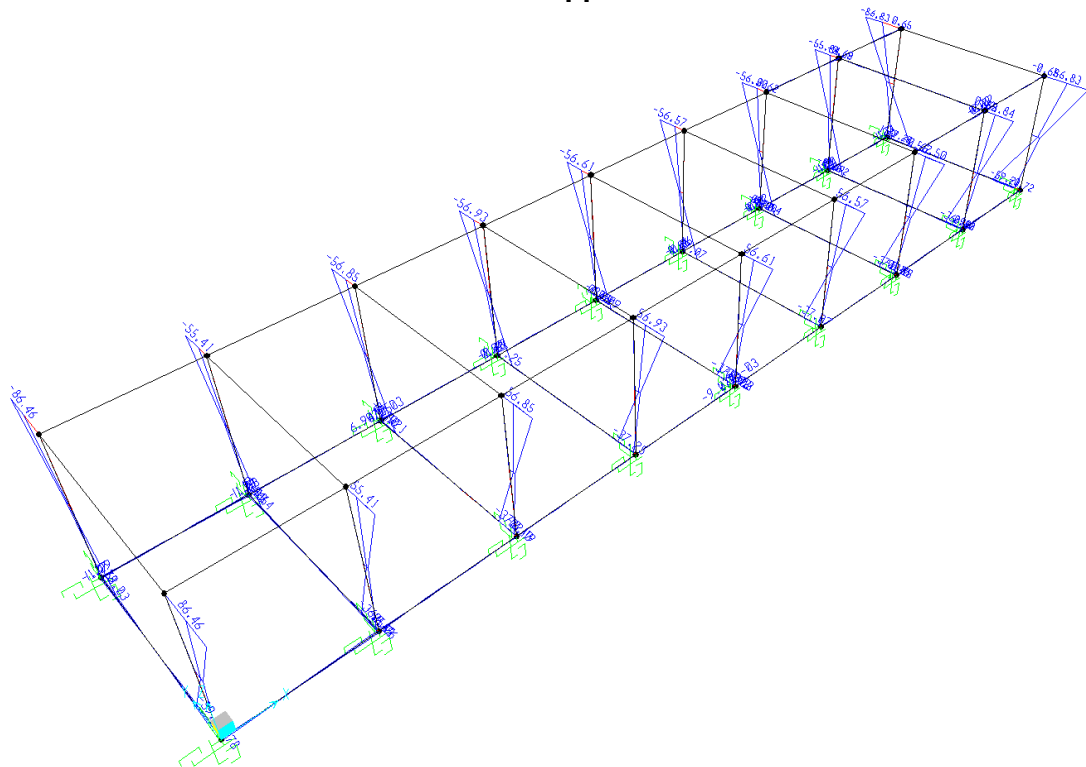
Momento M2 - Involuppo SLV
