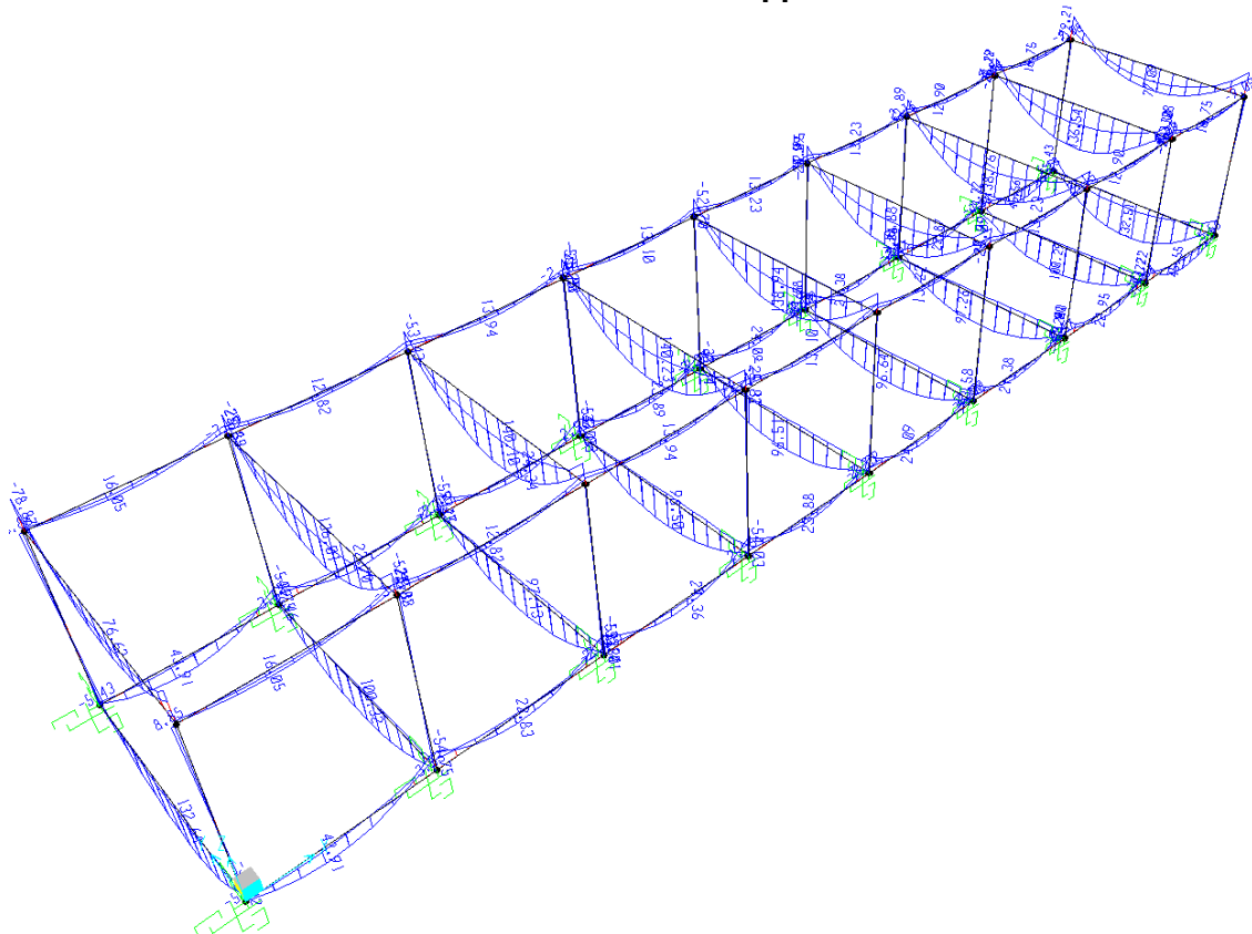
Momento M3 - Involuppo SLER
