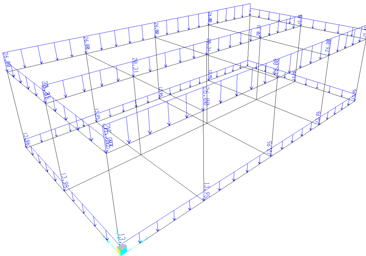
G2 – Permanenti non strutturali
