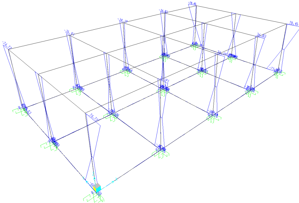
Momento M2 - Inviluppo SLV
