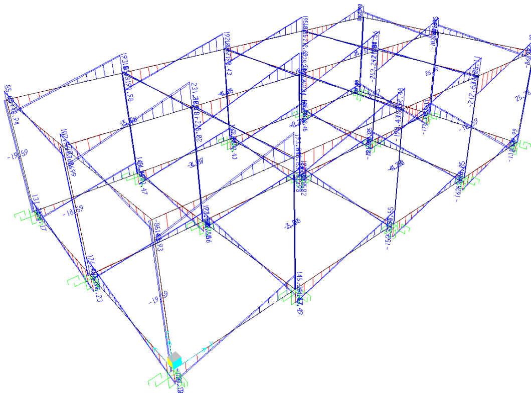
Taglio V2 - Involuppo SLU
