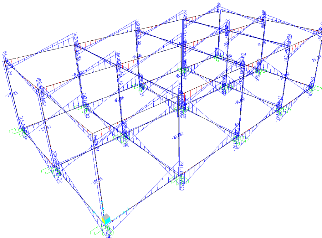
Taglio V2 - Involuppo SLV
