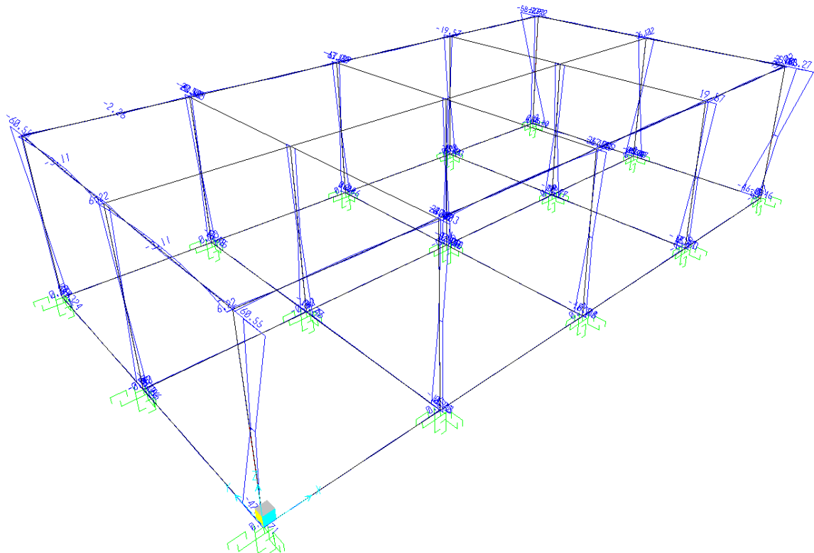
Momento M2 - Involuppo SLER
