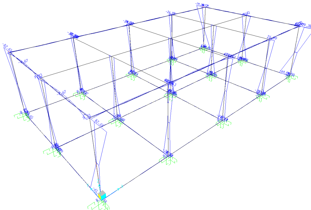
Momento M2 - Involuppo SLU
