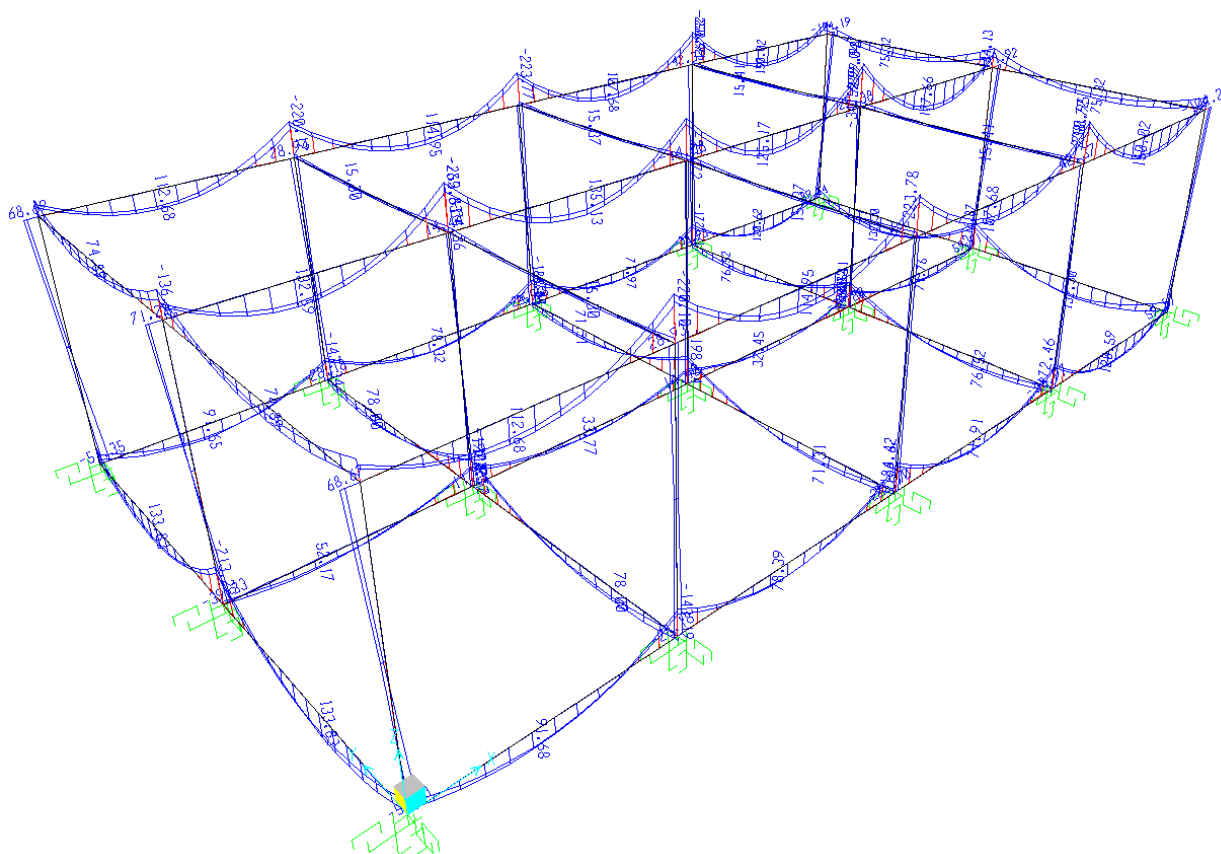
Momento M3 - Involuppo SLU
