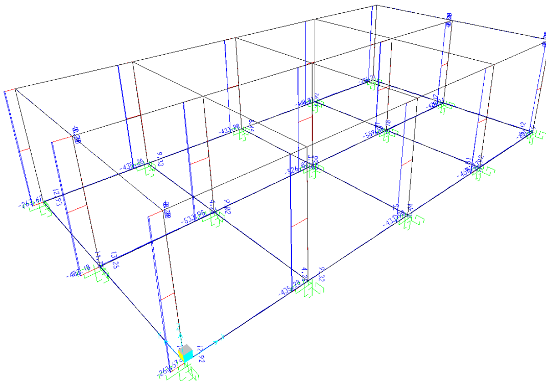
Sforzo Normale N - Involuppo SLU
