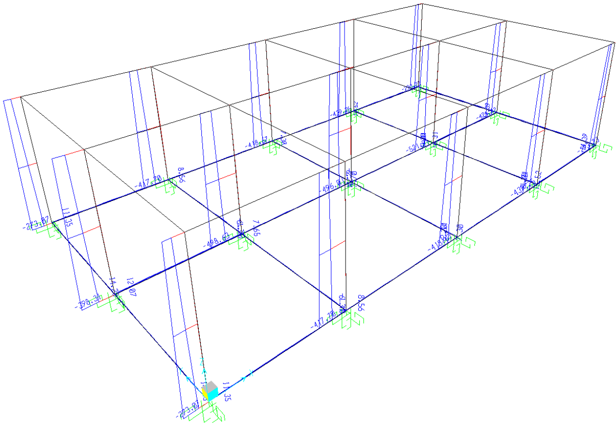
Sforzo Normale N - Involuppo SLV
