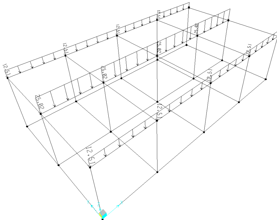
G1 – Peso solaio
