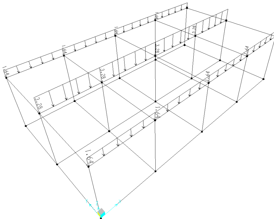
Q H1 – Accidentali (Manutenzione)
