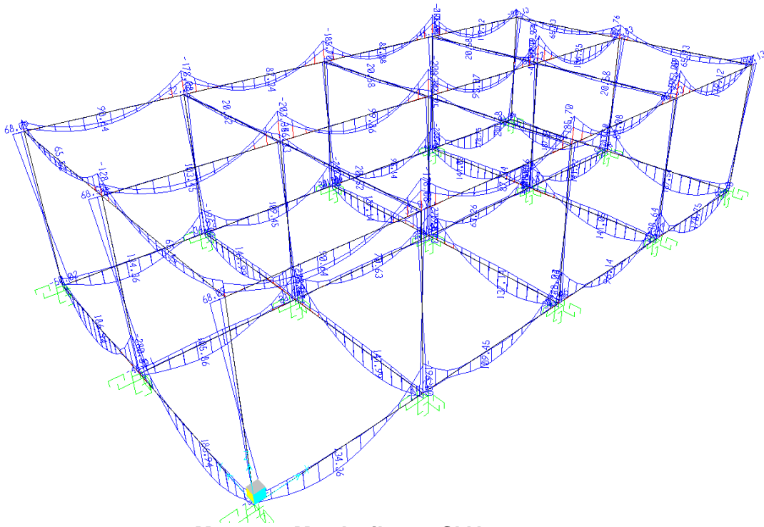
Momento M3 - Inviluppo SLV
