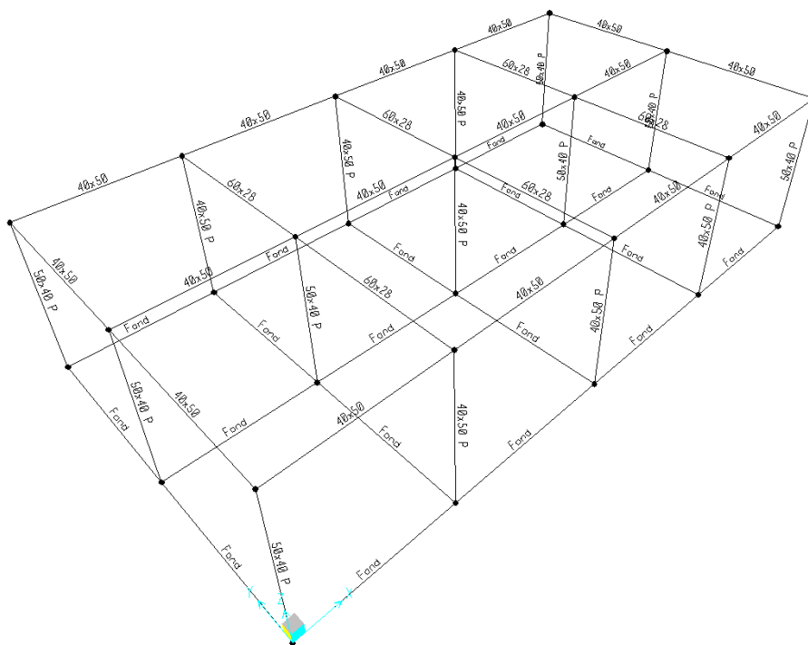
Figura 2: tipologia aste
