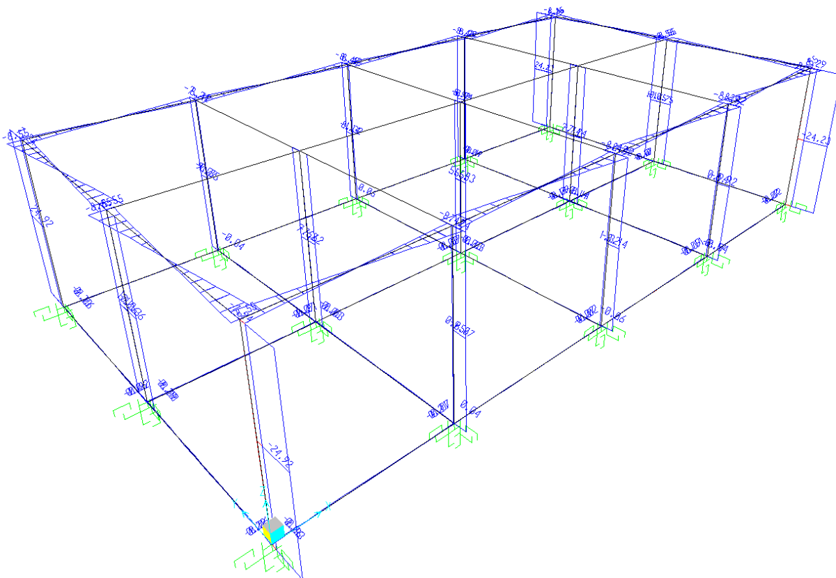
Taglio V3 - Involuppo SLU
