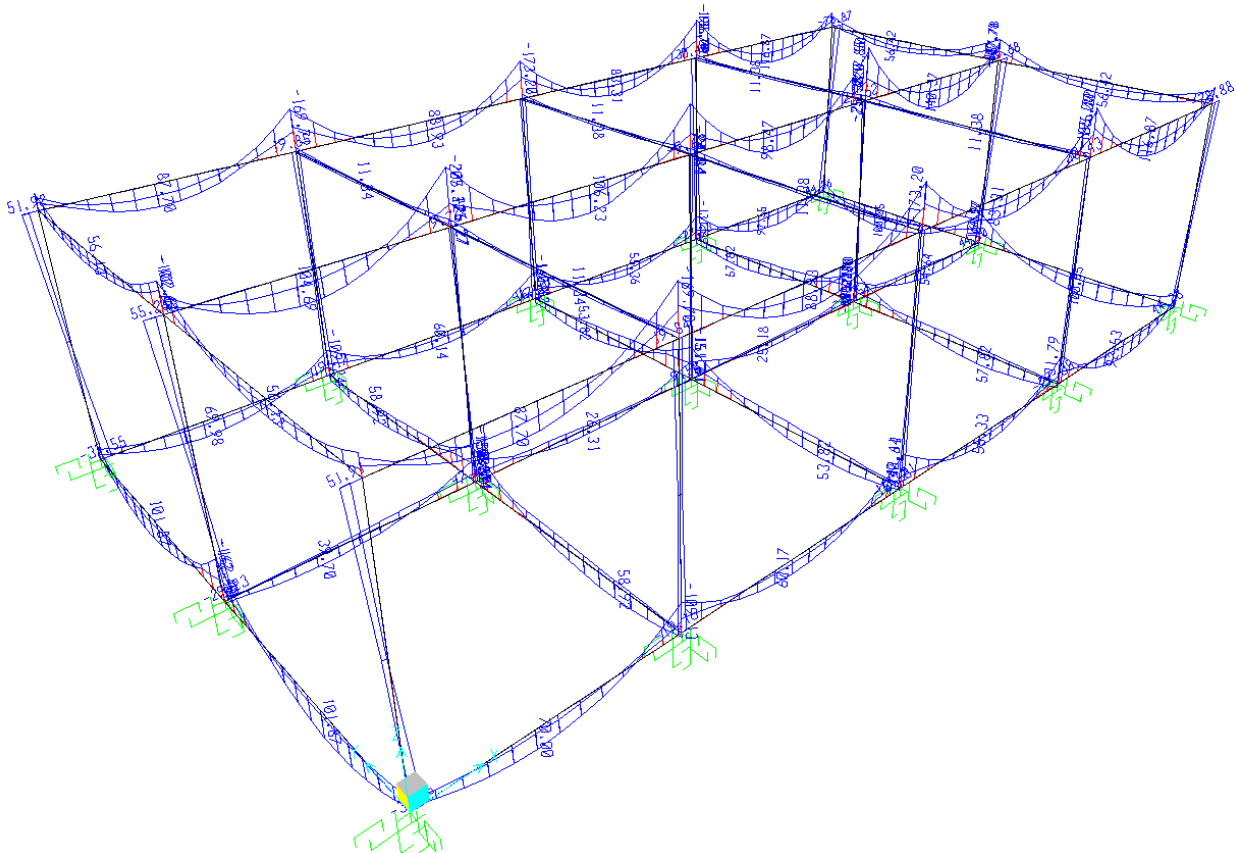
Momento M3 - Involuppo SLER
