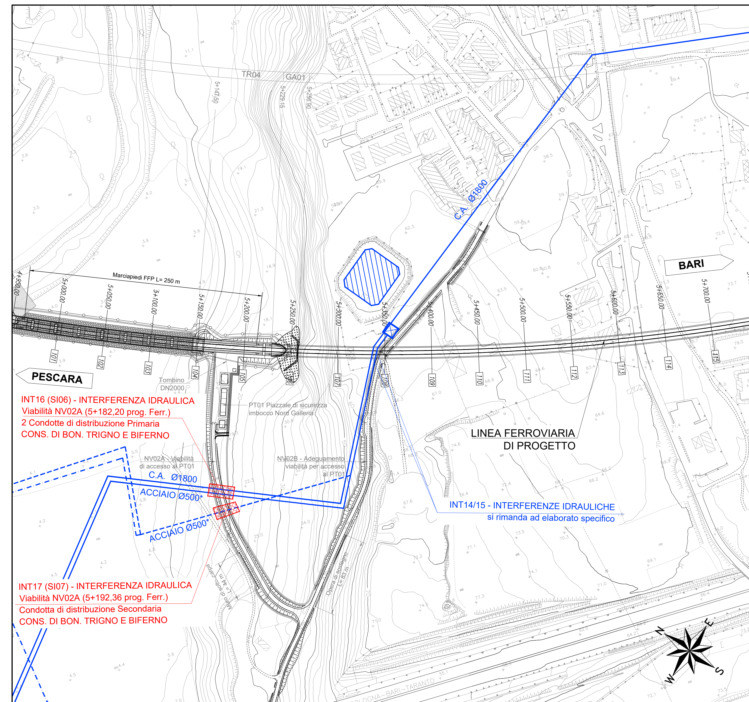
SI06 SI07 RILIEVO scala 1:2000
