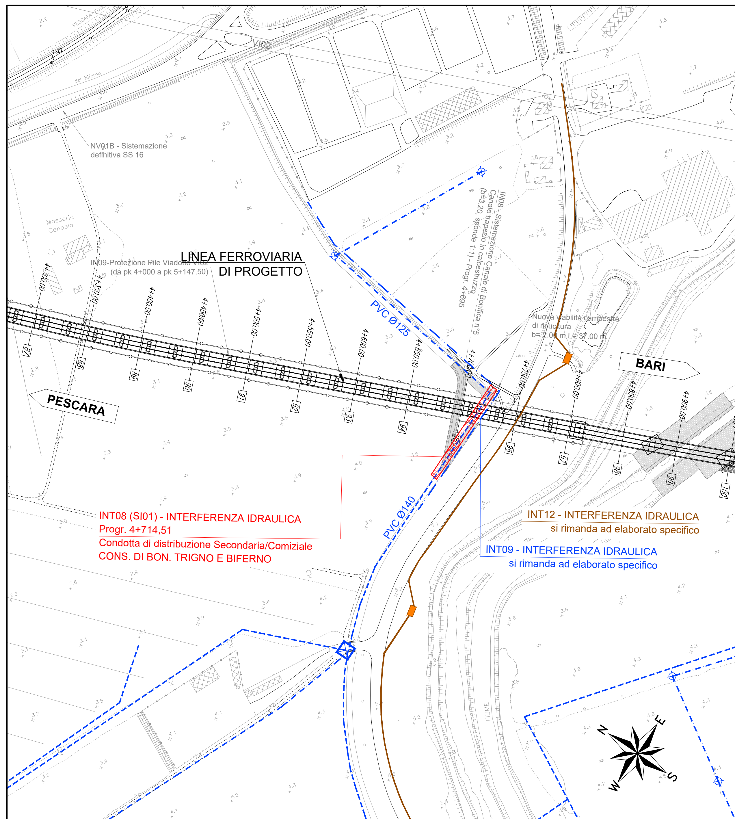
SI01 RILIEVO scala 1:2000
