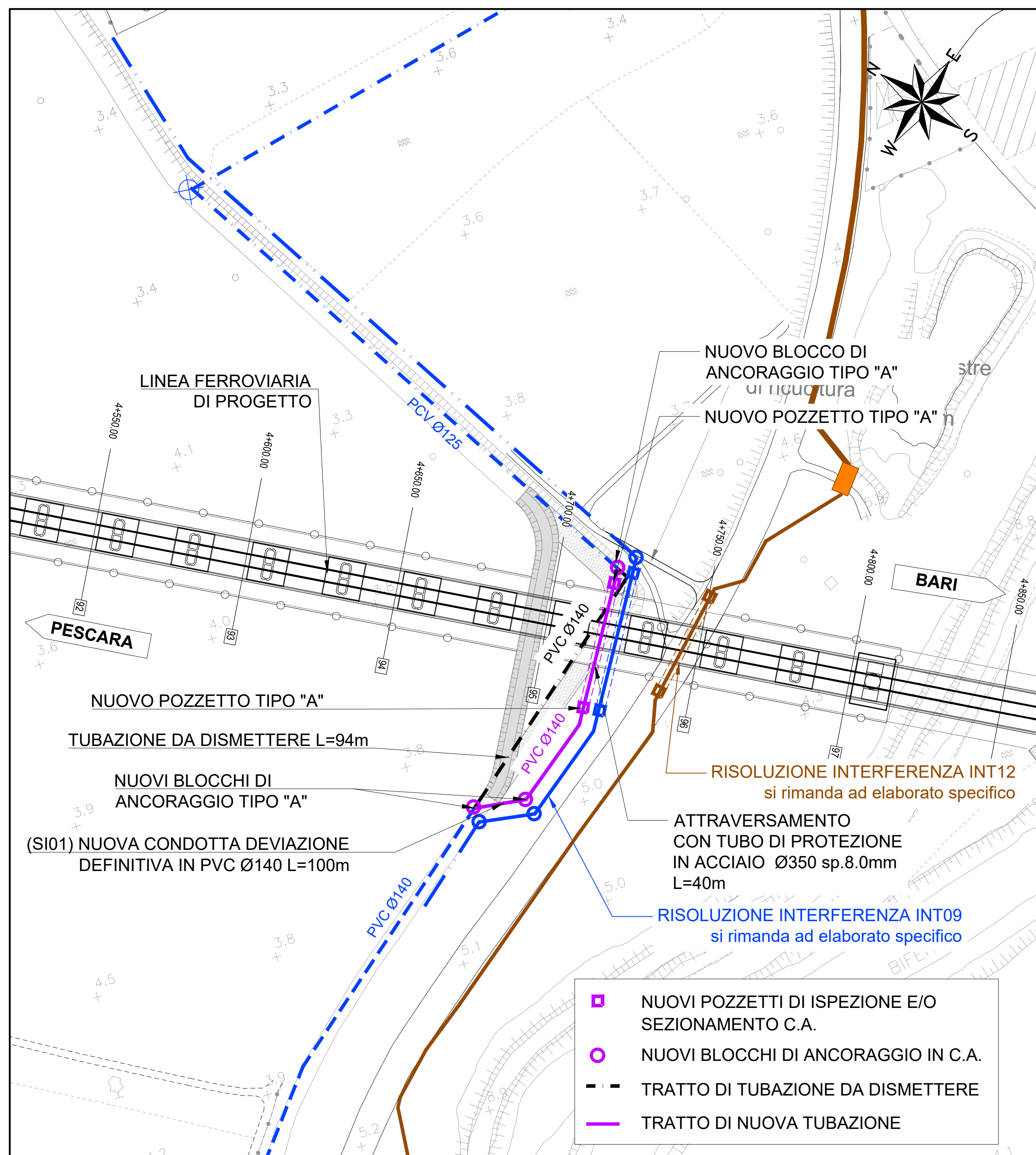
SI01 RISOLUZIONE scala 1:1000
