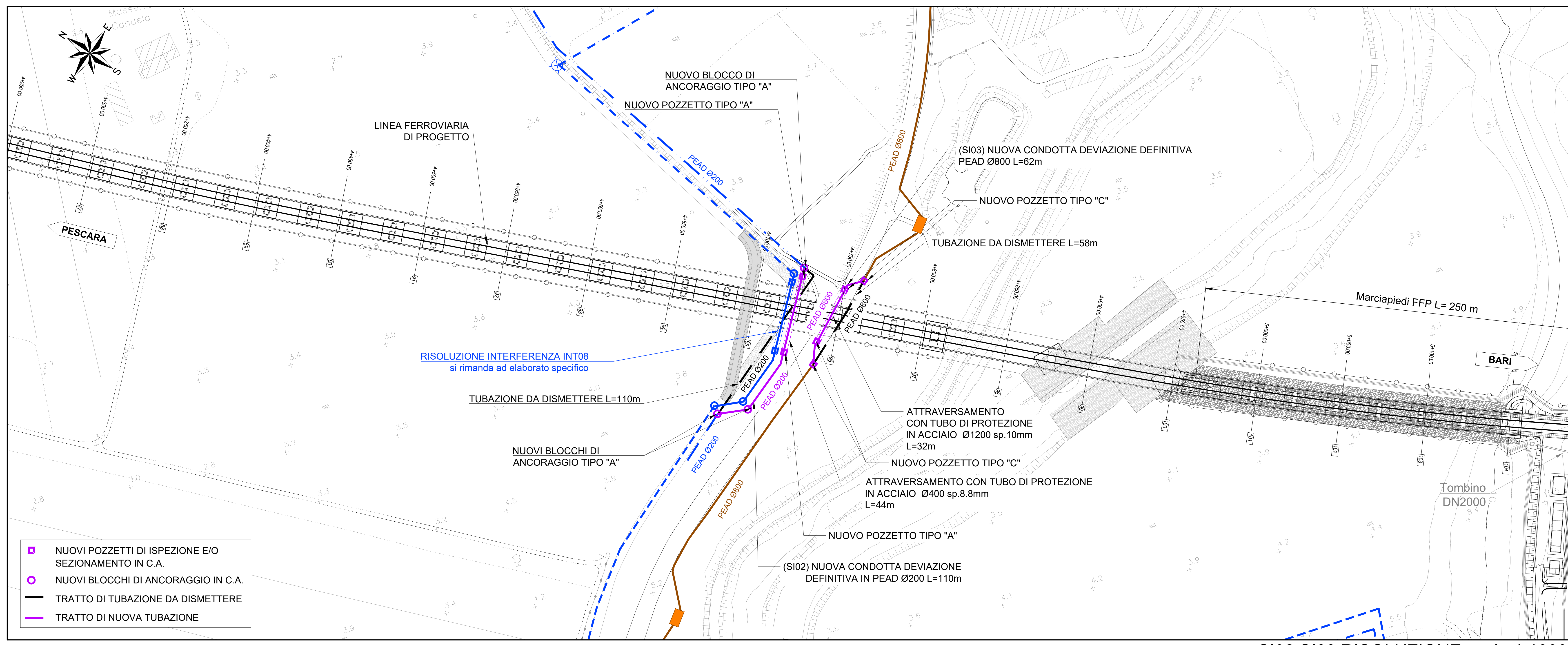
SI02 SI03 RISOLUZIONE scala 1:1000
