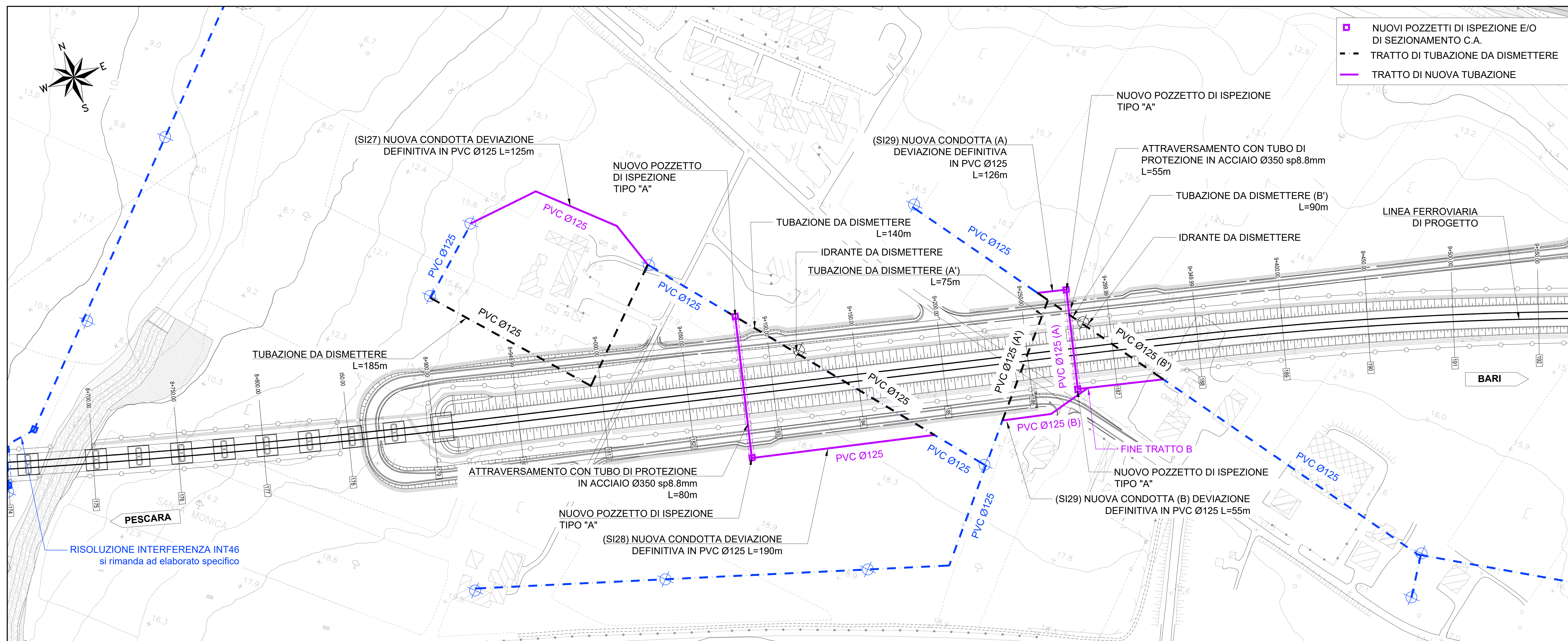
SI27 SI28 SI29 RISOLUZIONE - SCALA 1:2000
