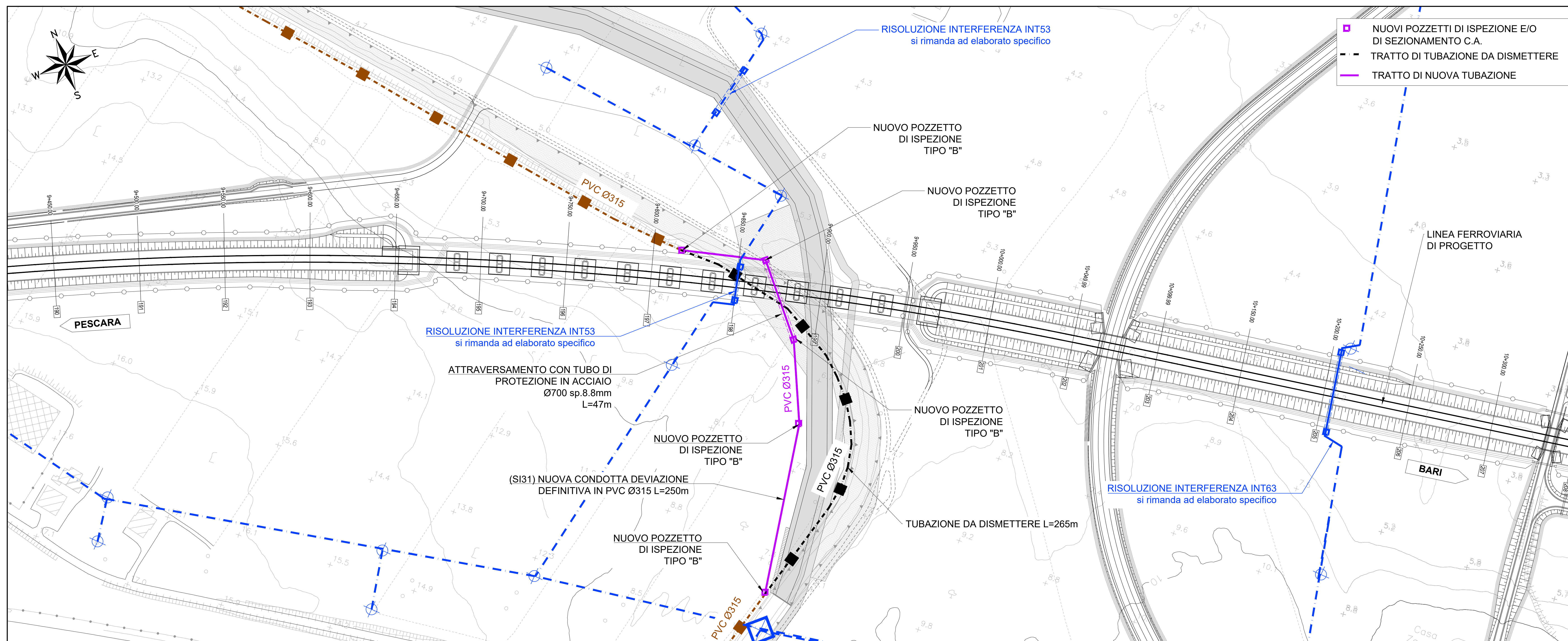
SI31 RISOLUZIONE - SCALA 1:1000
