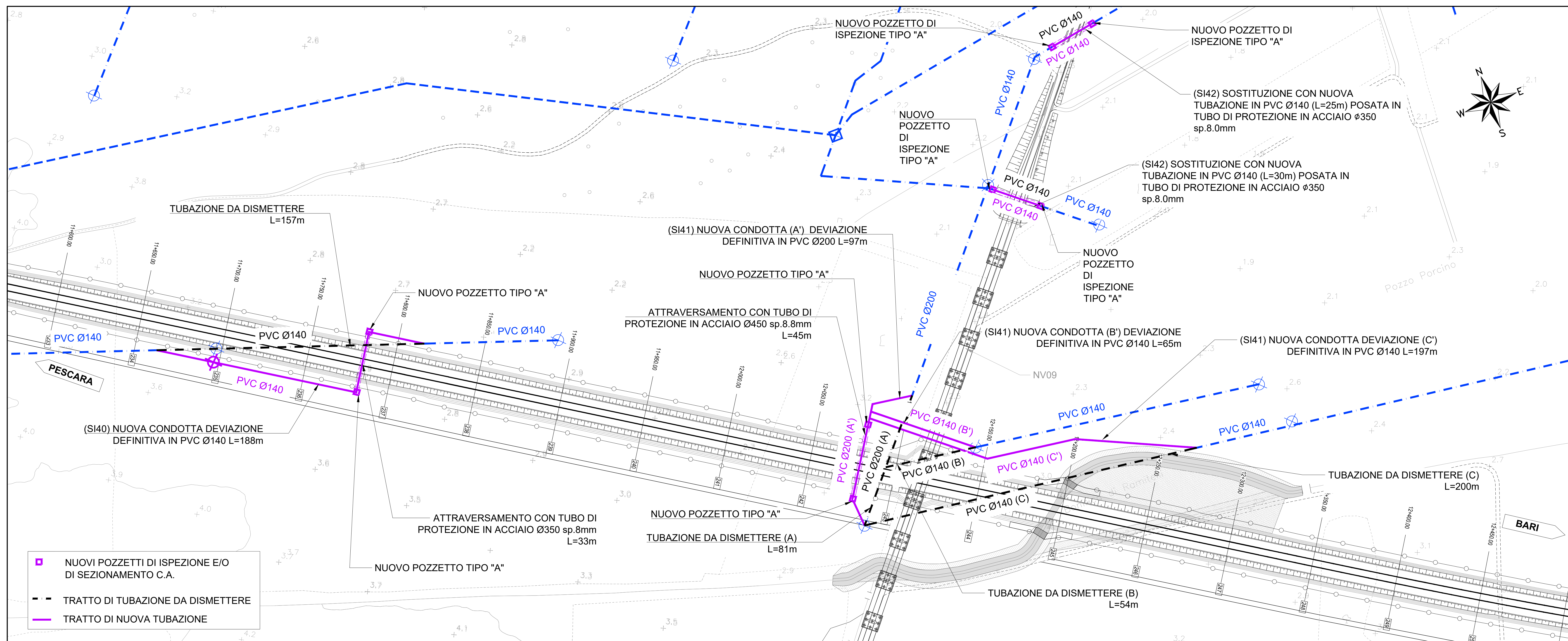
SI40 SI41 SI42 RISOLUZIONE - SCALA 1:1000
