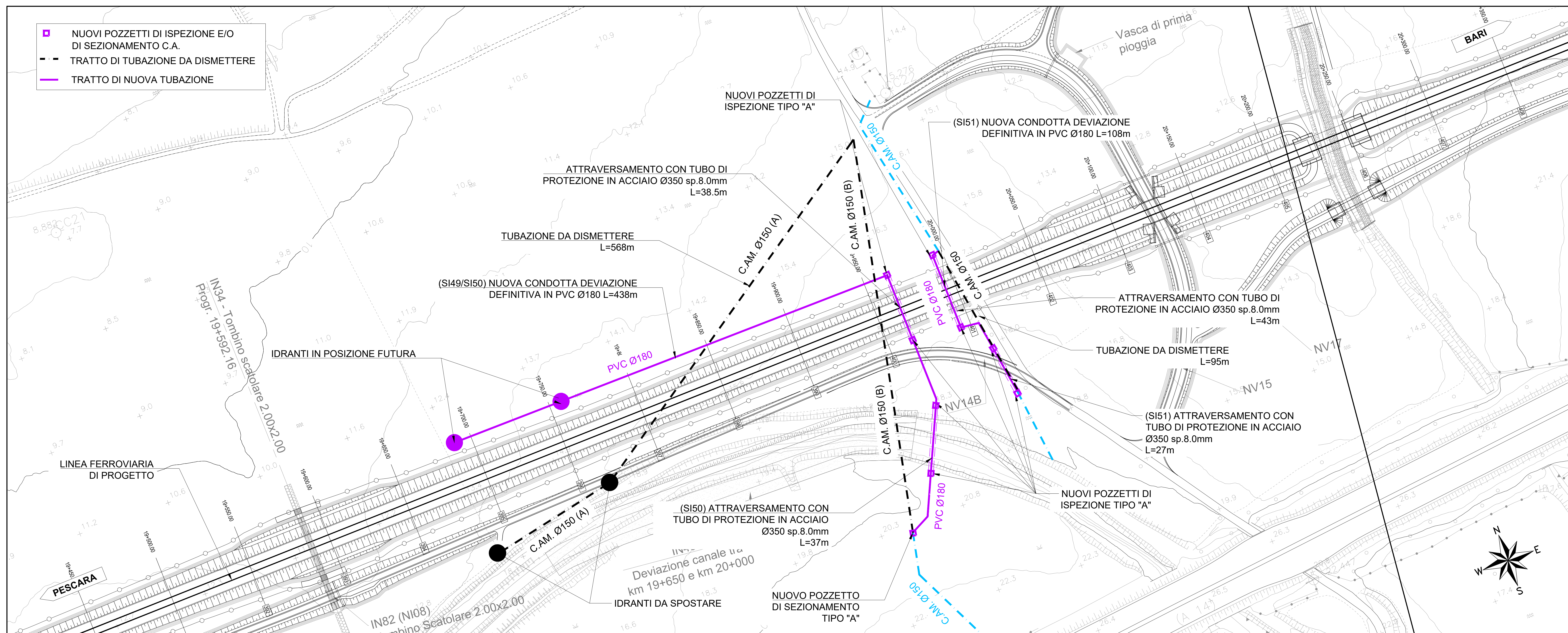
SI49/SI50/SI51 RISOLUZIONE - SCALA 1:1000
