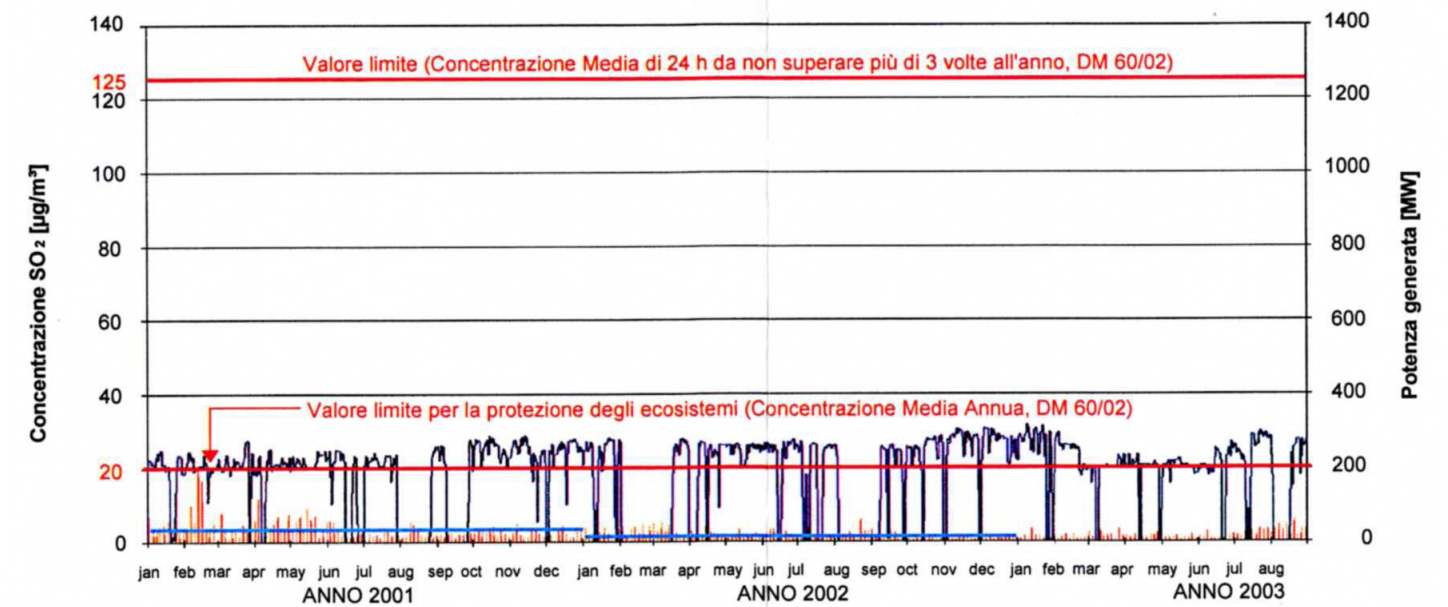
CONCENTRAZIONI MEDIE GIORNALIERE DI SO 2 Postazione No. 3 in località La Rosa
