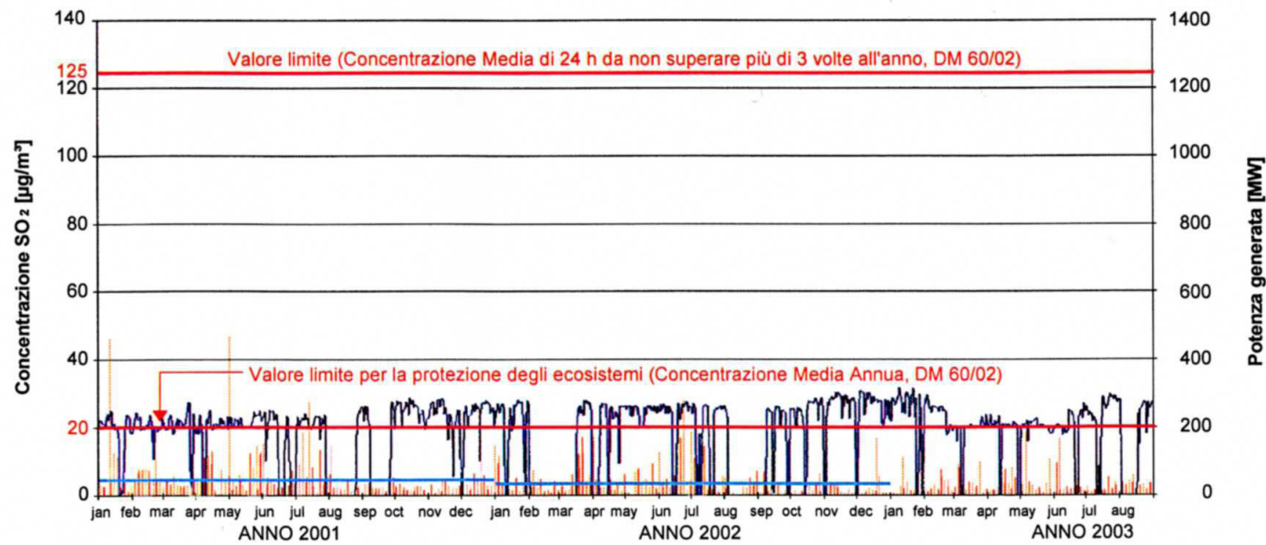
CONCENTRAZIONI MEDIE GIORNALIERE DI SO 2 Postazione No. 2 in località Tutarano
