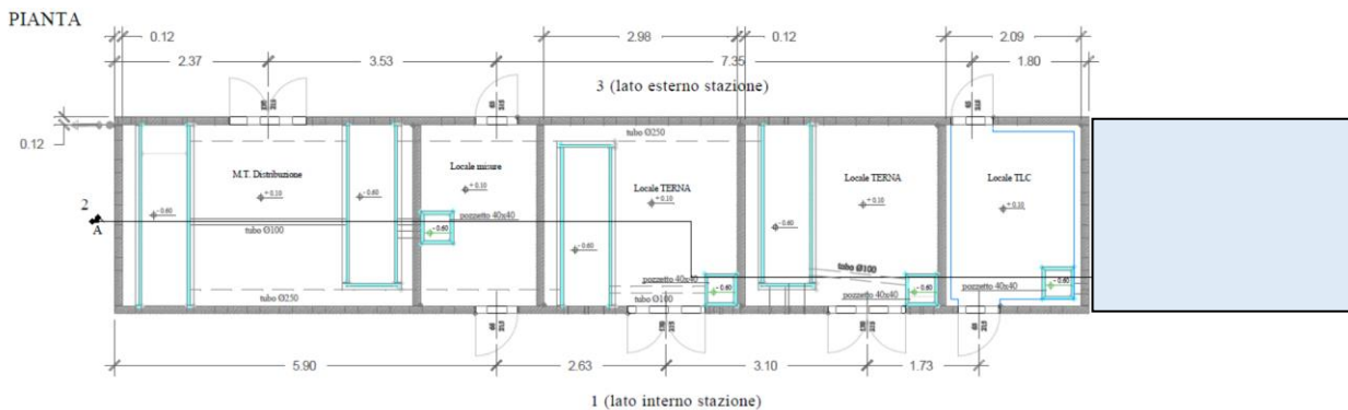
Fig. 2 – Layout in SSE Produttore autorizzato con individuato il nuovo locale tecnico da realizzare (celeste).
