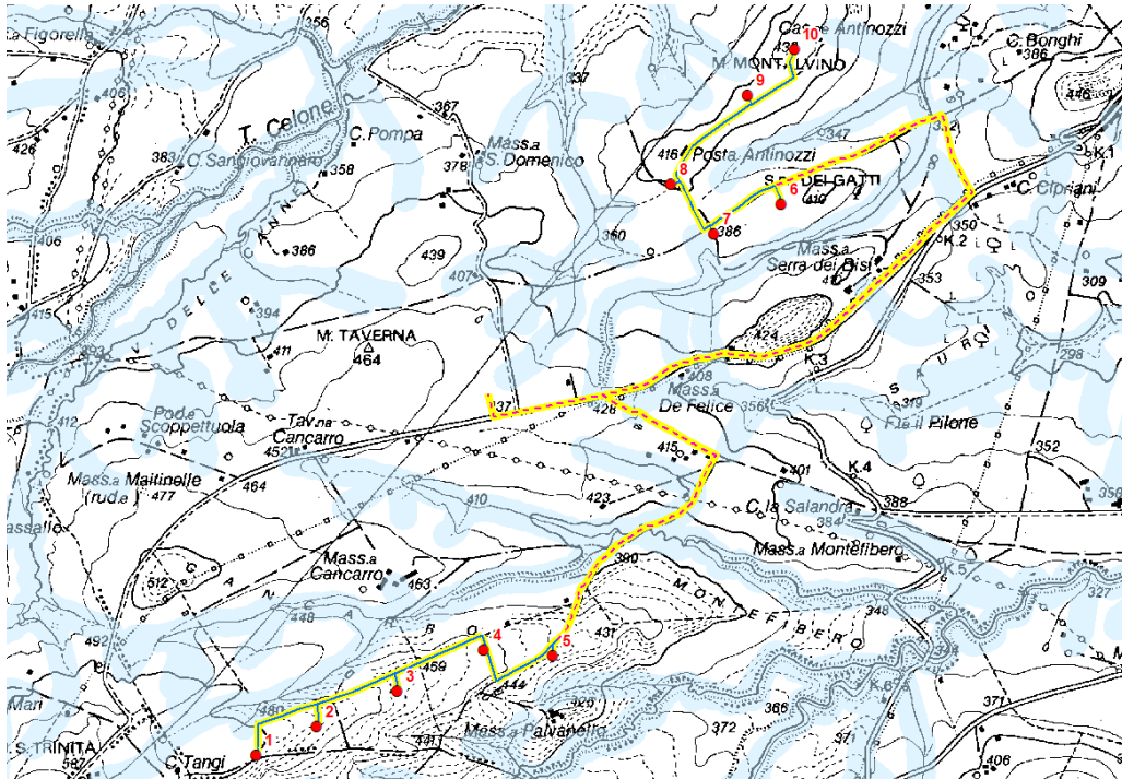
Fig. 2 - Reticolo idrografico Carta Idrogeomorfologica AdB Interferenza con strade e cavidotto
