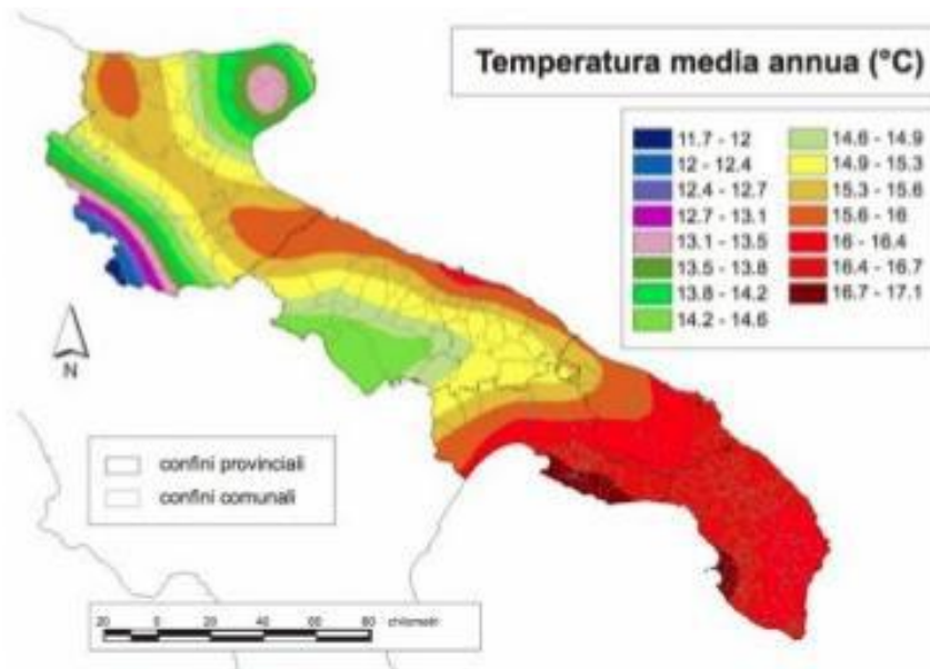
Fig. 5 - Distribuzione spaziale delle temperature medie annue in Puglia
