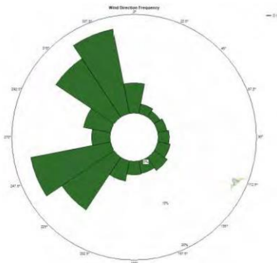
Fig. 6 - WIND Rose del sito
