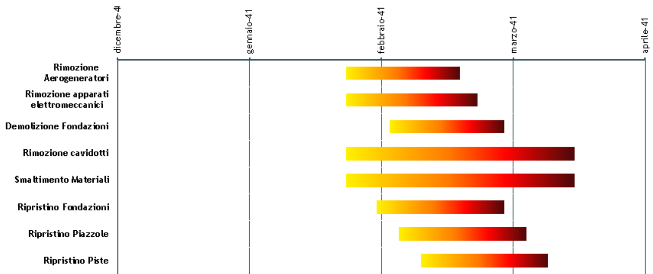
Figura 2 Cronoprogramma dismissione
