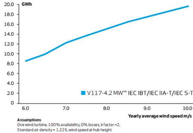
Figura 1. Curva di Potenza di una Vestas V117
