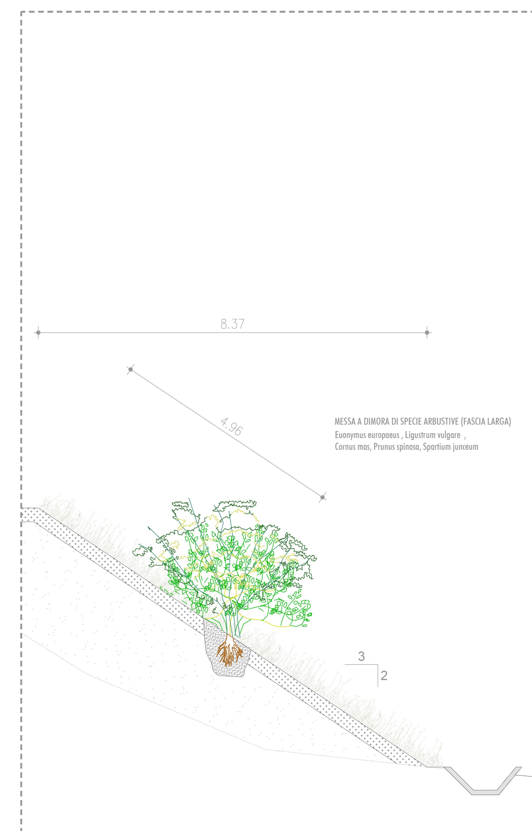
PARTICOLARE C: SISTEMAZIONE A VERDE DELLE SCARPATE SCALA 1:50
