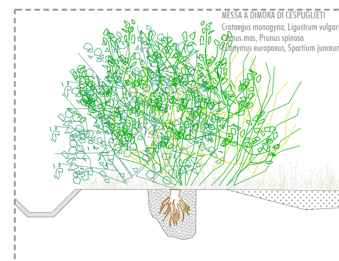
PARTICOLARE B: INTERVENTI DI SISTEMAZIONE NATURALISTICA E PAESAGGISTICA DELLE AREE INTERCLUSE TRA LA VIABILITÀ PRINCIPALE E QUELLA SECONDARIA 1:50
