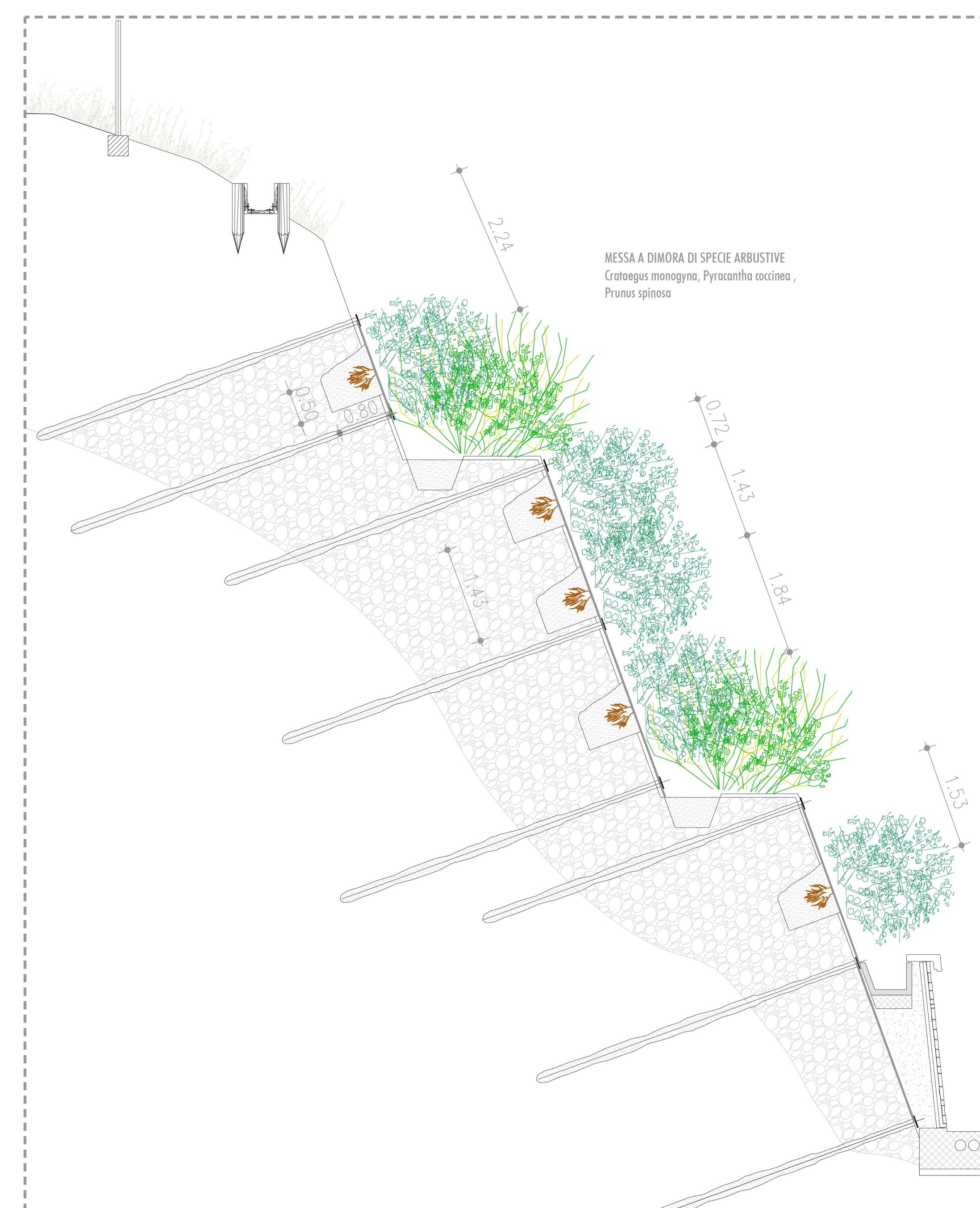
PARTICOLARE A: INTERVENTI DI INGEGNERIA NATURALISTICA SCALA 1:50
