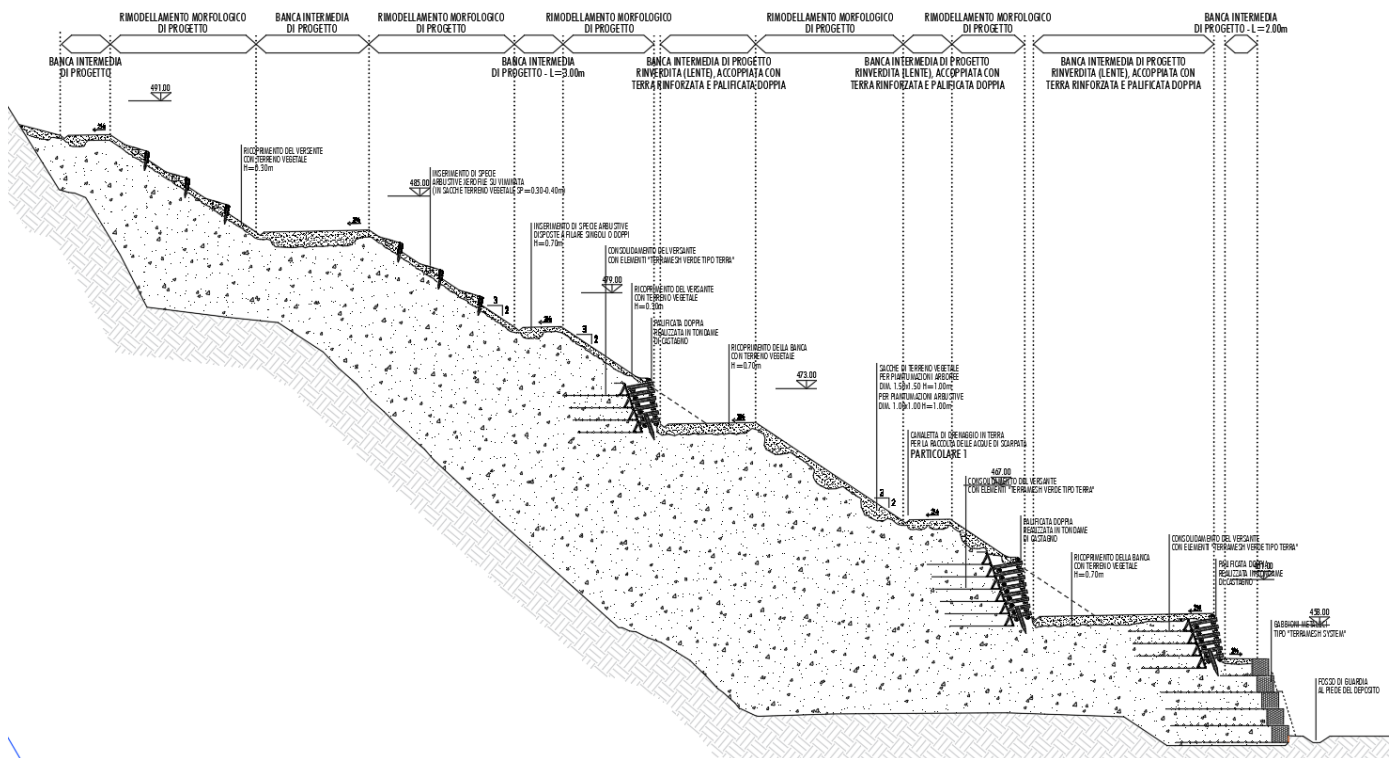
FIGURA 4-5 – SEZIONE TIPO
