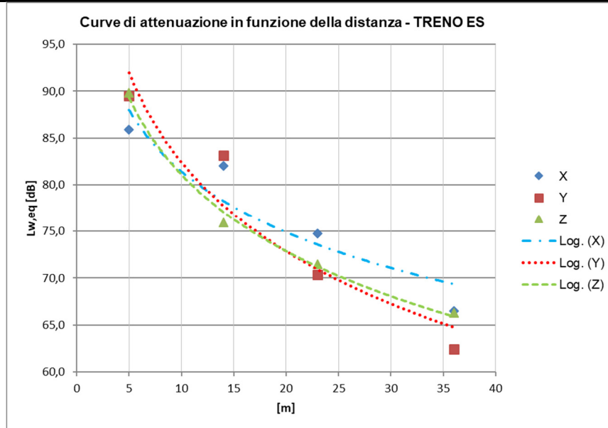
Figura 15 - Curva di attenuazione del L_{w,eq} in funzione della distanza dal binario, ricavata dai rilievi sperimentali sull'attuale linea in esercizio lungo gli assi x,y e z, in corrispondenza delle VIB 01,02, 03 e 04 – TIPOLOGIA TRENO ES
