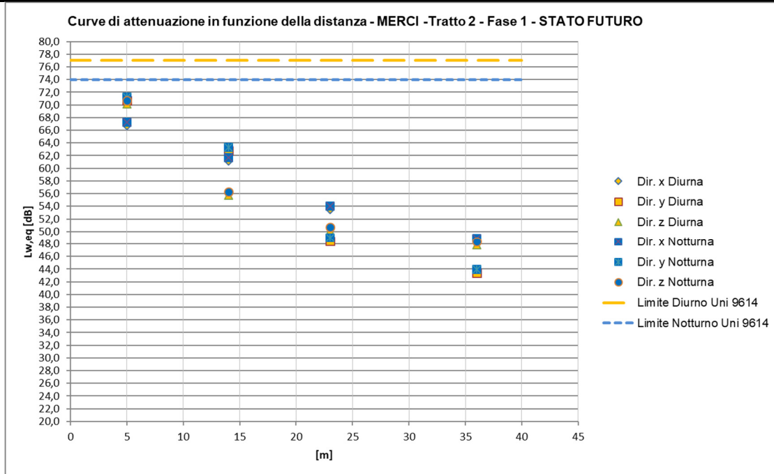
Figura 31 – Curve di attenuazione in funzione della distanza relativa al traffico ferroviario di progetto – Treni Mercy
