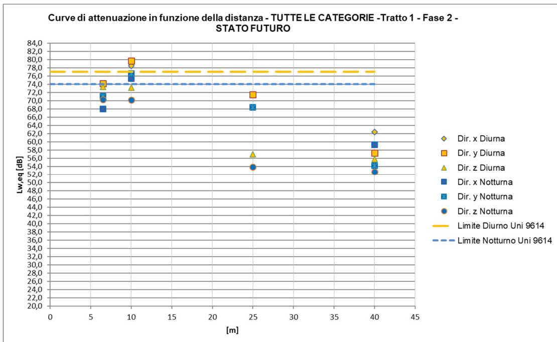
Figura 28 – Curve di attenuazione in funzione della distanza relativa al traffico ferroviario di progetto – Treni Totali Regionali + Metropolitani + Mercati + IC/EC + ES
