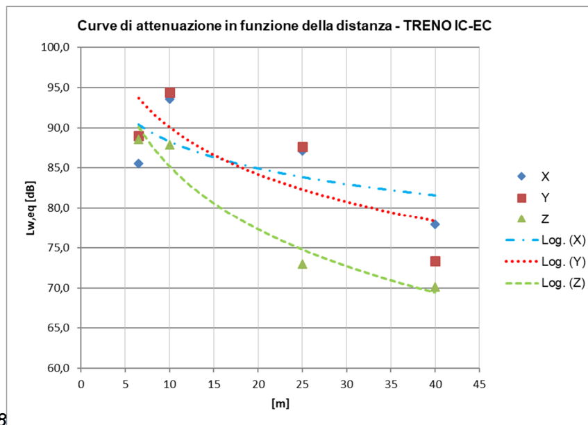
Figura 8 - Curva di attenuazione del L_{w,eq} in funzione della distanza dal binario, ricavata dai rilievi sperimentali sull'attuale linea in esercizio lungo gli assi x,y e z, in corrispondenza delle VIB 01,02, 03 e 04 – TIPOLOGIA TRENO IC/EC
