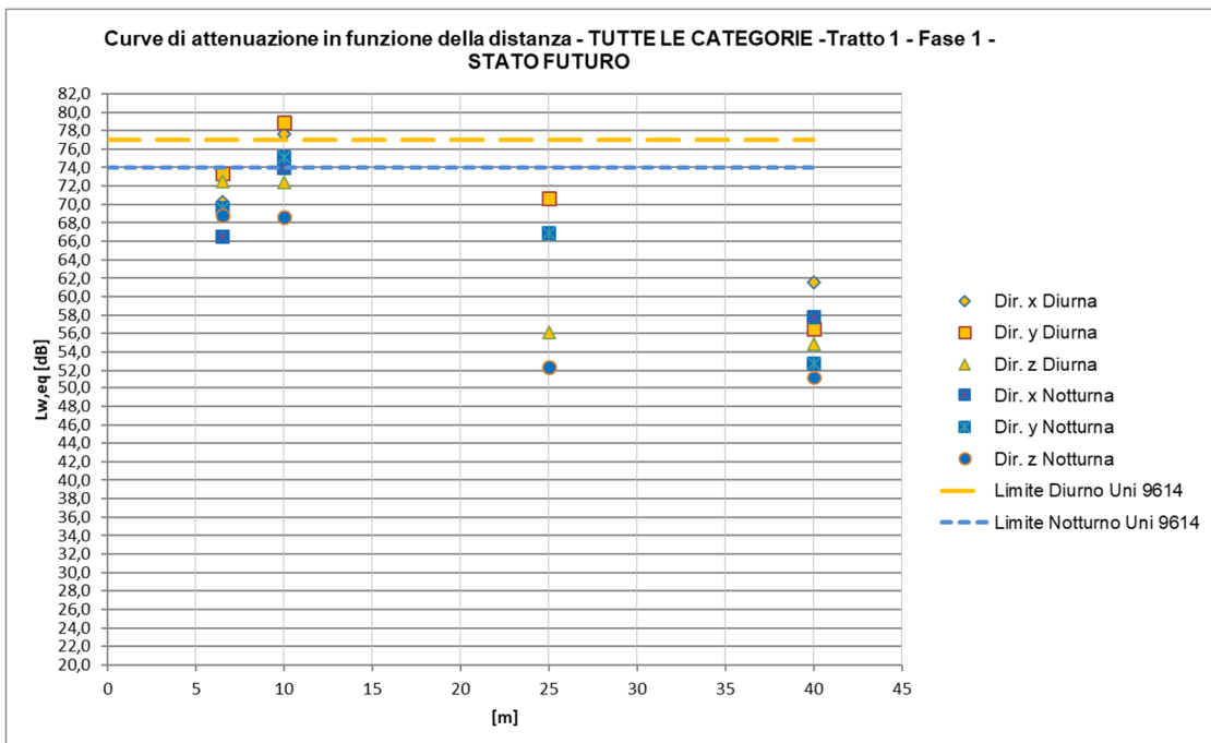
Figura 22 – Curve di attenuazione in funzione della distanza relativa al traffico ferroviario di progetto – Treni Totali Regionali + Metropolitani + Mercati + IC/EC + ES
