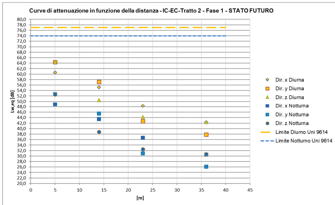
Figura 32 – Curve di attenuazione in funzione della distanza relativa al traffico ferroviario di progetto – Treni IC/EC
