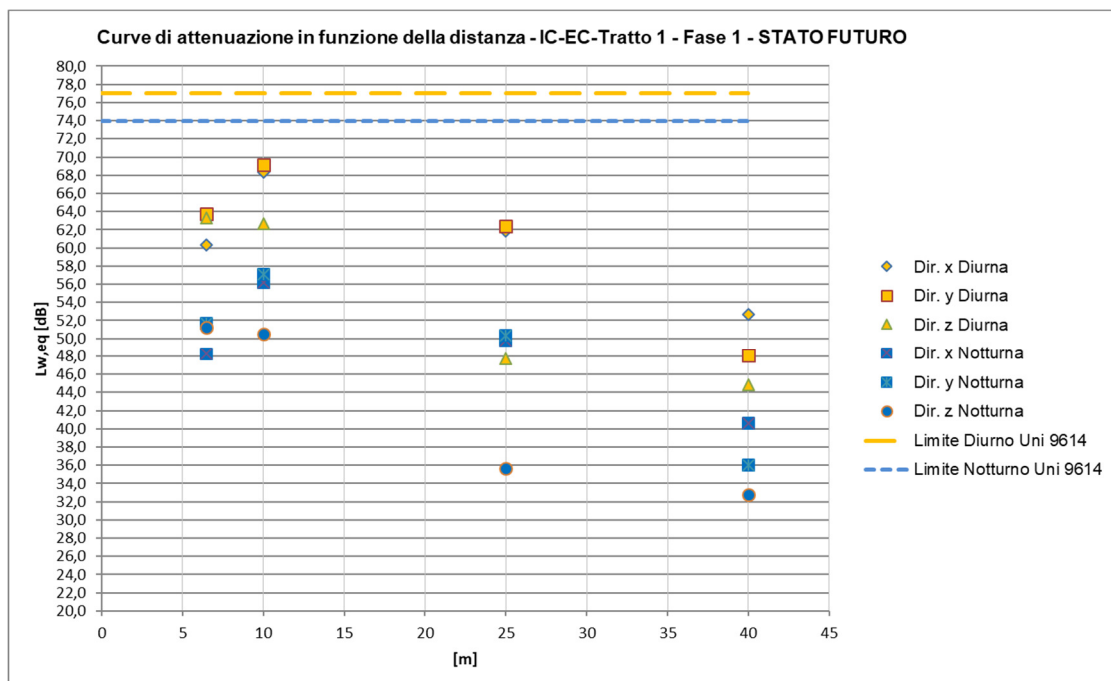
Figura 20 – Curve di attenuazione in funzione della distanza relativa al traffico ferroviario di progetto – Treni IC/EC
