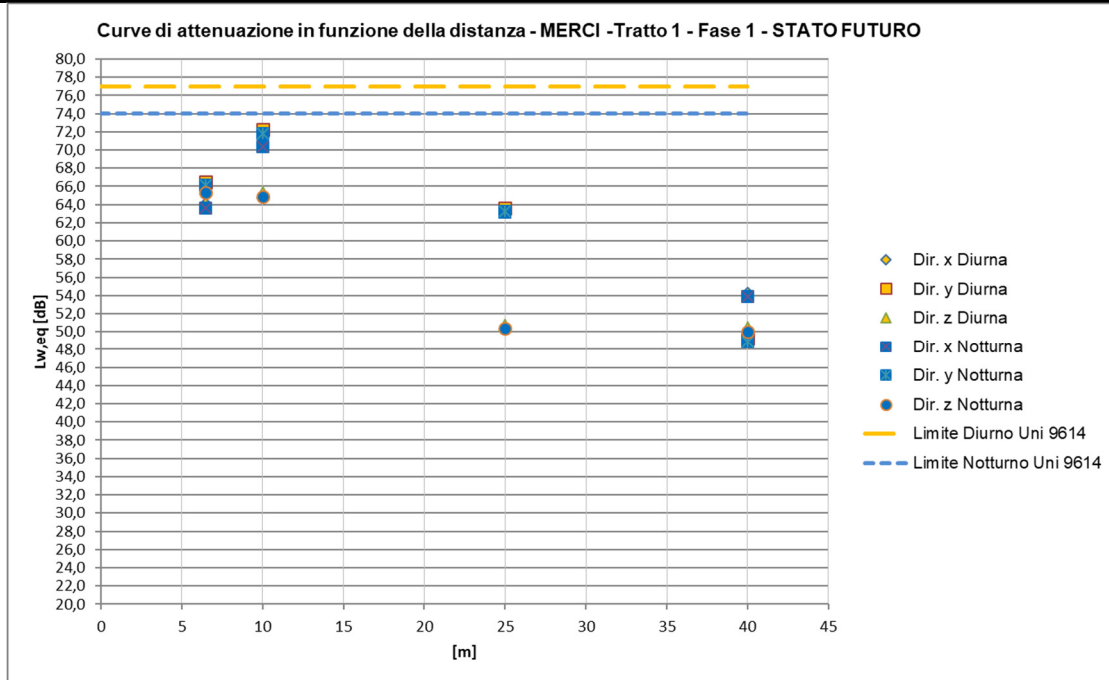
Figura 19 – Curve di attenuazione in funzione della distanza relativa al traffico ferroviario di progetto – Treni Mercy
