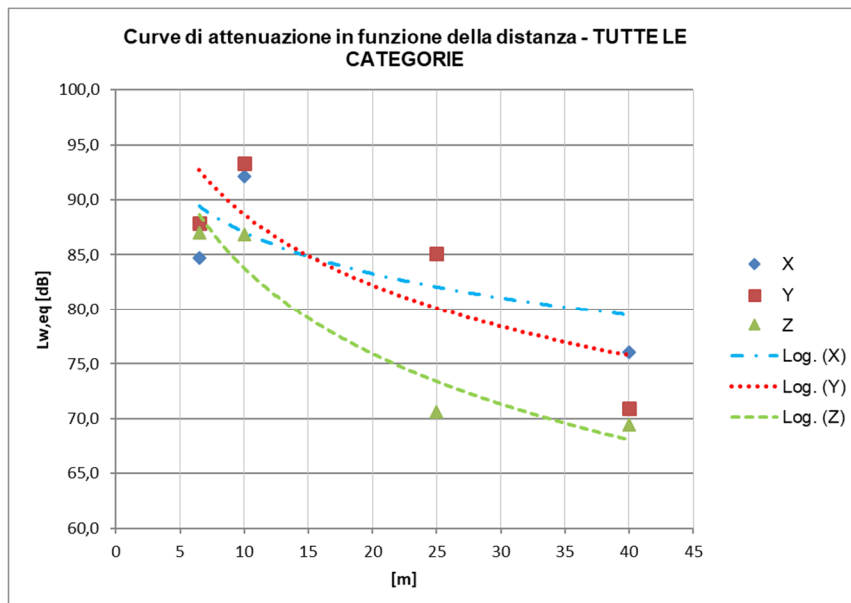
Figura 10 - Curva di attenuazione del L_{w,eq} in funzione della distanza dal binario, ricavata dai rilievi sperimentali sull'attuale linea in esercizio lungo gli assi x,y e z, in corrispondenza delle VIB 01,02, 03 e 04 – TOTALE REGIONALI + METROPOLITANO+MERC1+IC/EC+ES
