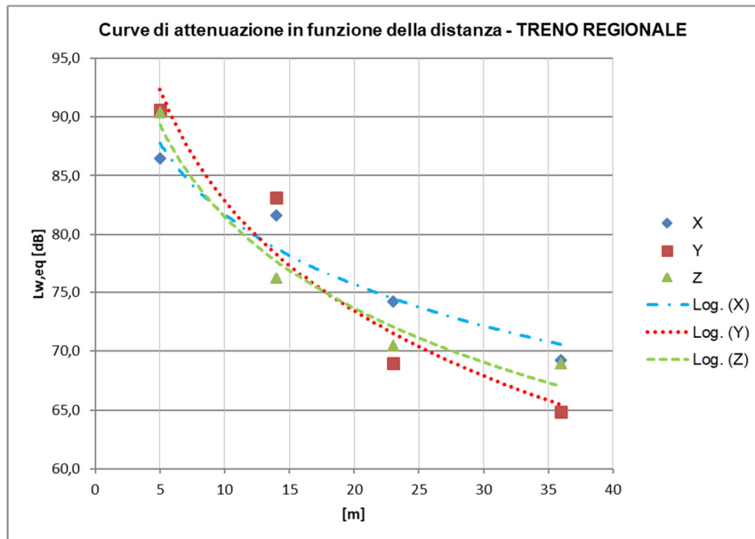
Figura 11 - Curva di attenuazione del L_{w,eq} in funzione della distanza dal binario, ricavata dai rilievi sperimentali sull'attuale linea in esercizio lungo gli assi x,y e z, in corrispondenza delle VIB 01,02, 03 e 04 – TIPOLOGIA TRENO REGIONALE
