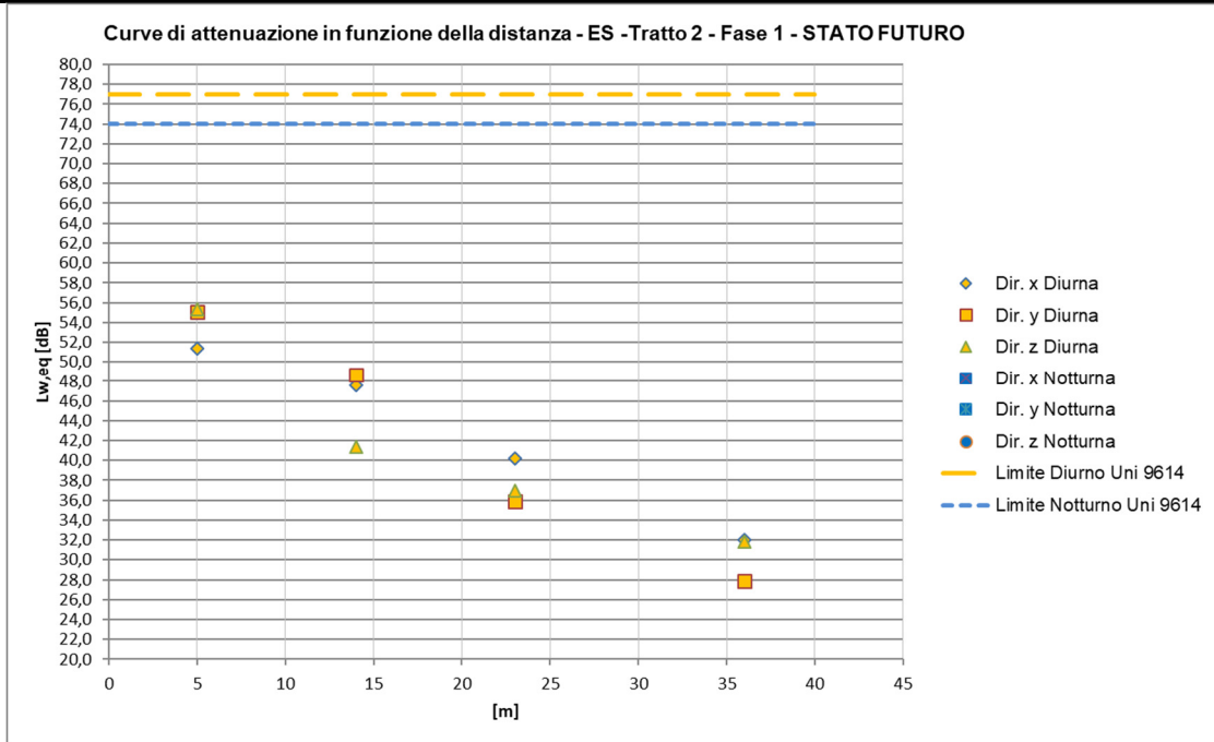
Figura 33 – Curve di attenuazione in funzione della distanza relativa al traffico ferroviario di progetto – Treni ES
