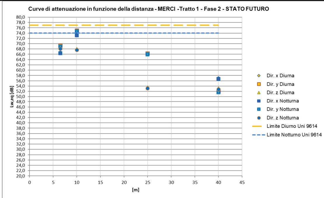
Figura 25 – Curve di attenuazione in funzione della distanza relativa al traffico ferroviario di progetto – Treni Mercy
