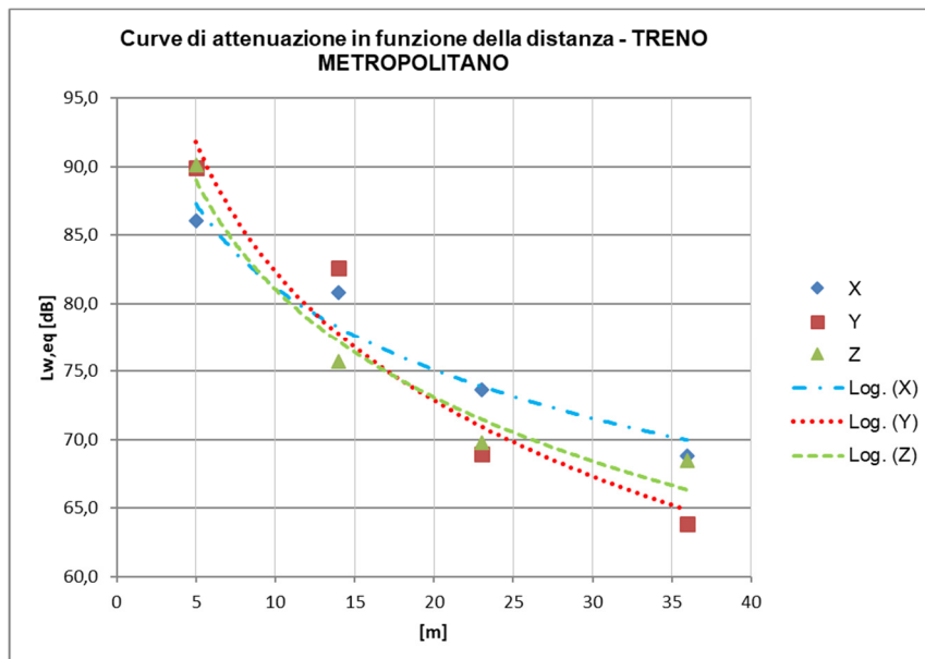
Figura 12 - Curva di attenuazione del L_{w,eq} in funzione della distanza dal binario, ricavata dai rilievi sperimentali sull'attuale linea in esercizio lungo gli assi x,y e z, in corrispondenza delle VIB 01,02, 03 e 04 – TIPOLOGIA TRENO METROPOLITANO
