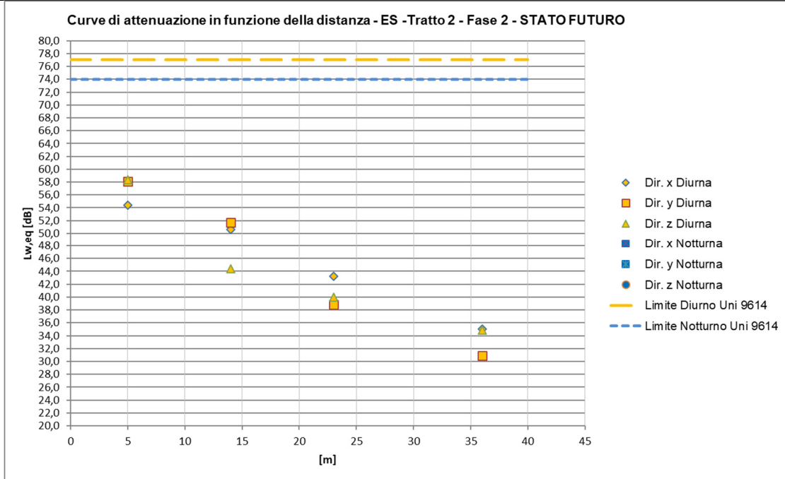
Figura 39 – Curve di attenuazione in funzione della distanza relativa al traffico ferroviario di progetto – Treni ES
