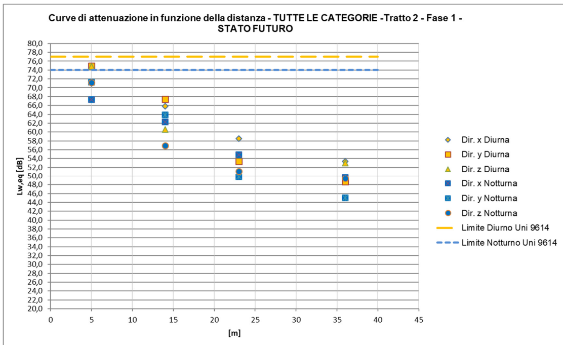
Figura 34 – Curve di attenuazione in funzione della distanza relativa al traffico ferroviario di progetto – Treni Totali Regionali + Metropolitani + Mercati + IC/EC + ES
