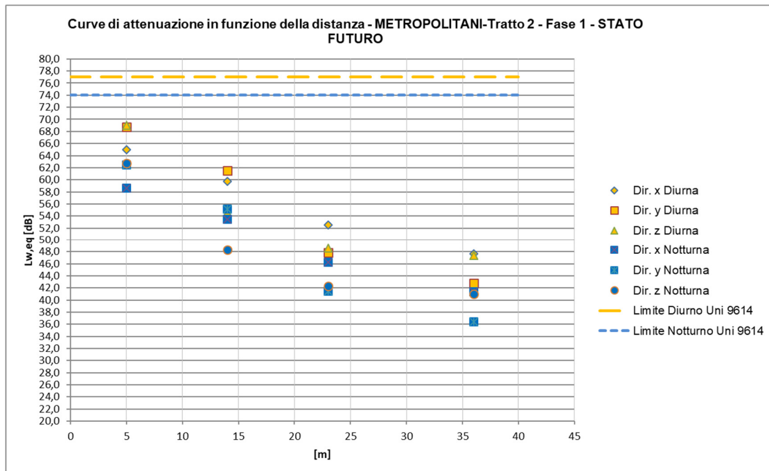
Figura 30 – Curve di attenuazione in funzione della distanza relativa al traffico ferroviario di progetto – Treni Metropolitan
