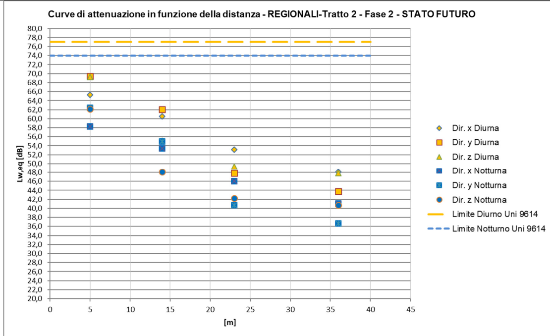
Figura 35 – Curve di attenuazione in funzione della distanza relativa al traffico ferroviario di progetto – Treni Regionale
