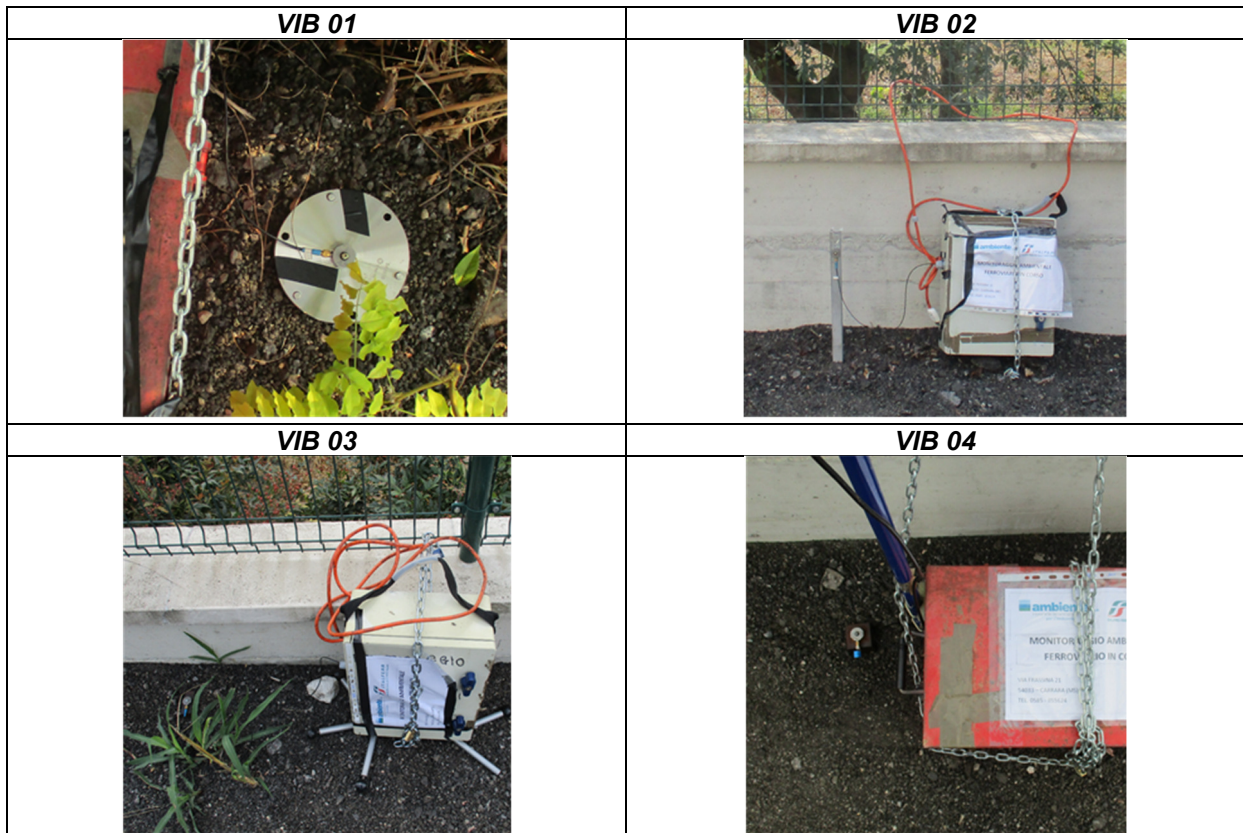
Figura 4 - Report fotografico postazioni di misura (Asse x: ortogonale alla linea; Asse Y: parallelo alla linea; Asse Z verticale)
