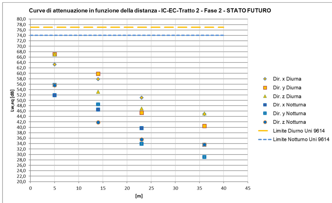
Figura 38 – Curve di attenuazione in funzione della distanza relativa al traffico ferroviario di progetto – Treni IC/EC
