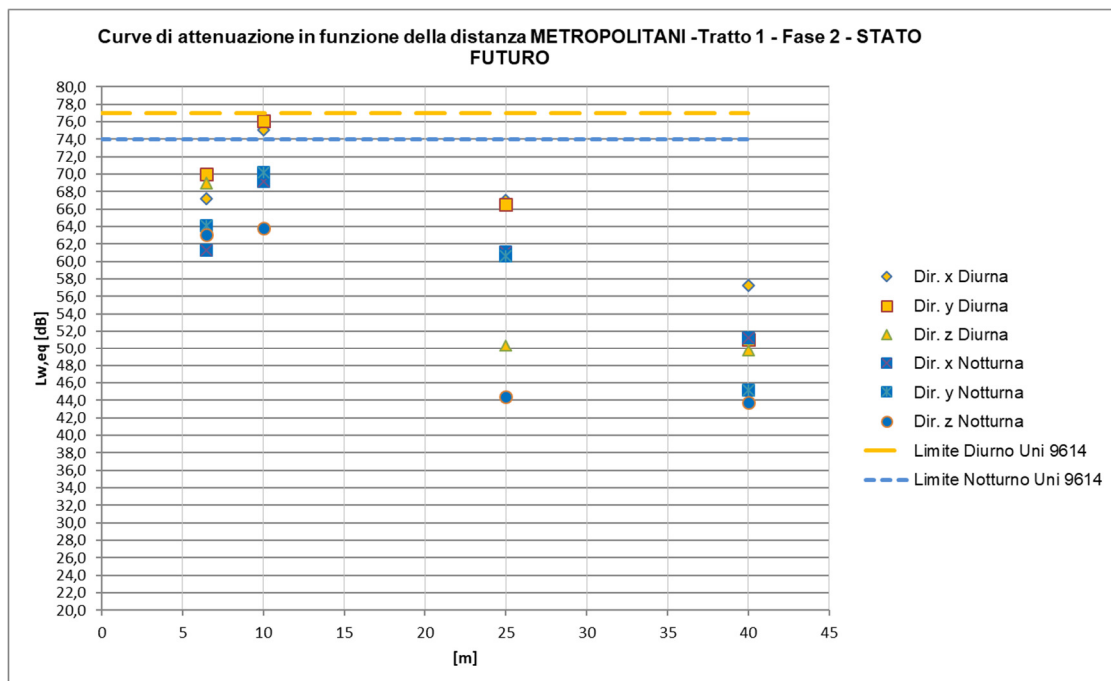
Figura 24 – Curve di attenuazione in funzione della distanza relativa al traffico ferroviario di progetto – Treni Metropolitan
