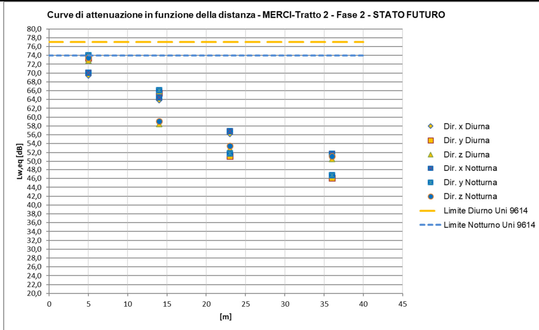
Figura 37 – Curve di attenuazione in funzione della distanza relativa al traffico ferroviario di progetto – Treni Mercier
