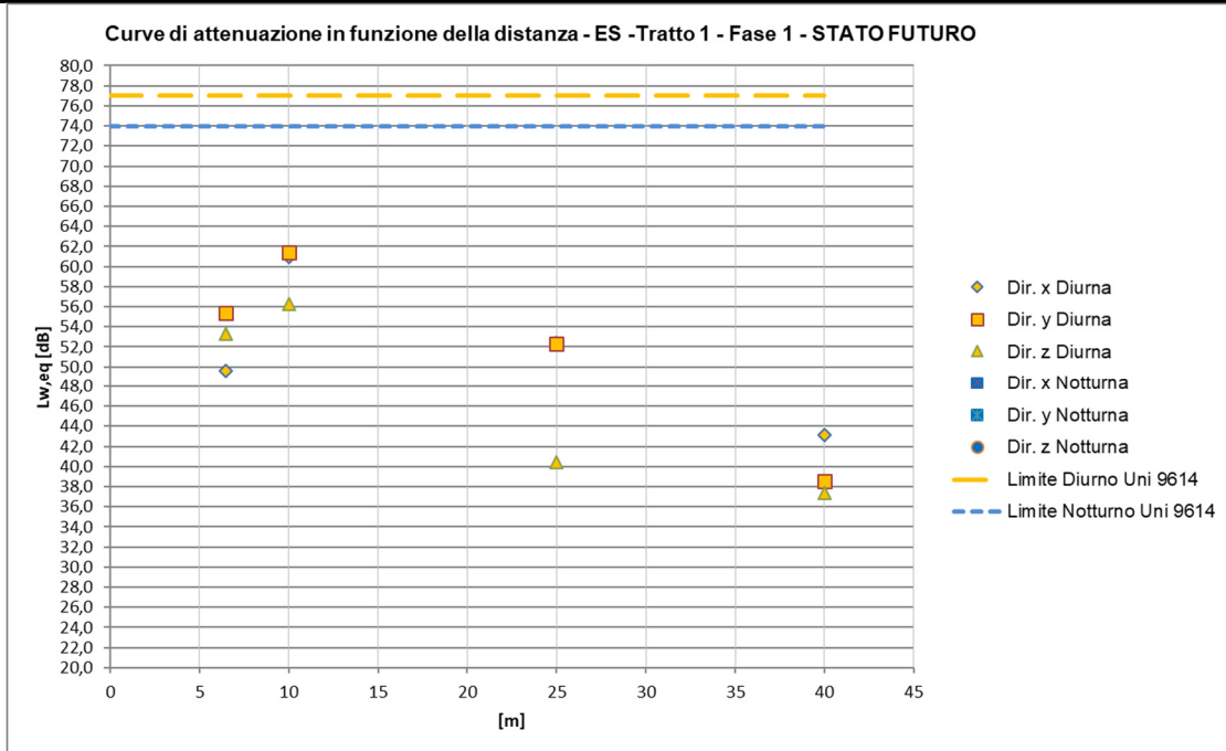
Figura 21 – Curve di attenuazione in funzione della distanza relativa al traffico ferroviario di progetto – Treni ES
