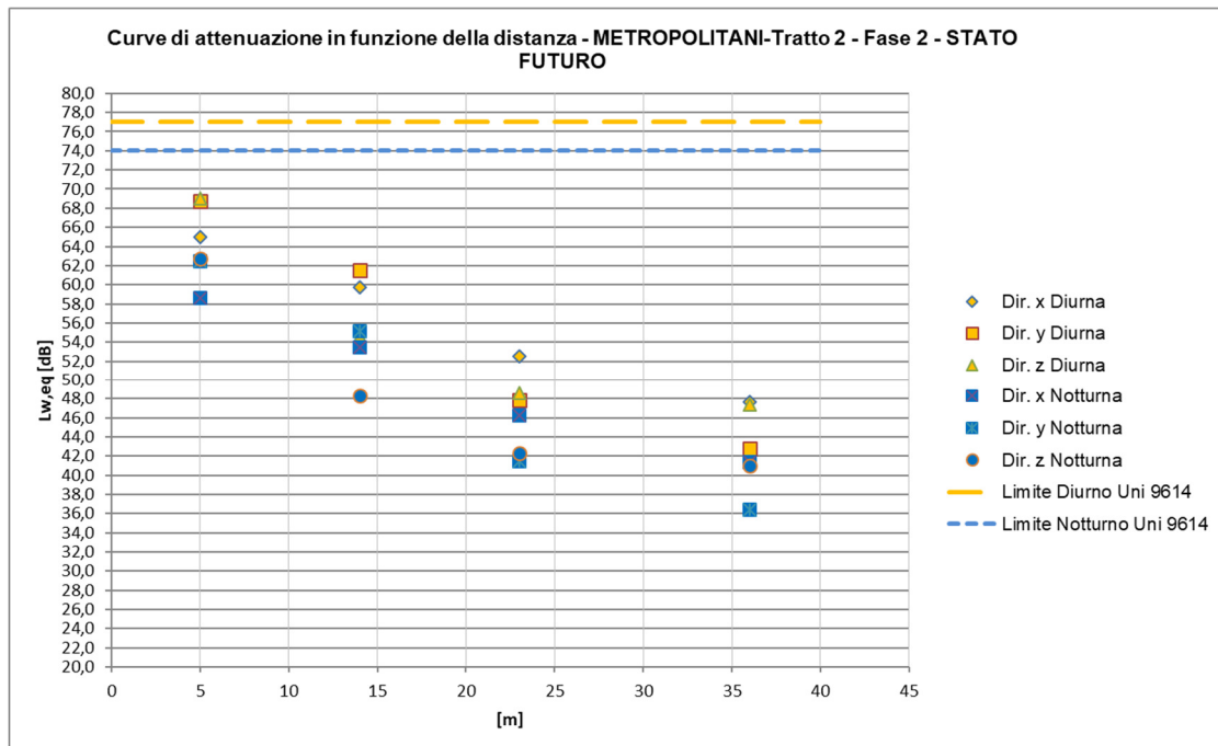
Figura 36 – Curve di attenuazione in funzione della distanza relativa al traffico ferroviario di progetto – Treni Metropolitan
