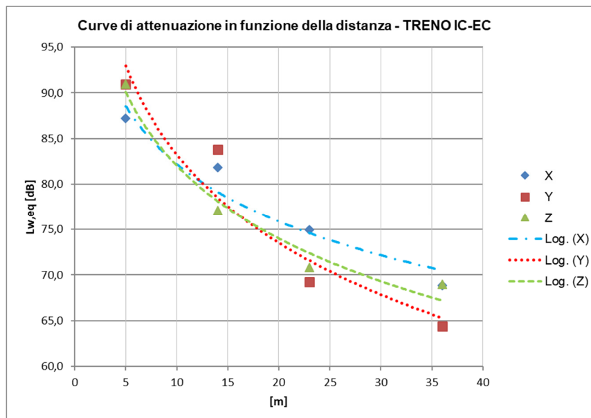
Figura 14 - Curva di attenuazione del L_{w,eq} in funzione della distanza dal binario, ricavata dai rilievi sperimentali sull'attuale linea in esercizio lungo gli assi x,y e z, in corrispondenza delle VIB 01,02, 03 e 04 – TIPOLOGIA TRENO IC/EC
