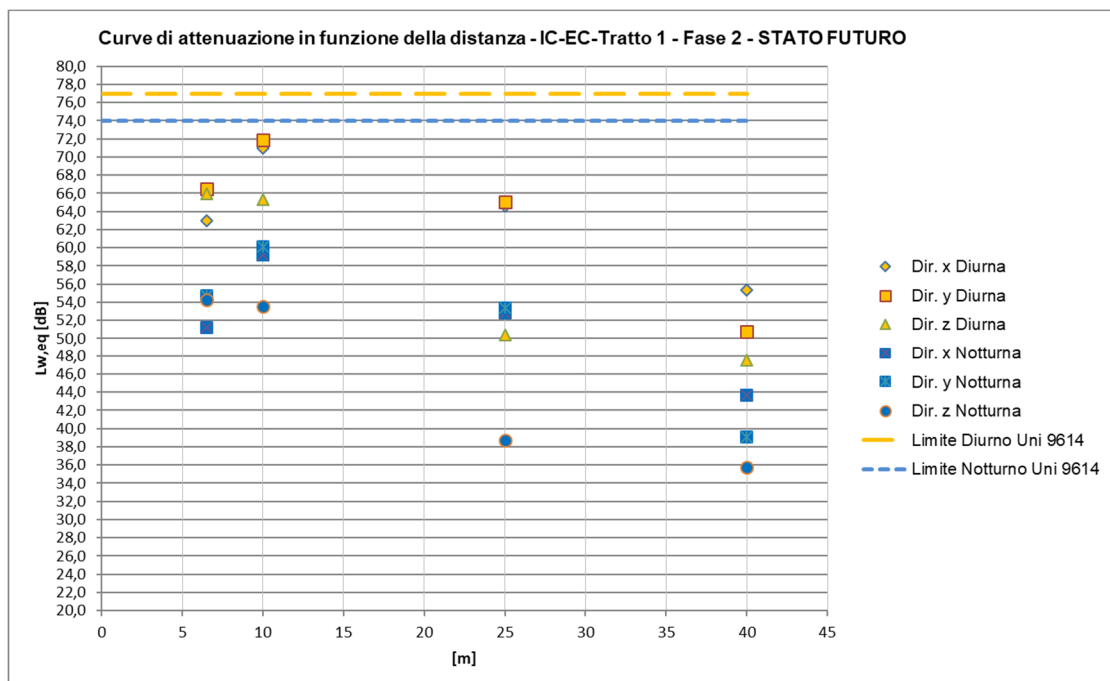
Figura 26 – Curve di attenuazione in funzione della distanza relativa al traffico ferroviario di progetto – Treni IC/EC
