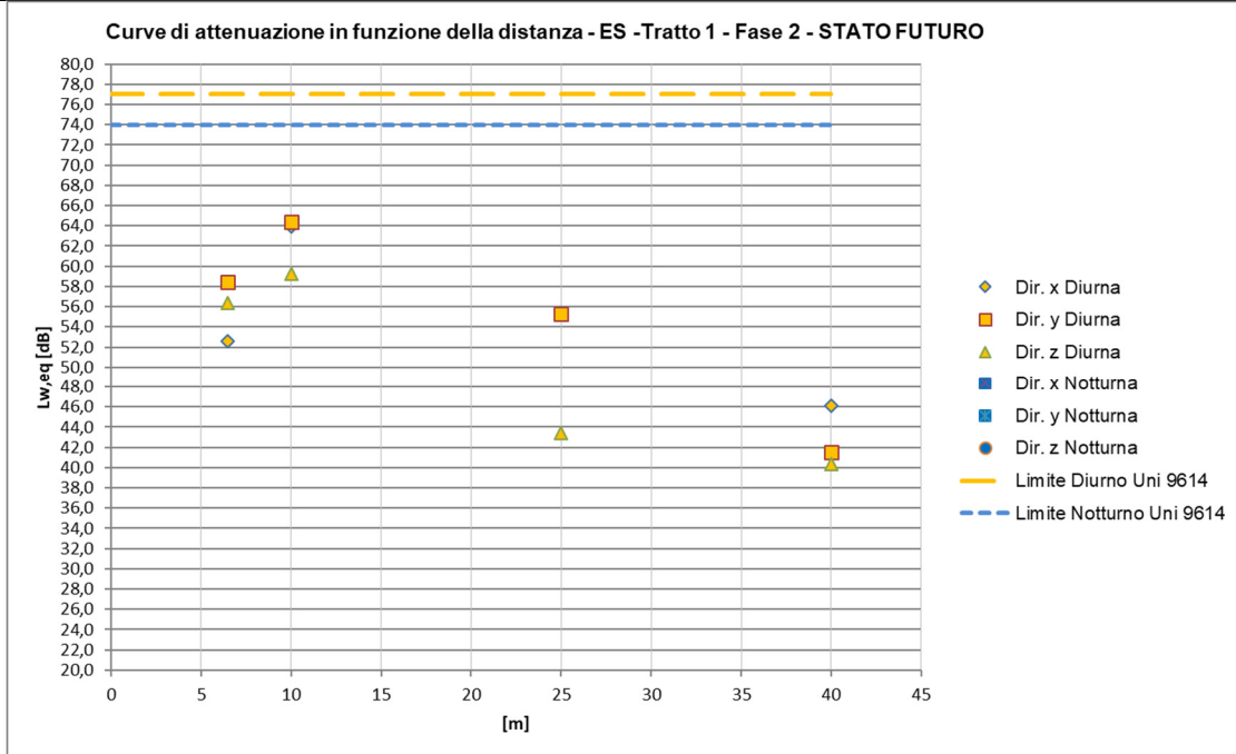
Figura 27 – Curve di attenuazione in funzione della distanza relativa al traffico ferroviario di progetto – Treni ES
