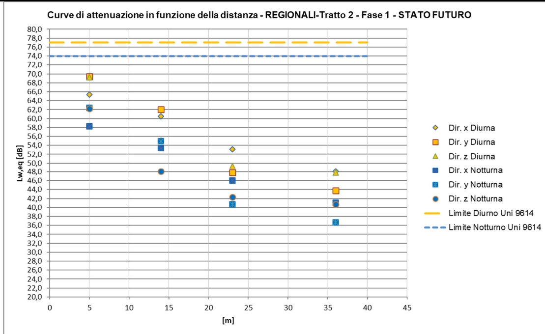
Figura 29 – Curve di attenuazione in funzione della distanza relativa al traffico ferroviario di progetto – Treni Regionale
