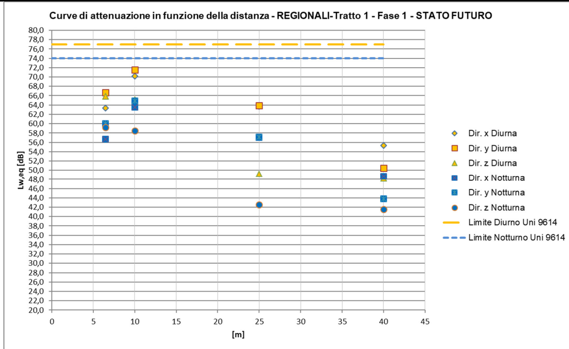
Figura 17 – Curve di attenuazione in funzione della distanza relativa al traffico ferroviario di progetto – Treni Regionale
