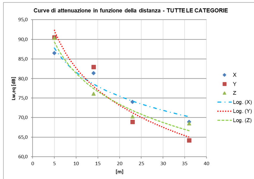
Figura 16 - Curva di attenuazione del L_{w,eq} in funzione della distanza dal binario, ricavata dai rilievi sperimentali sull'attuale linea in esercizio lungo gli assi x,y e z, in corrispondenza delle VIB 01,02, 03 e 04 – TOTALE REGIONALI + METROPOLITANO+MERCATI+IC/EC+ES
