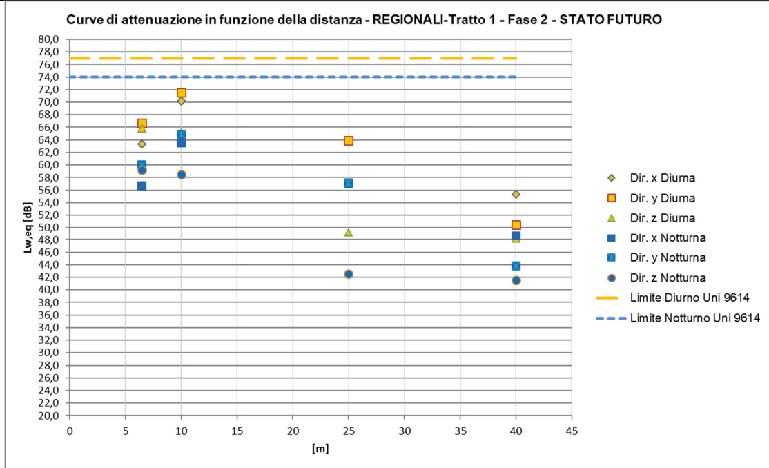
Figura 23 – Curve di attenuazione in funzione della distanza relativa al traffico ferroviario di progetto – Treni Regionali
