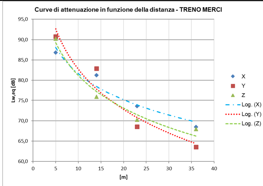
Figura 13 - Curva di attenuazione del L_{w,eq} in funzione della distanza dal binario, ricavata dai rilievi sperimentali sull'attuale linea in esercizio lungo gli assi x,y e z, in corrispondenza delle VIB 01,02, 03 e 04 – TIPOLOGIA TRENO MERCI
