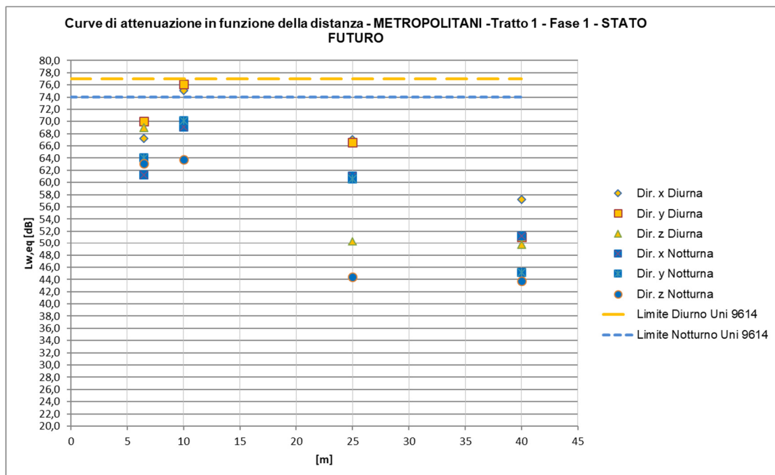
Figura 18 – Curve di attenuazione in funzione della distanza relativa al traffico ferroviario di progetto – Treni Metropolitan
