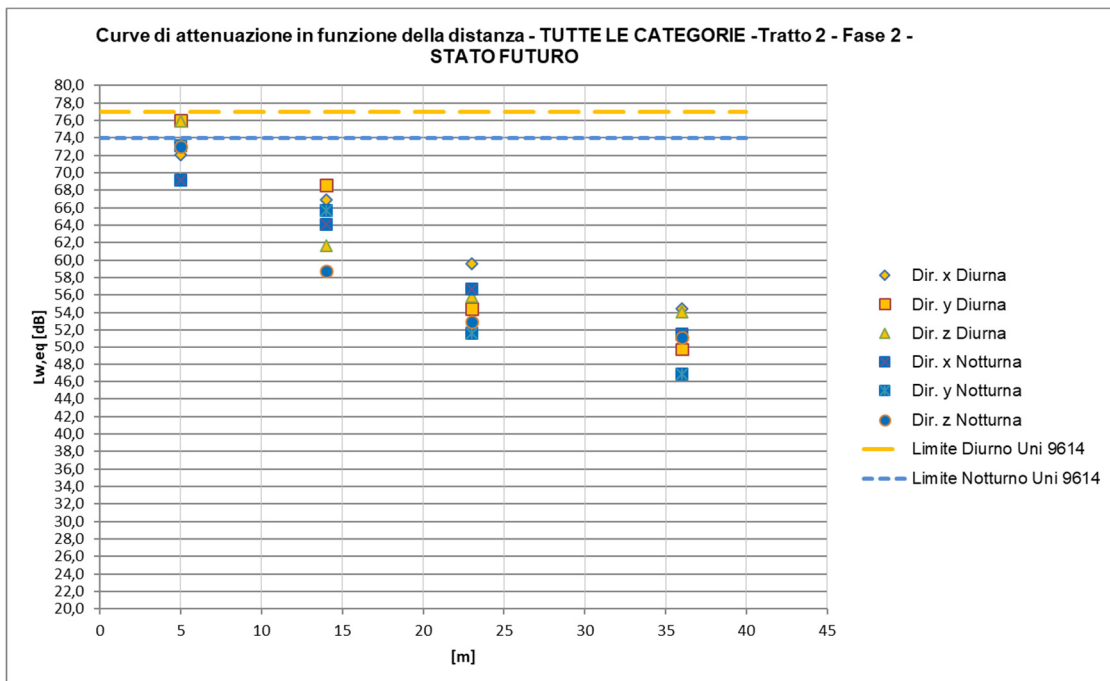
Figura 40 – Curve di attenuazione in funzione della distanza relativa al traffico ferroviario di progetto – Treni Totali Regionali + Metropolitani + Mercati + IC/EC + ES
