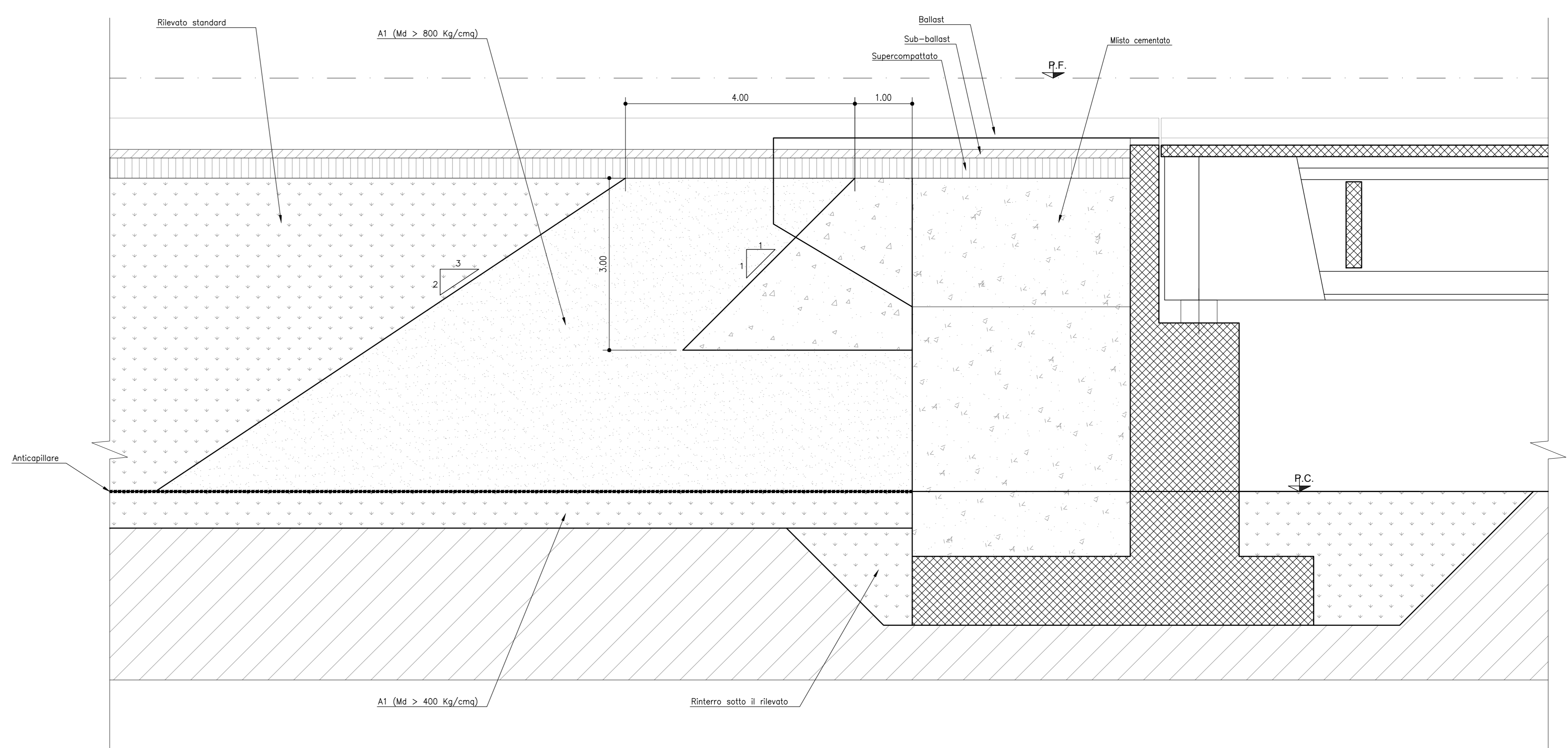
SEZIONE DI TRANSIZIONE RILEVATO-VIADOTTO - H>400 m SCALA 1:10
