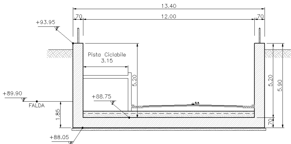
Figura 3: Sezione tipologica
