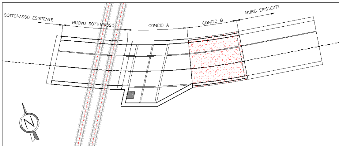
Figura 2 : Planimetria
