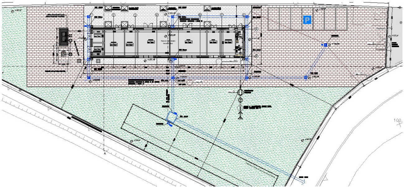
Figura 6.1- Schema idraulico
