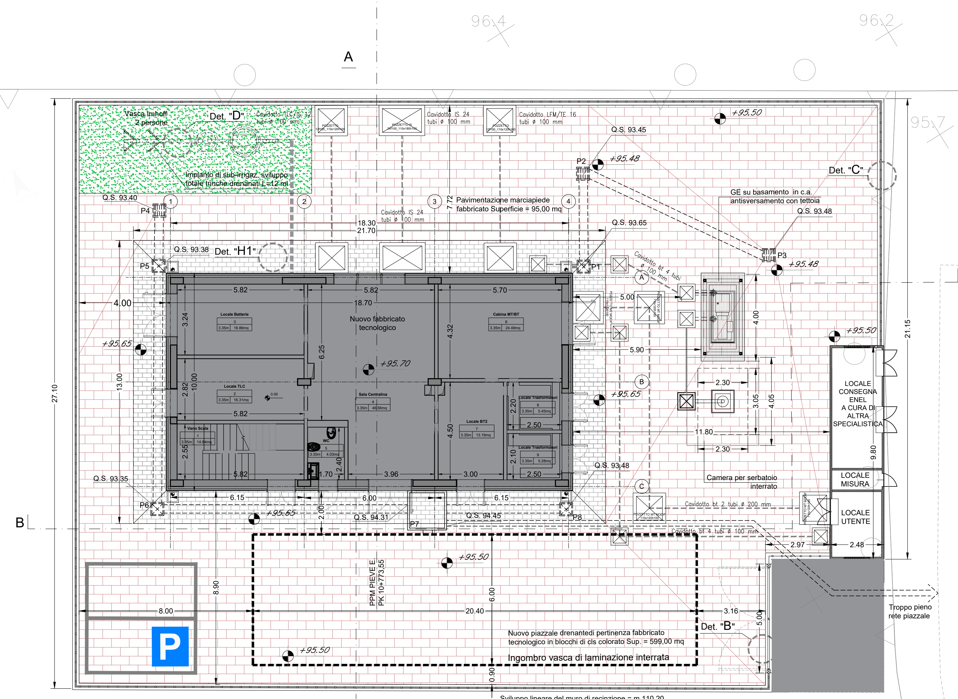
PLANIMETRIA PIAZZALE scala 1:100
