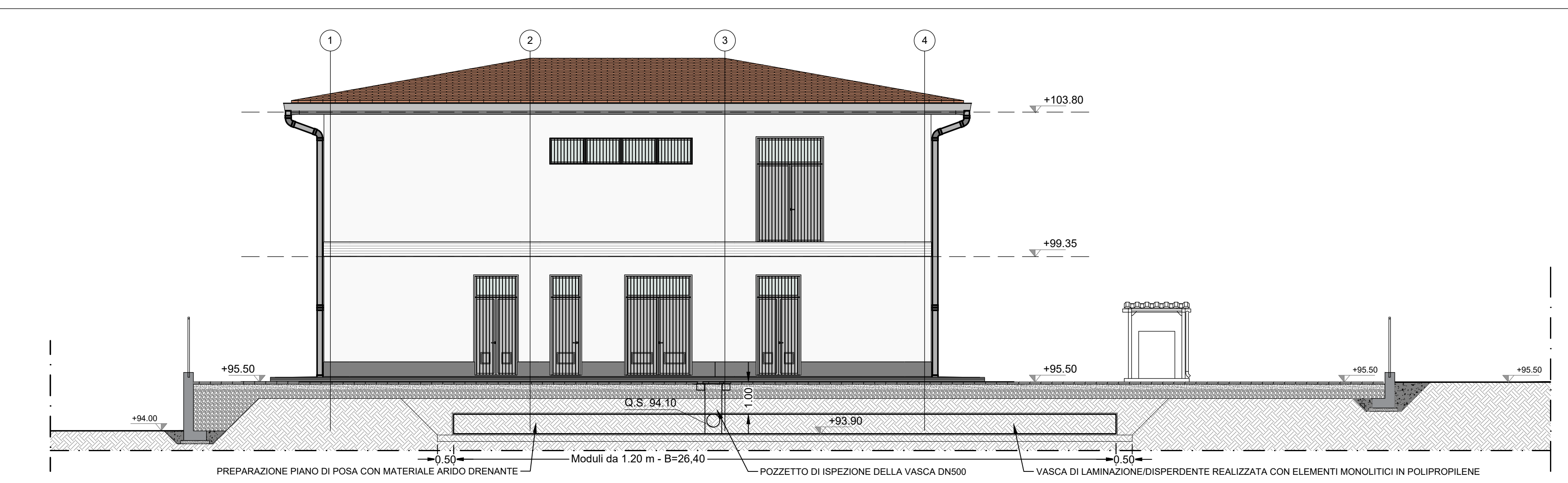
PROSPETTO SEZIONE B-B Scala 1:100
