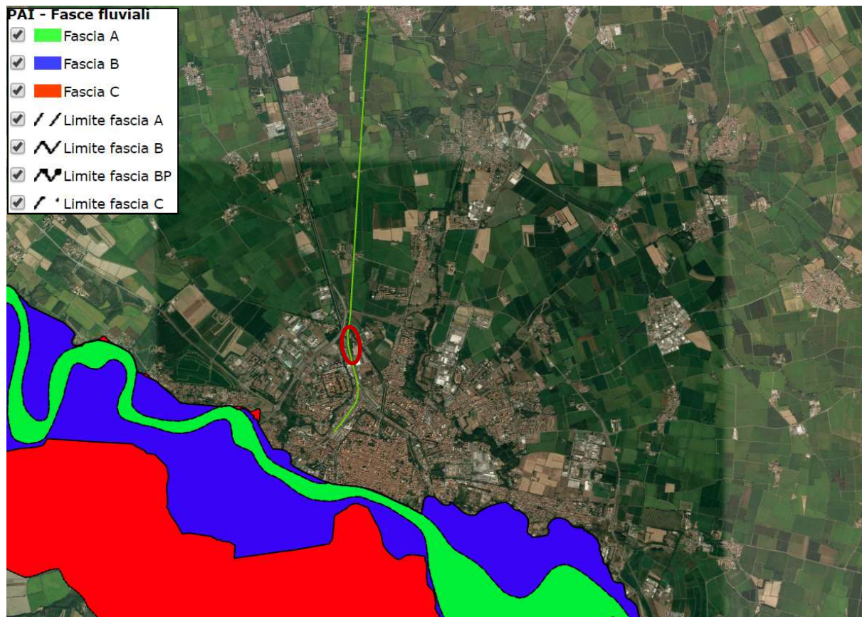
Figura 5.5 – Stralcio planimetrico di delimitazione delle fasce fluviali AdB Po
