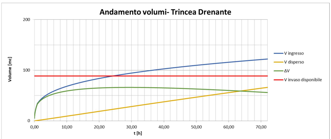
Figura 6.5 - Dimensionamento trincea drenante
