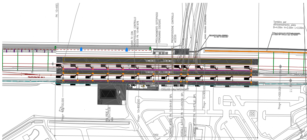
Figura 5 – Stralcio planimetrico elaborato NMOZ10D26P8FV020B001A
