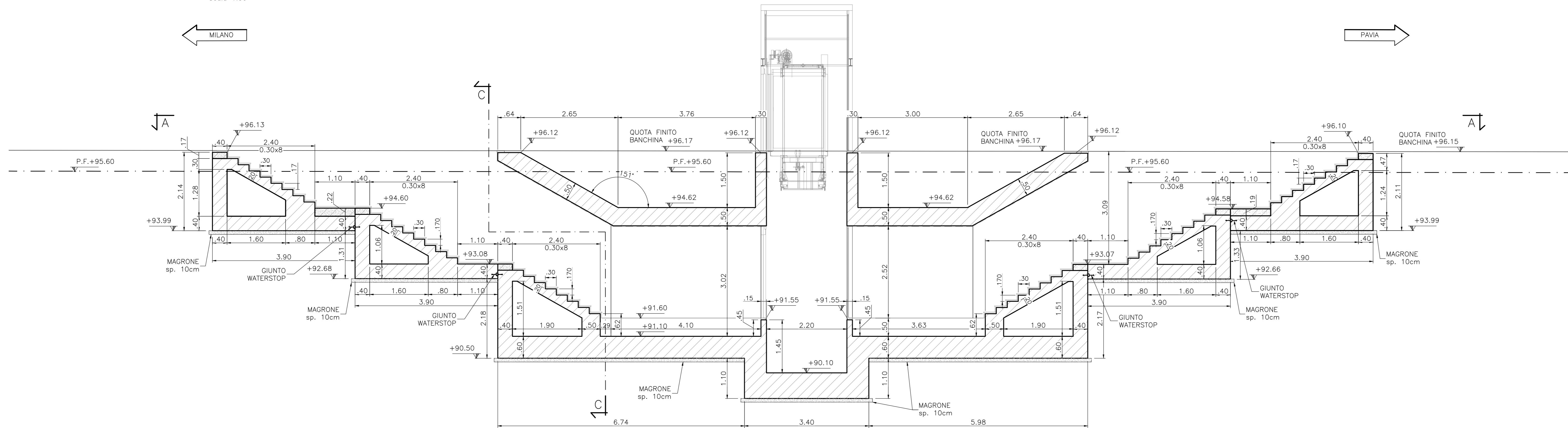
SEZIONE C-C Scala 1:50
