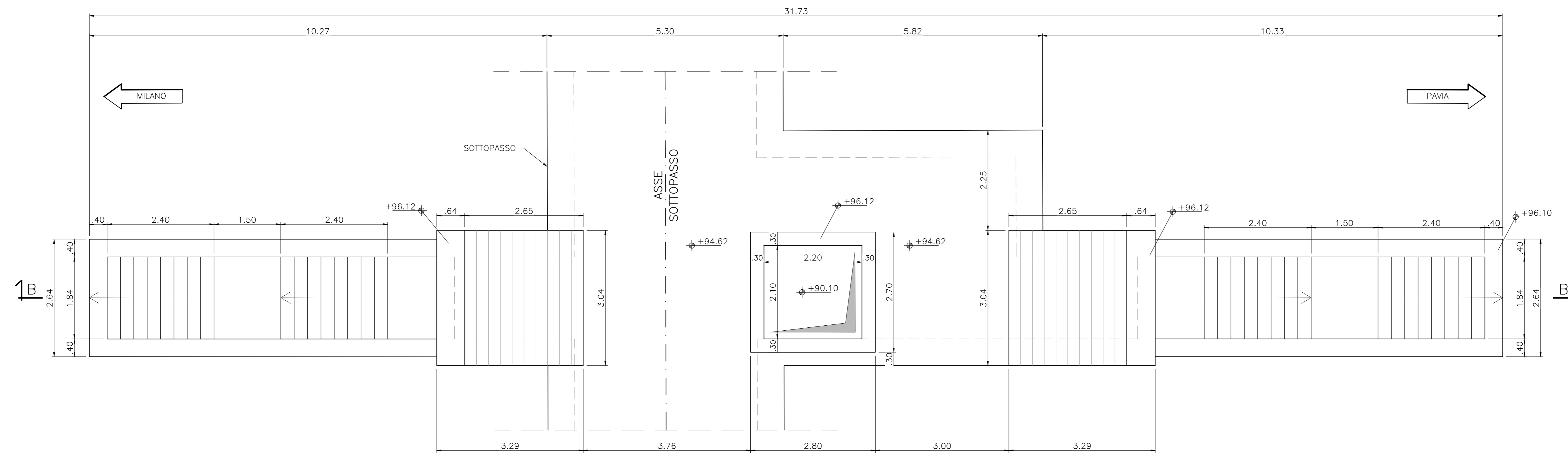
PIANTA A-A Scala 1:50
