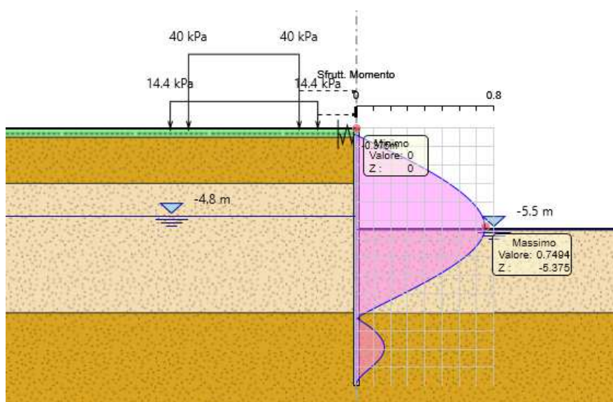
Figura 8-2: Tasso di sfruttamento momento flettente - Fase: realizzazione dello scavo - A1+M1+R1
