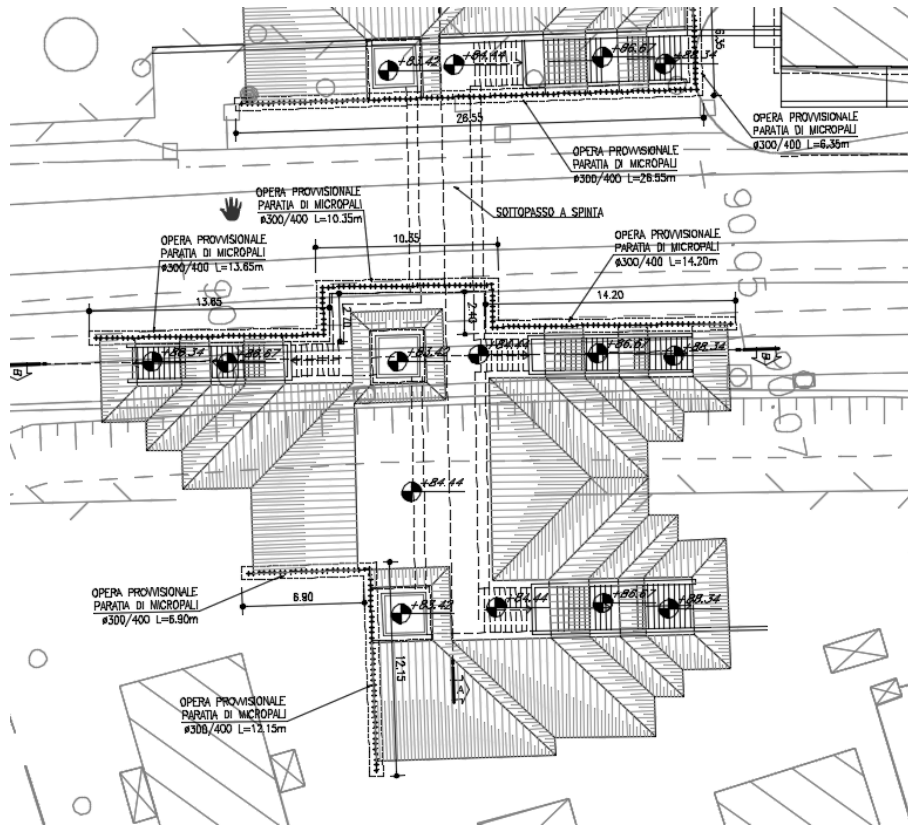
Figura 2: Vista in pianta dell'opera da realizzare
