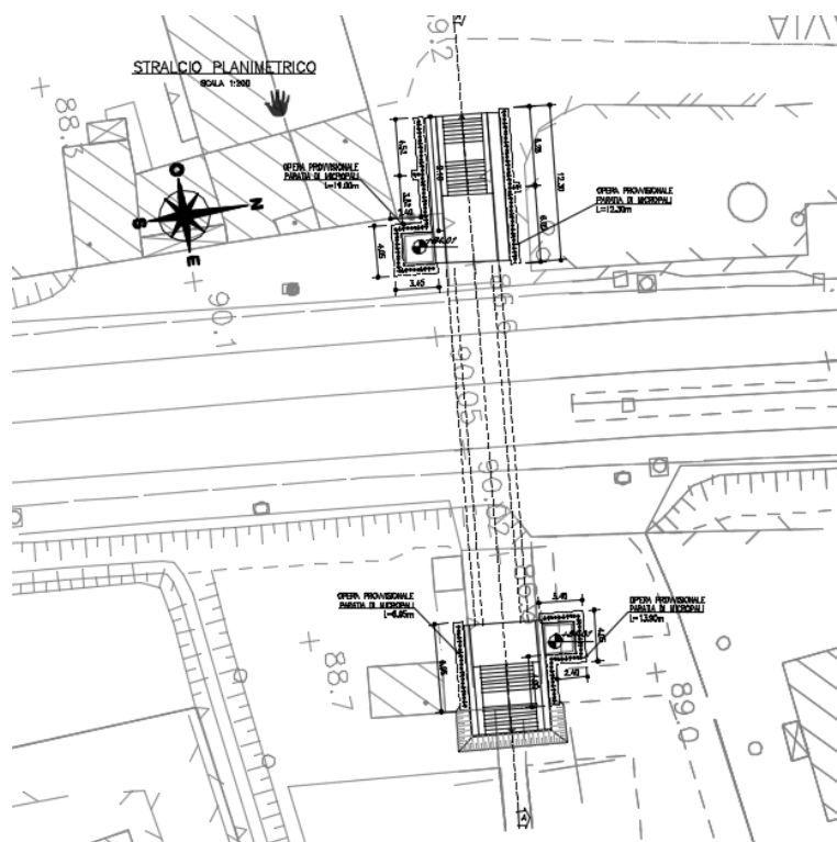
Figura 2: Vista in pianta dell'opera da realizzare
