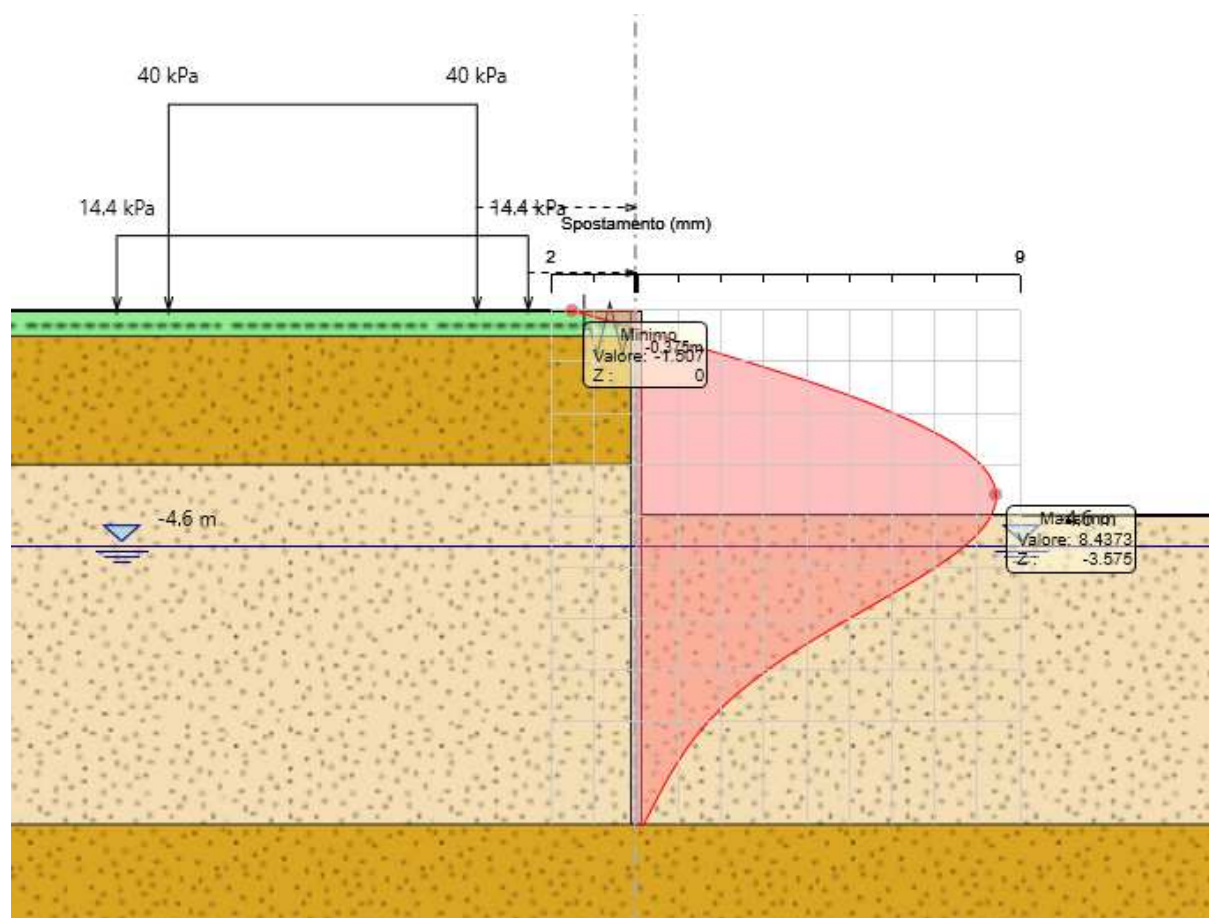
Figura 9-1: Spostamenti massimi agli SLE
