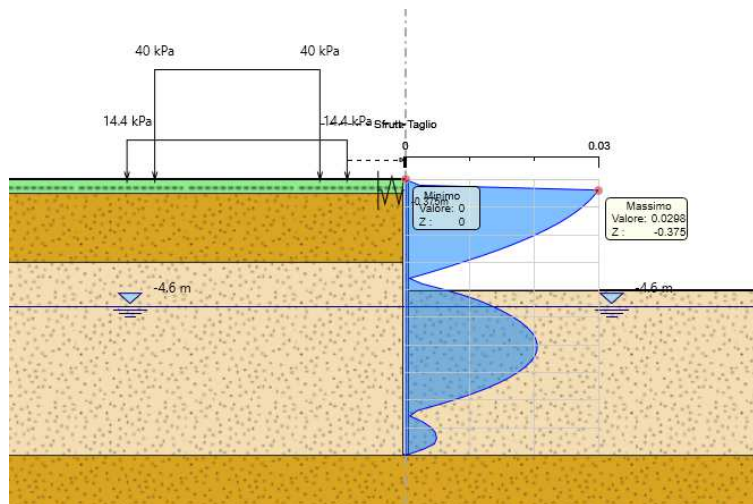
Figura 8-4: Tasso di sfruttamento taglio - Fase: realizzazione dello scavo – A2+M2+R1
