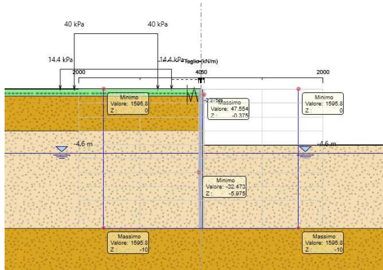
Figura 8-3: Diagrammi taglio - Fase: realizzazione dello scavo – A2+M2+R1
