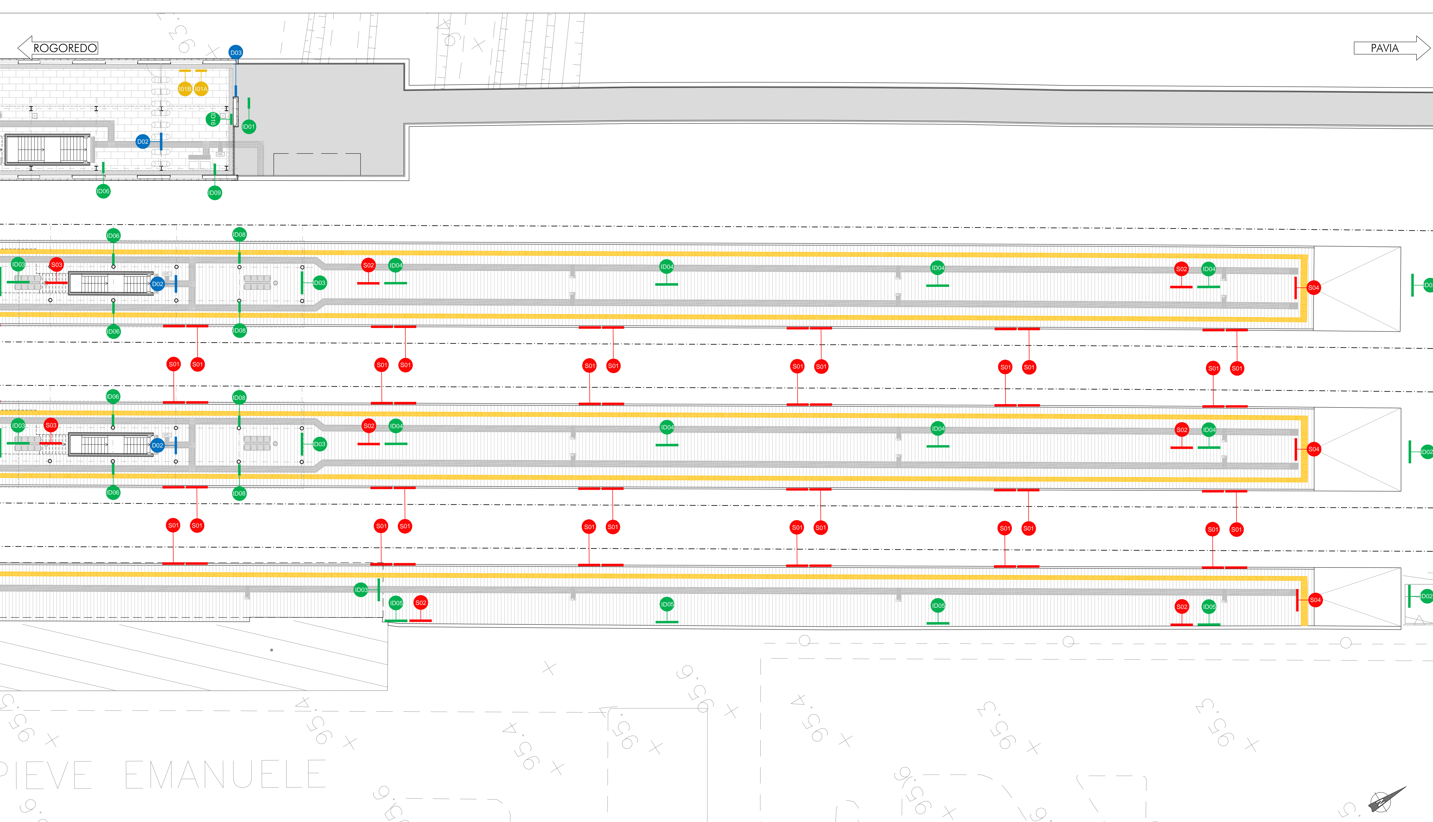
B PIANTA QUOTA BANCHINA 1:200
