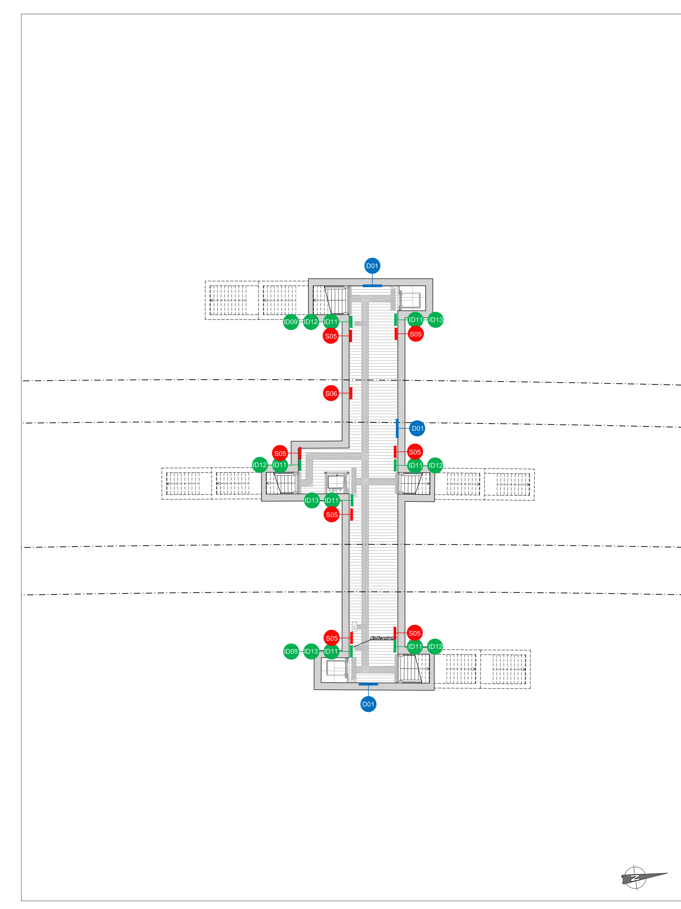
C PIANTA QUOTA SOTTOPASSO 1:200
