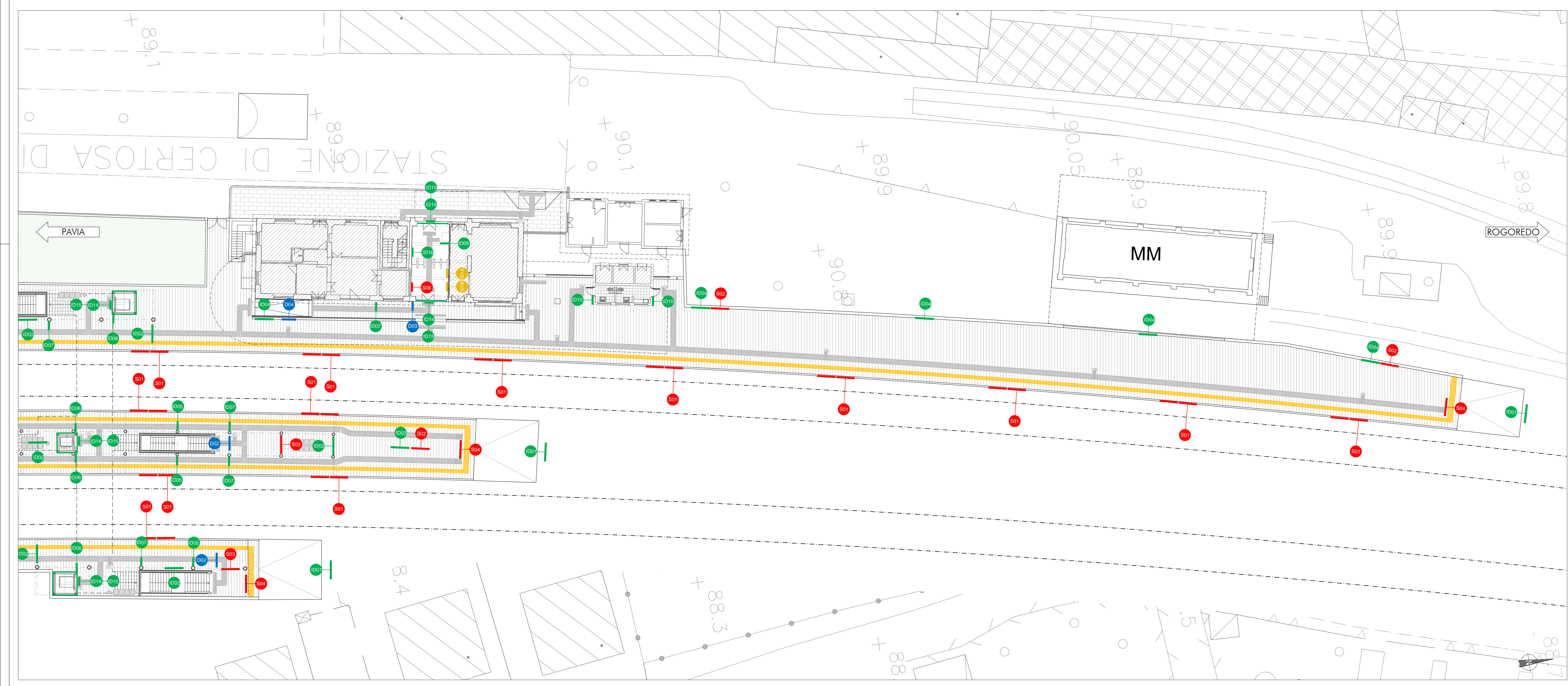
B PIANTA QUOTA BANCHINA 1:200
