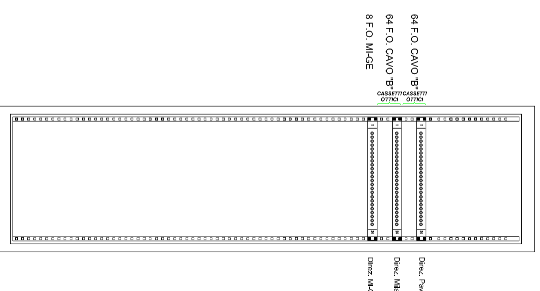
Telaio N3 per cassette olti 600X300X2200 mm
