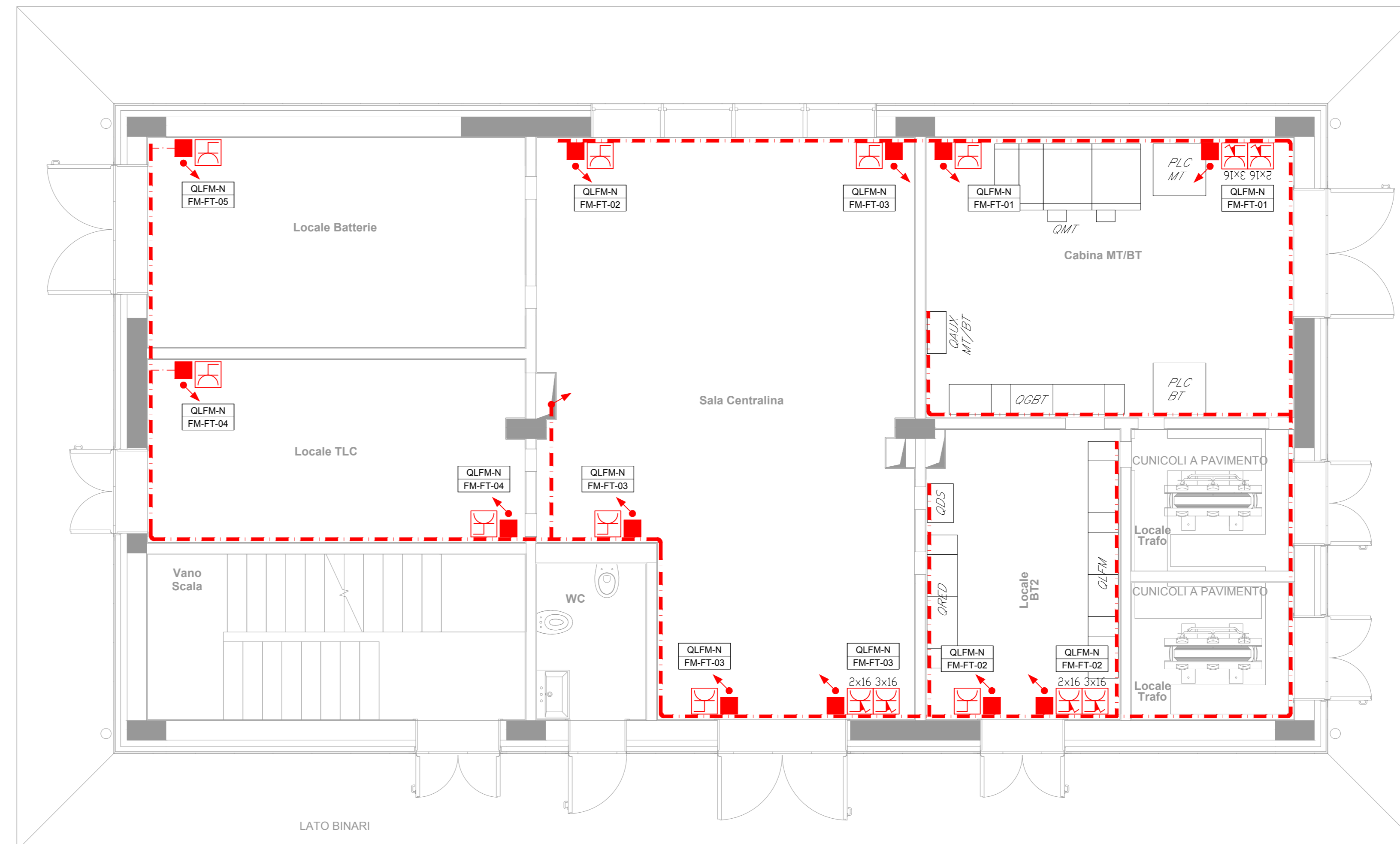
PIANTA PIANO TERRA (FORZA MOTTRICE)
