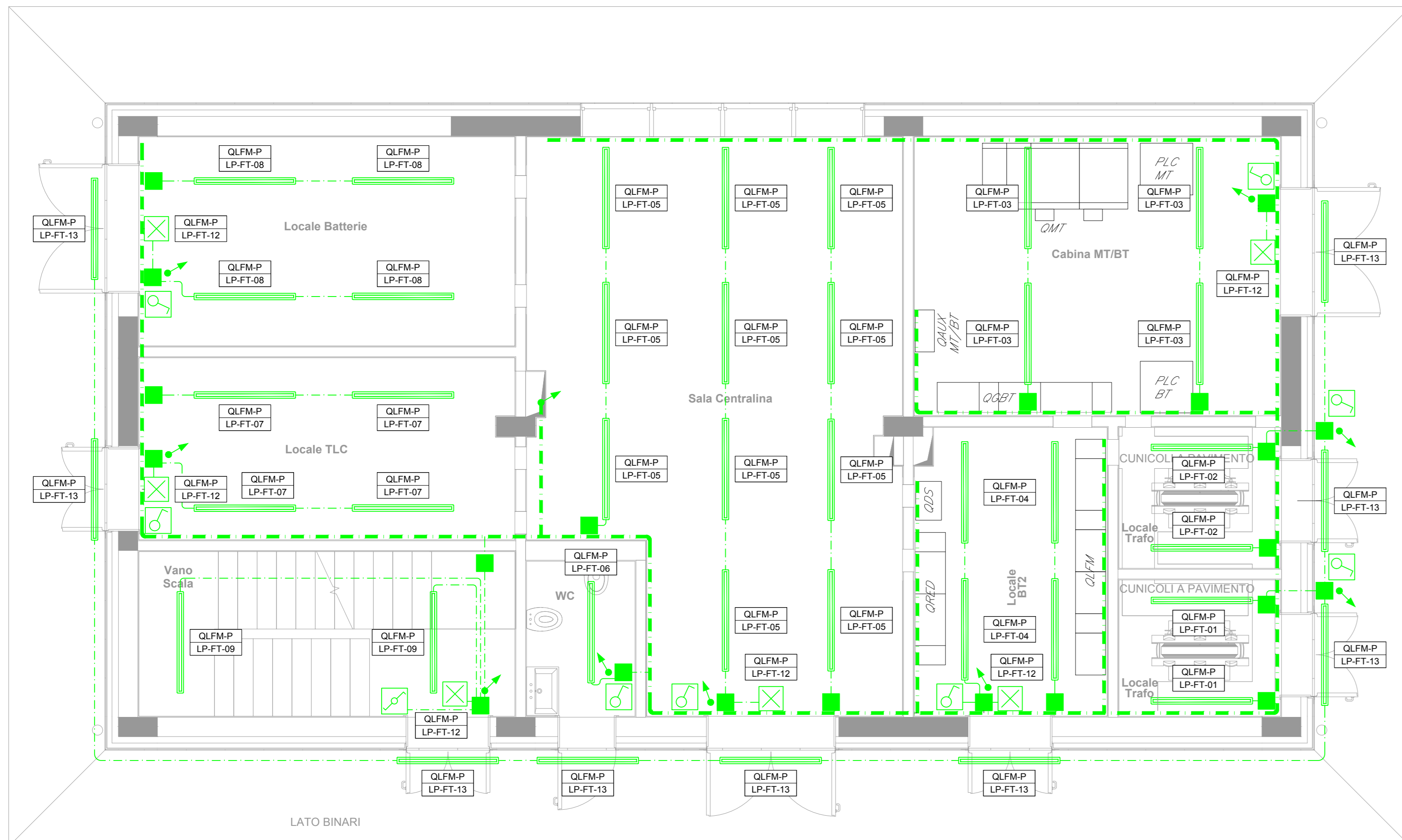
PIANTA PIANO TERRA (LUCI)
