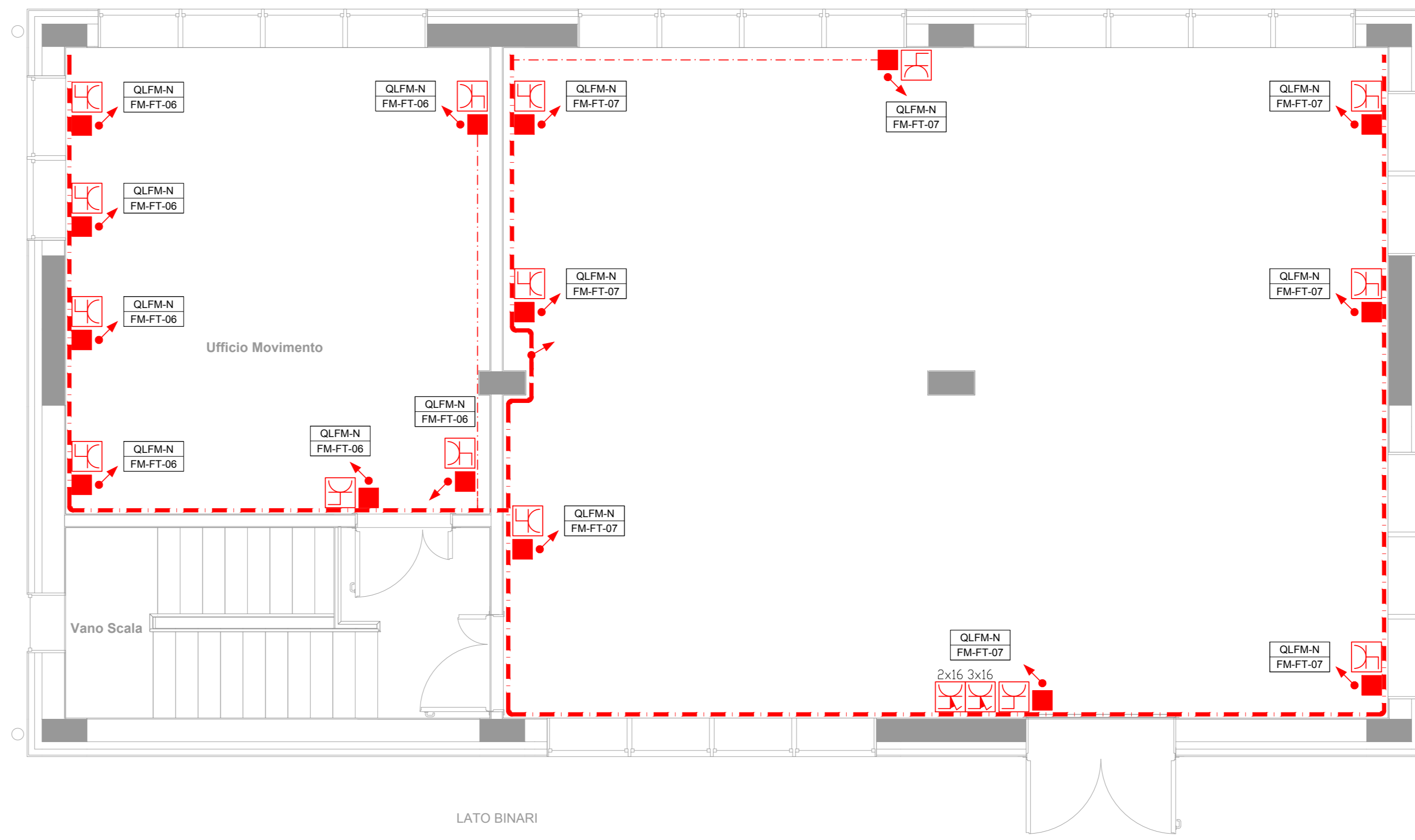
PIANTA PIANO PRIMO (FORZA MOTTRICE)
