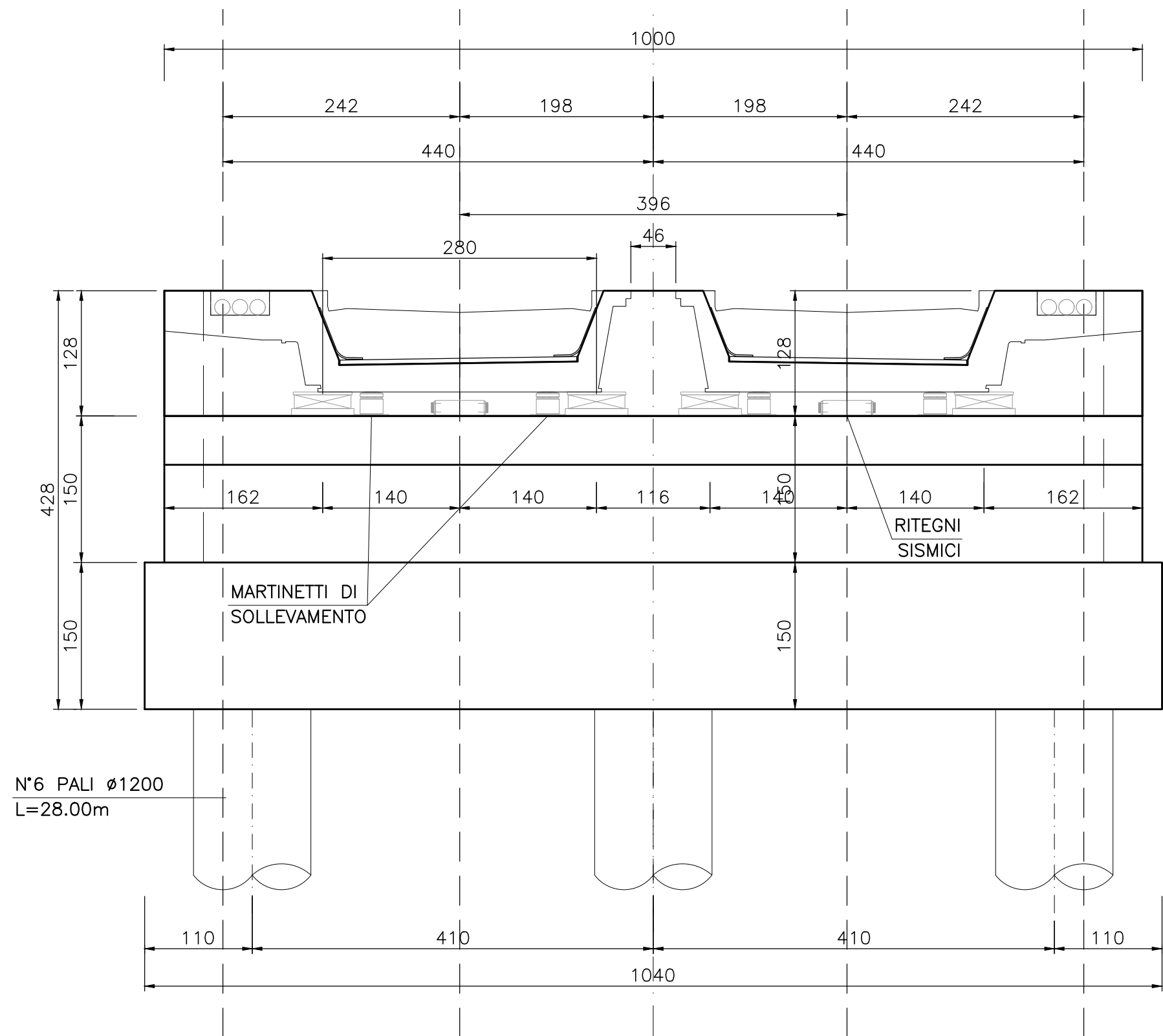
VISTA IN RETTO
