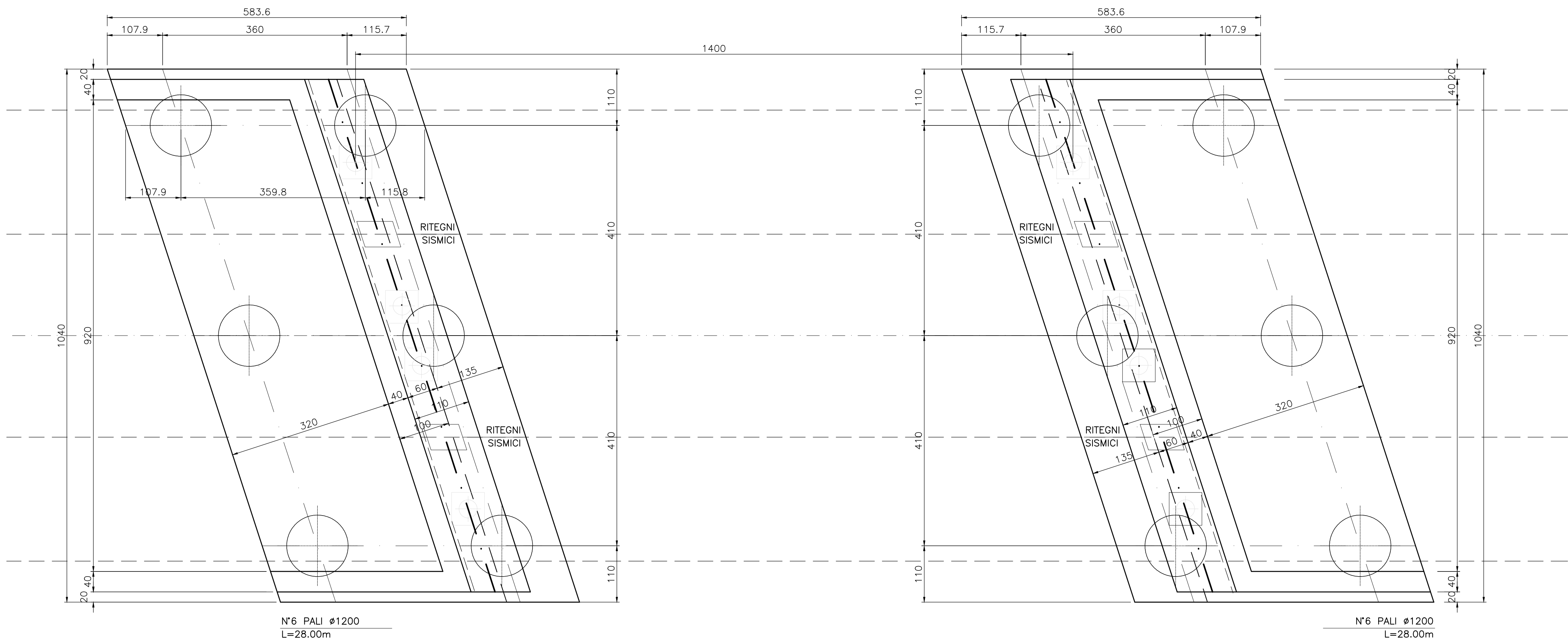
PIANTA DELLE FONDAZIONI
