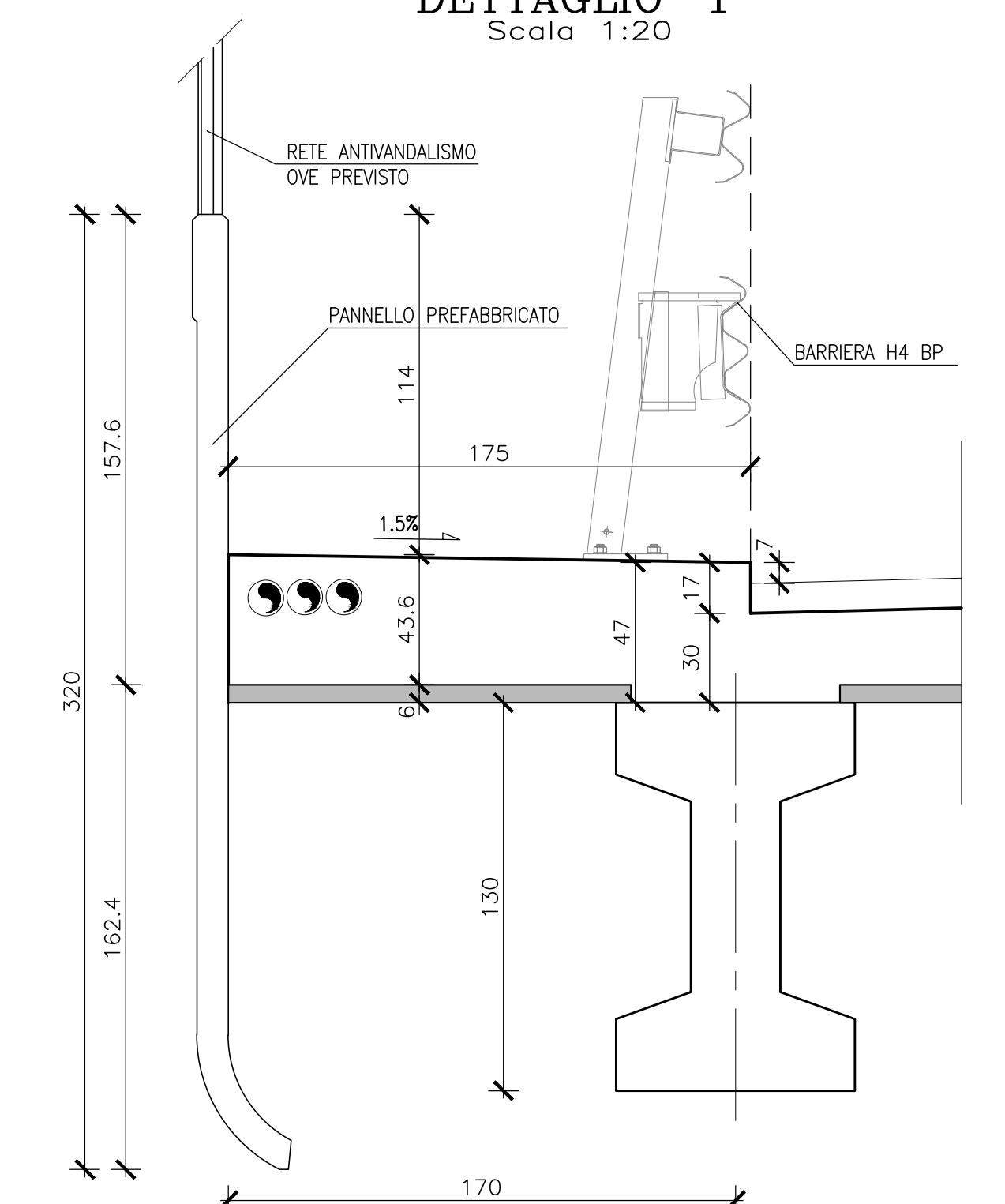
DETTAGLIO '1' Scala 1:20
