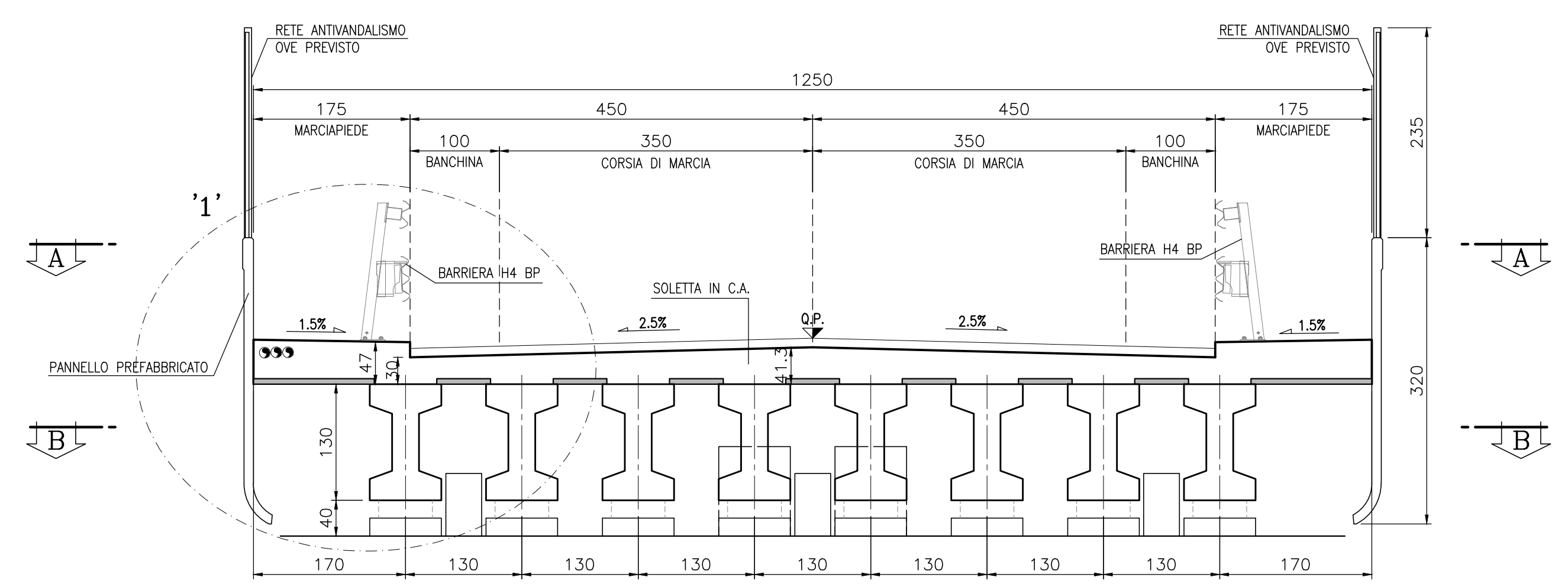
SEZIONE TRASVERSALE Scala 1:50
