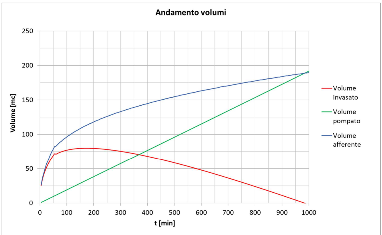
Figura 6.2 – Dimensionamento vasca volano
