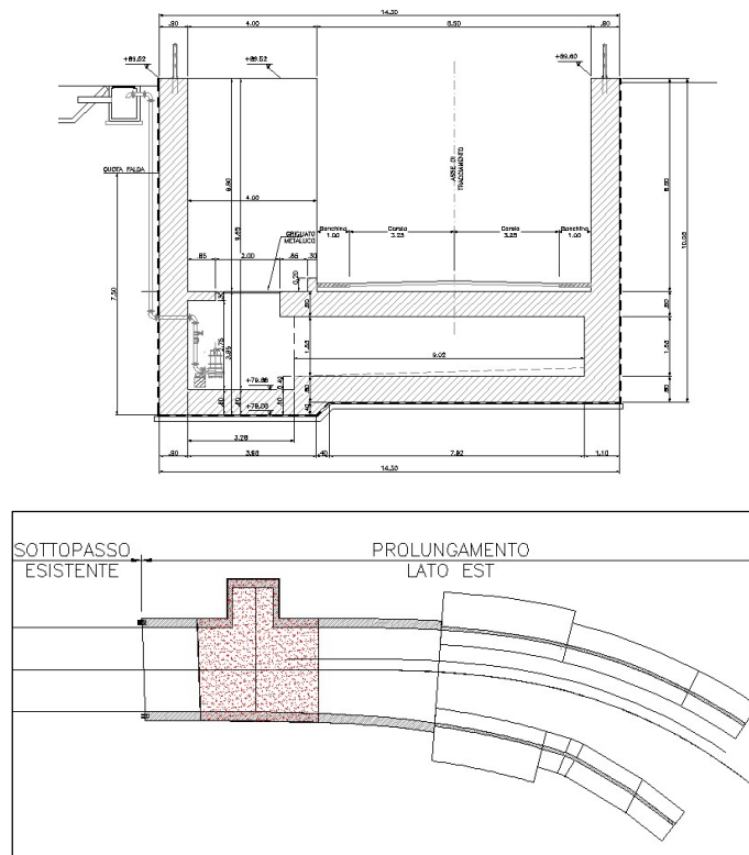
Figura 6.1 – Vasca volano
