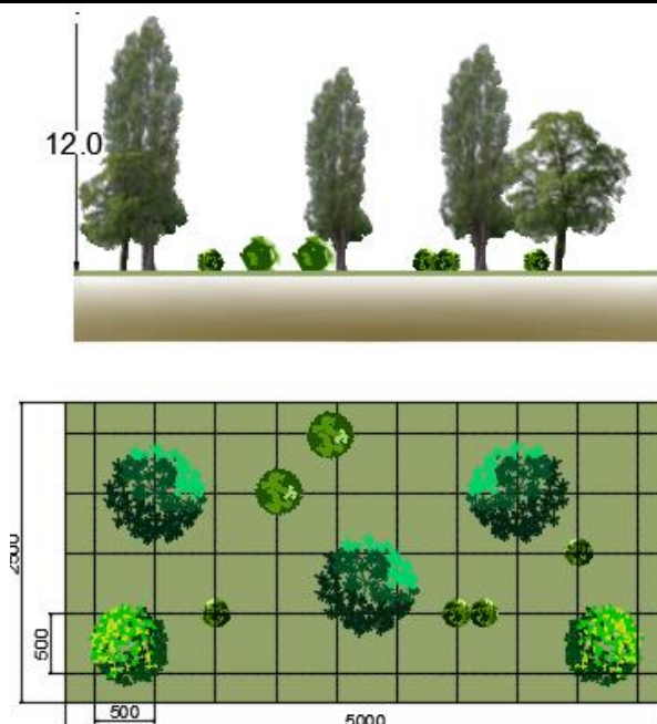
Figura 2-5: Modulo E – Prato arborato
