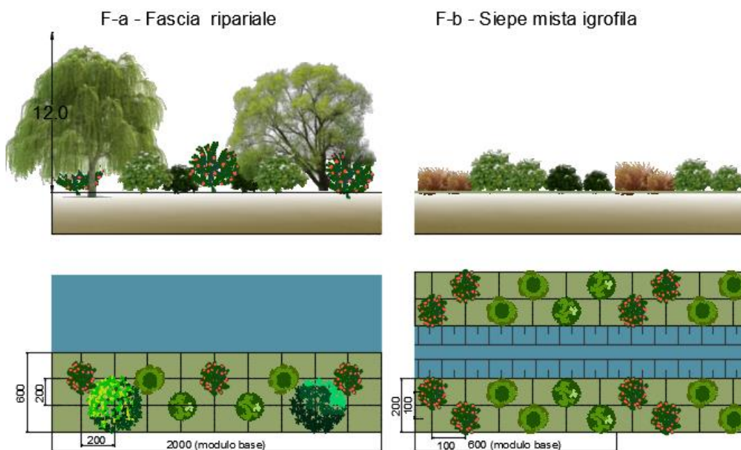
Figura 2-6: Modulo F – Sistemazione vegetale spondale
