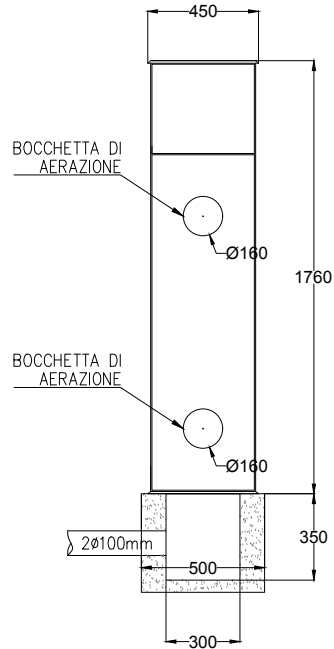
VISTA LATERALE
