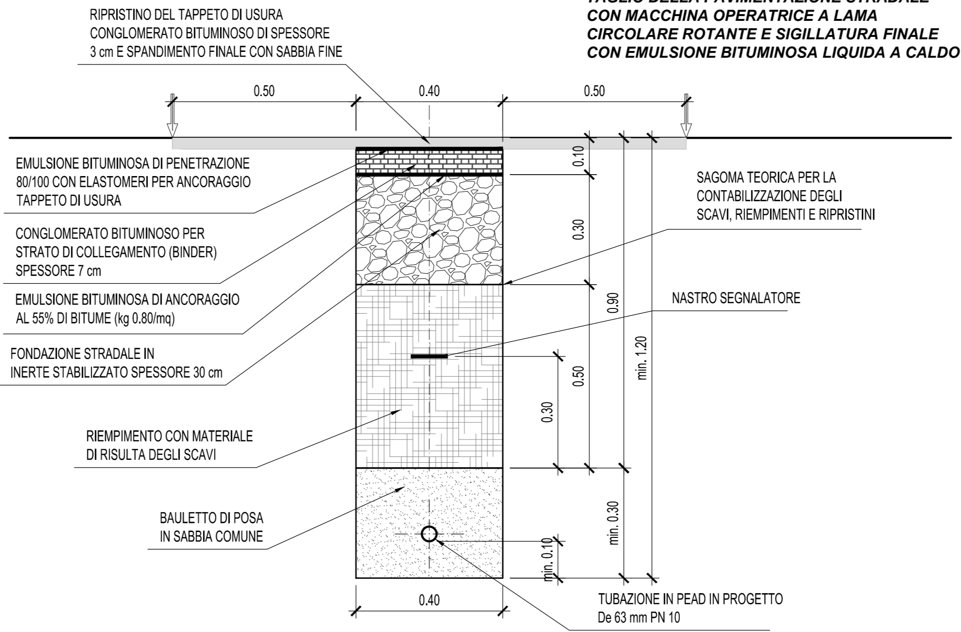
SEZIONE TIPO DI SCAVO SU STRADA ASFALTATA Scala 1:10
