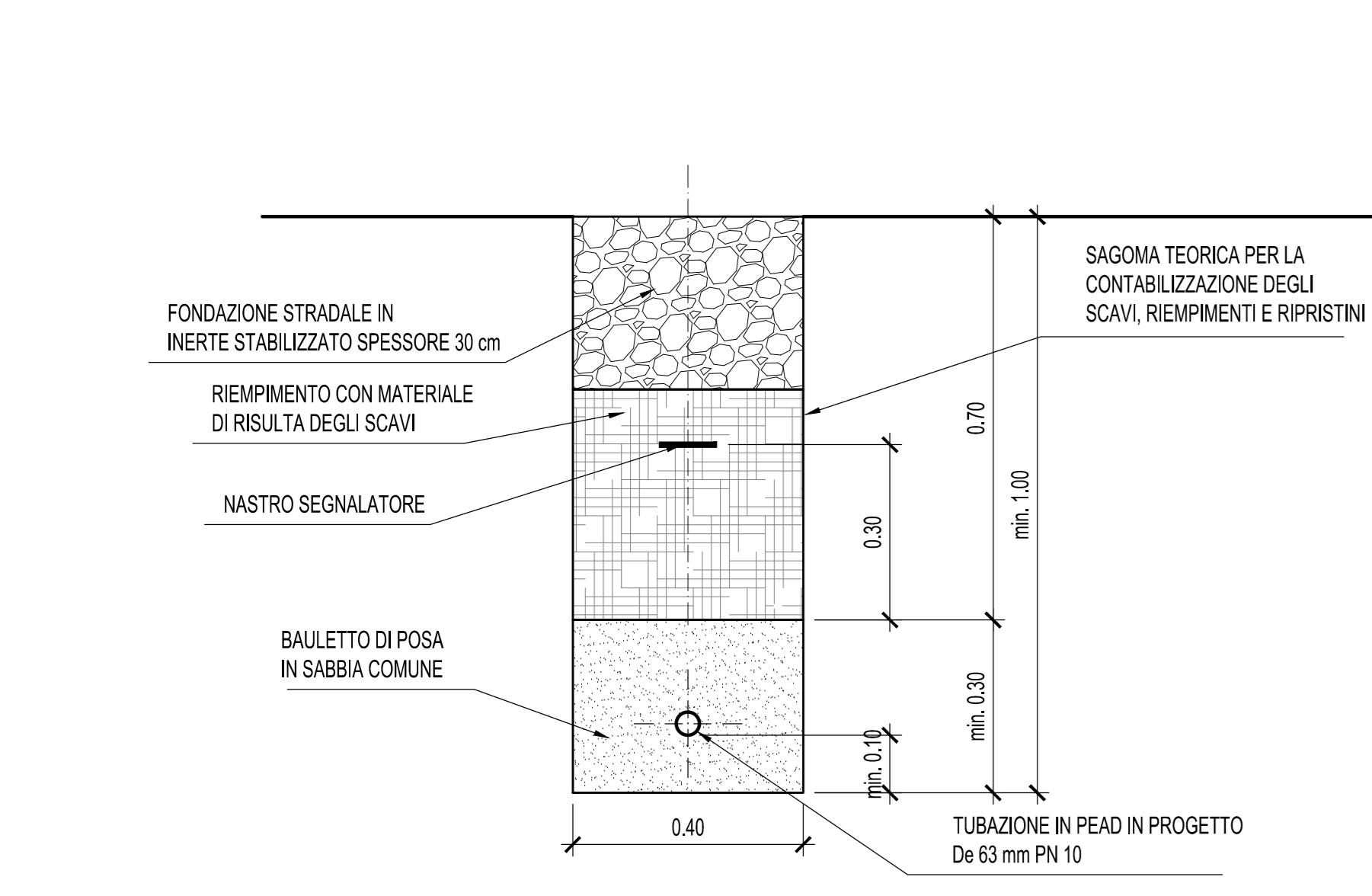
SEZIONE TIPO DI SCAVO SU STRADA STERRATA Scala 1:10
