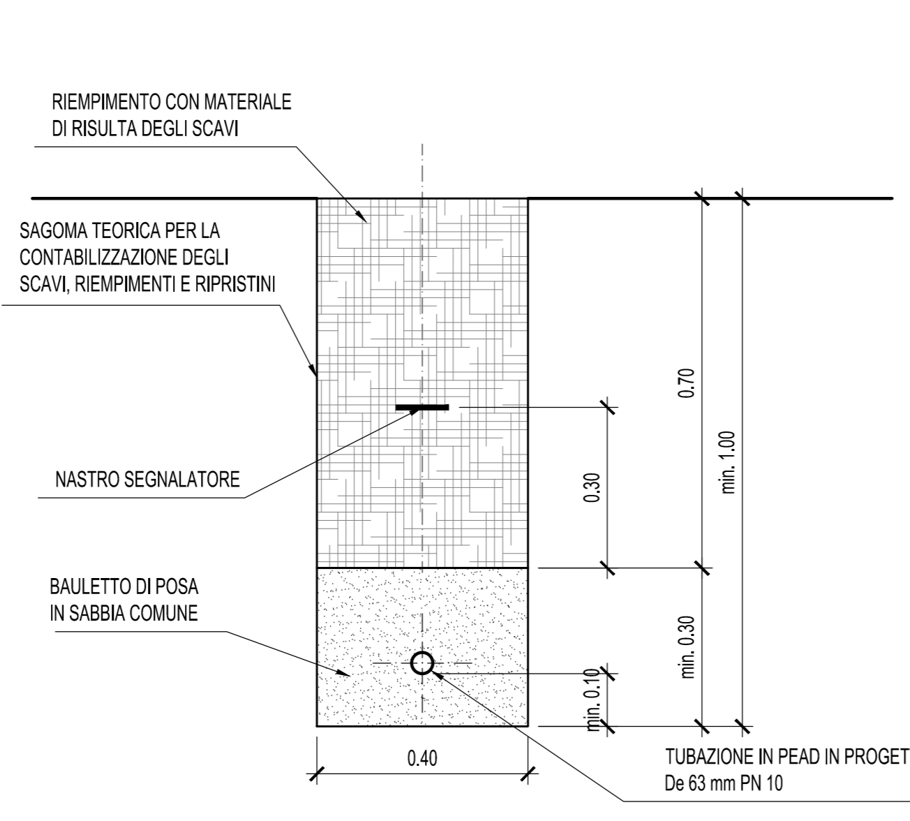
SEZIONE TIPO DI SCAVO SU TERRENO NATURALE Scala 1:10
