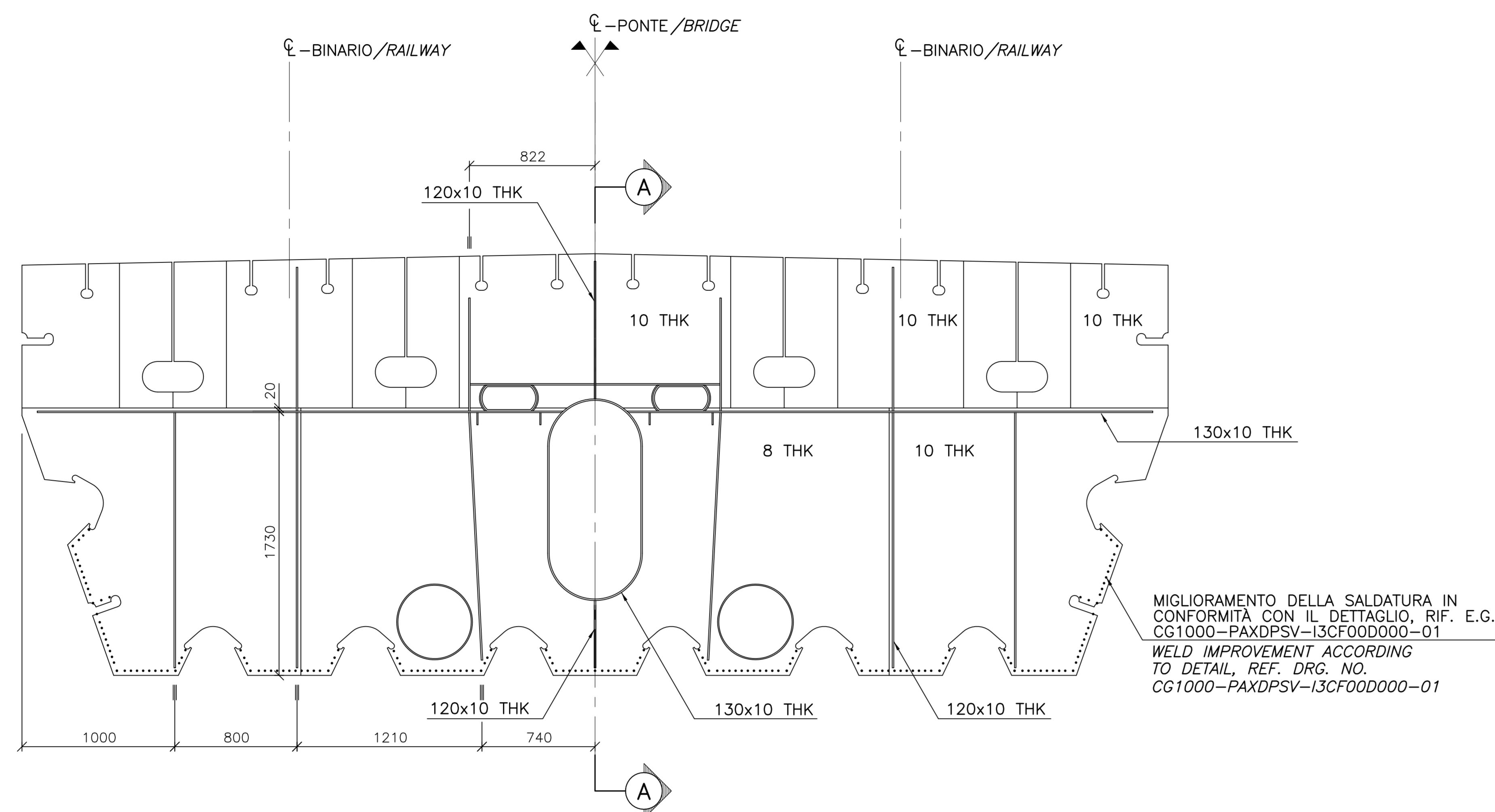
SEZIONE A-A SCALA 1:50 CASSONE FERROVIARIO TIPO CF3. MOSTRATA CAMPATA LATERALE. CAMPATA PRINCIPALE SIMILE. PER IL GIUNTO AL TRAVESSO, RIF. E.G. CG1000-PBXDPSV-I3CF00D000-01 SECTION A-A SCALE 1:50 RAILWAY GIRDER TYPE CF3. SIDE SPAN SHOWN. MAIN SPAN SIMILAR. FOR JOINT AT CROSS GIRDER, REF. DRG. NO. CG1000-PBXDPSV-I3CF00D000-01
