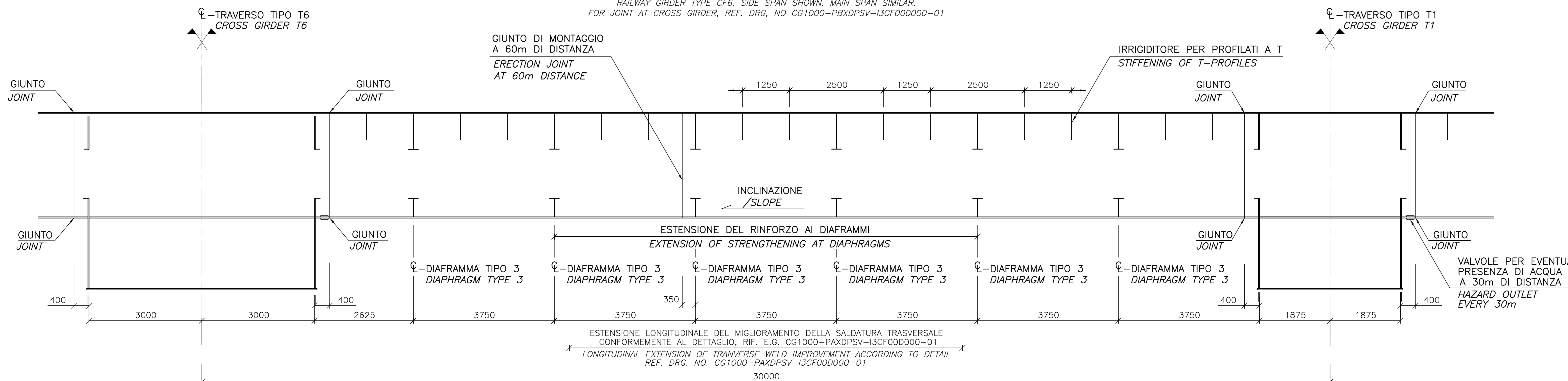
SEZIONE A-A SCALA 1:50 CASSONE FERROVIARIO TIPO CF6. MOSTRATA CAMPATA LATERALE. CAMPATA PRINCIPALE SIMILE. PER IL GIUNTO AL TRAVESSO, RIF. E.G. CG1000-PBXDPSV-I3CF00D000-01 SECTION A-A SCALE 1:50 RAILWAY GIRDER TYPE CF6. SIDE SPAN SHOWN. MAIN SPAN SIMILAR. FOR JOINT AT CROSS GIRDER, REF. DRG. NO. CG1000-PBXDPSV-I3CF00D000-01
