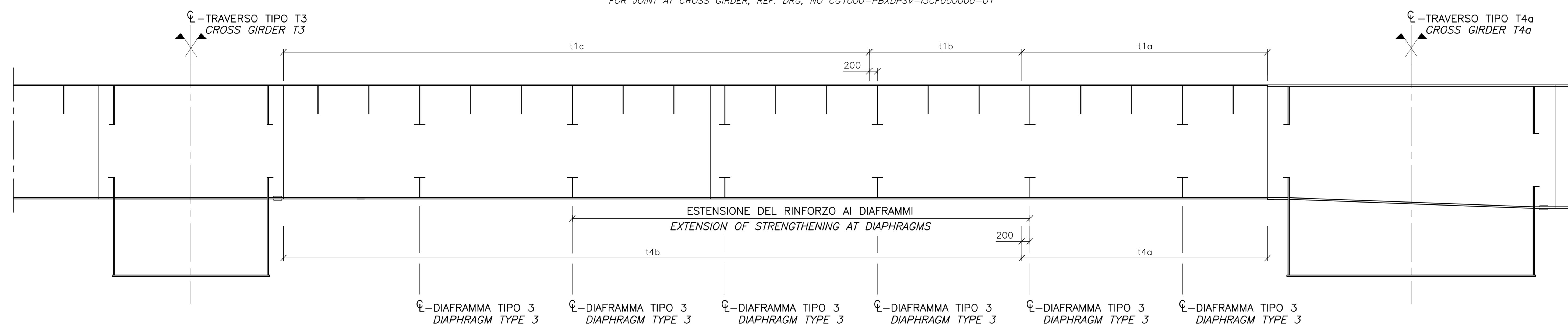
SEZIONE A-A SCALA 1:50 CASSONE FERROVIARIO TIPO CF6. MOSTRATA CAMPATA LATERALE. CAMPATA PRINCIPALE SIMILE. PER IL GIUNTO AL TRAVESSO, RIF. E.G. CG1000-PBXDPSV-I3CF00D000-01 SECTION A-A SCALE 1:50 RAILWAY GIRDER TYPE CF6. SIDE SPAN SHOWN. MAIN SPAN SIMILAR. FOR JOINT AT CROSS GIRDER, REF. DRG. NO. CG1000-PBXDPSV-I3CF00D000-01
