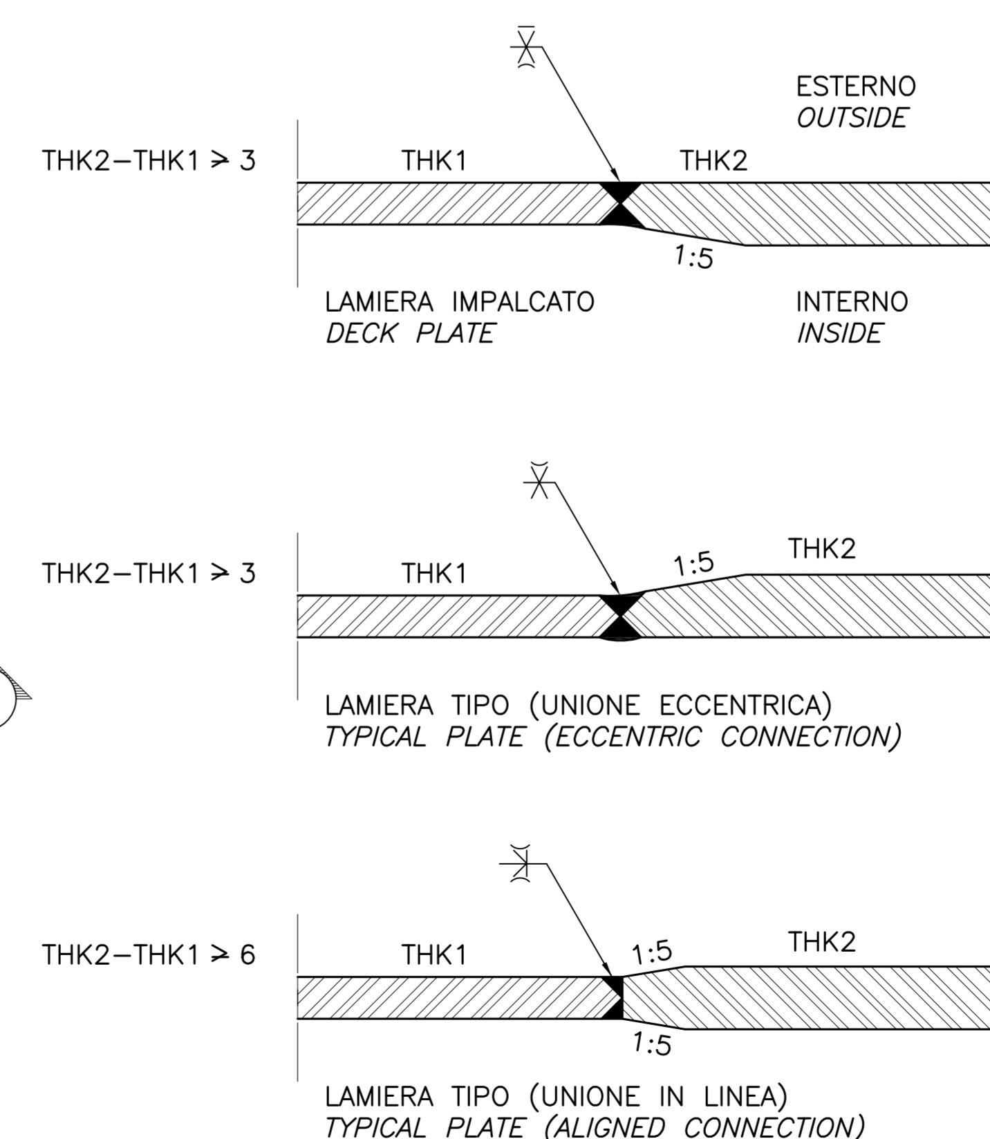
SALDATURE TIPO TRA LAMIERE DI SPESSORI DIVERSI SCALA 1:2 TYPICAL WELDING BETWEEN PLATES OF DIFFERENT THICKNESS SCALE 1:2
