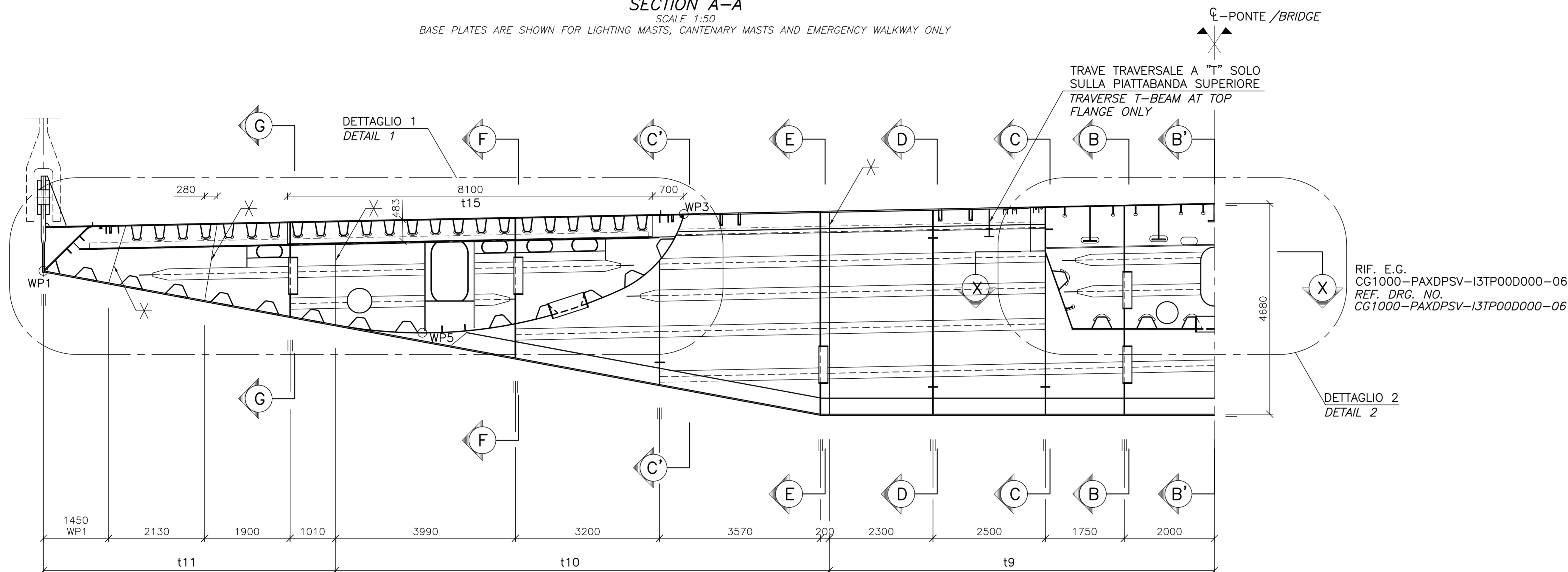
PIATTABANDA SUPERIORE SCALA 1:50 SONO MOSTRATE SOLO LE PIASTRE DI BASE PER I PALI DELLA LUCE ED I PALI DELLA CATENARIA TOP FLANGE SCALE 1:50 BASE PLATES ARE SHOWN FOR LIGHT MASTS AND CANTENARY MASTS ONLY
