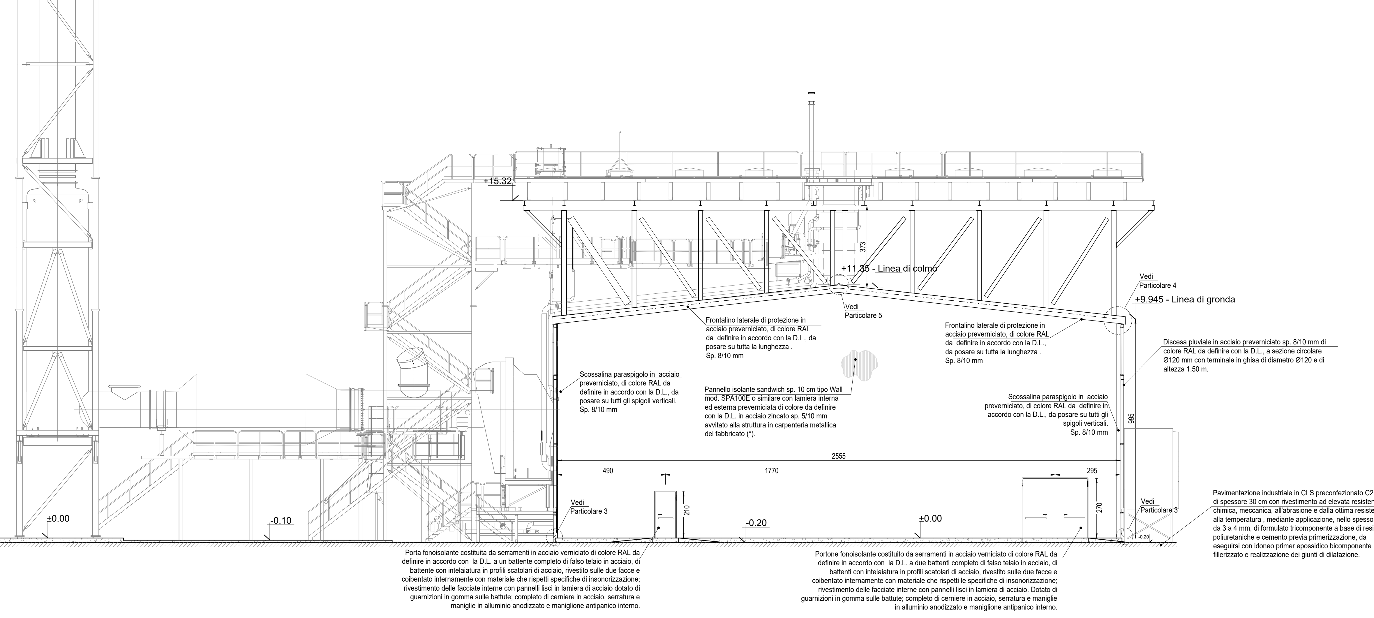
PROSPETTO 4 Scala: 1:100
