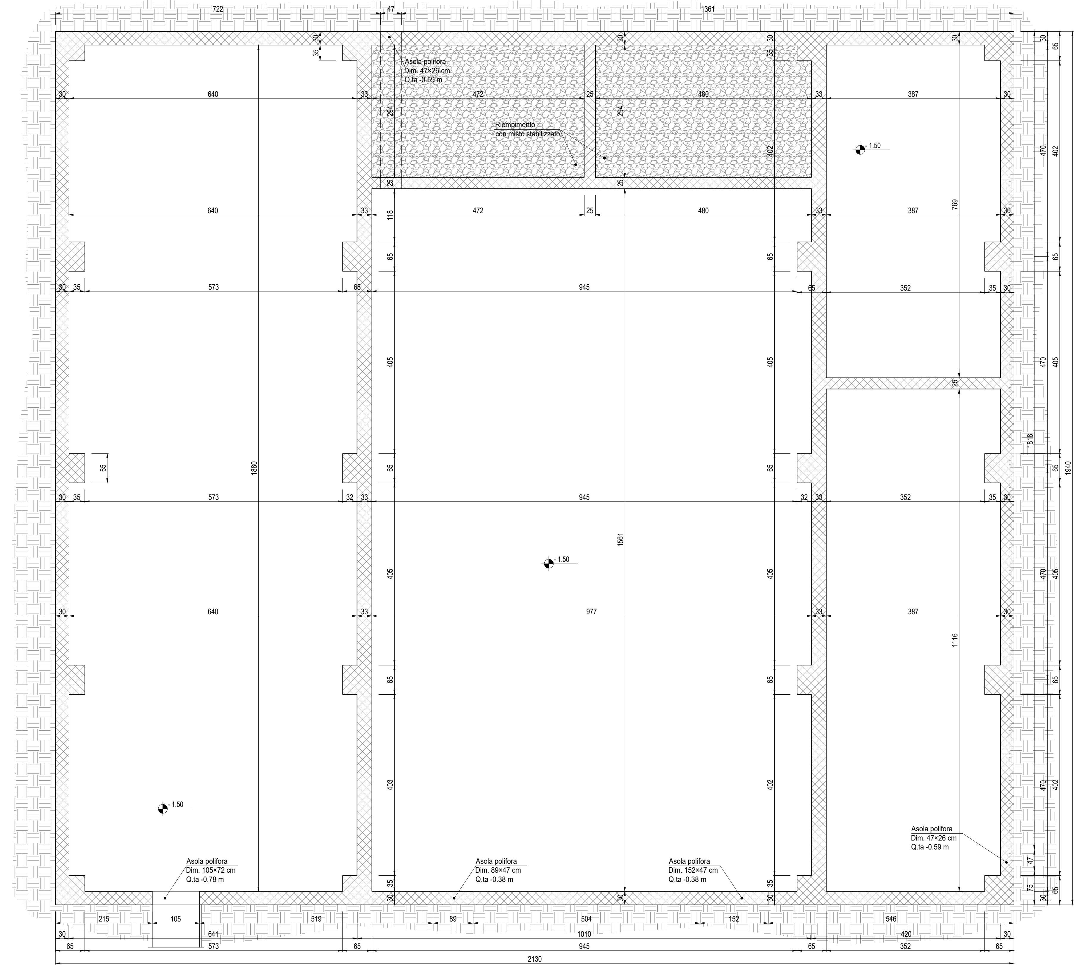
PIANTA Q.TA -1.50 m Scala: 1:50
