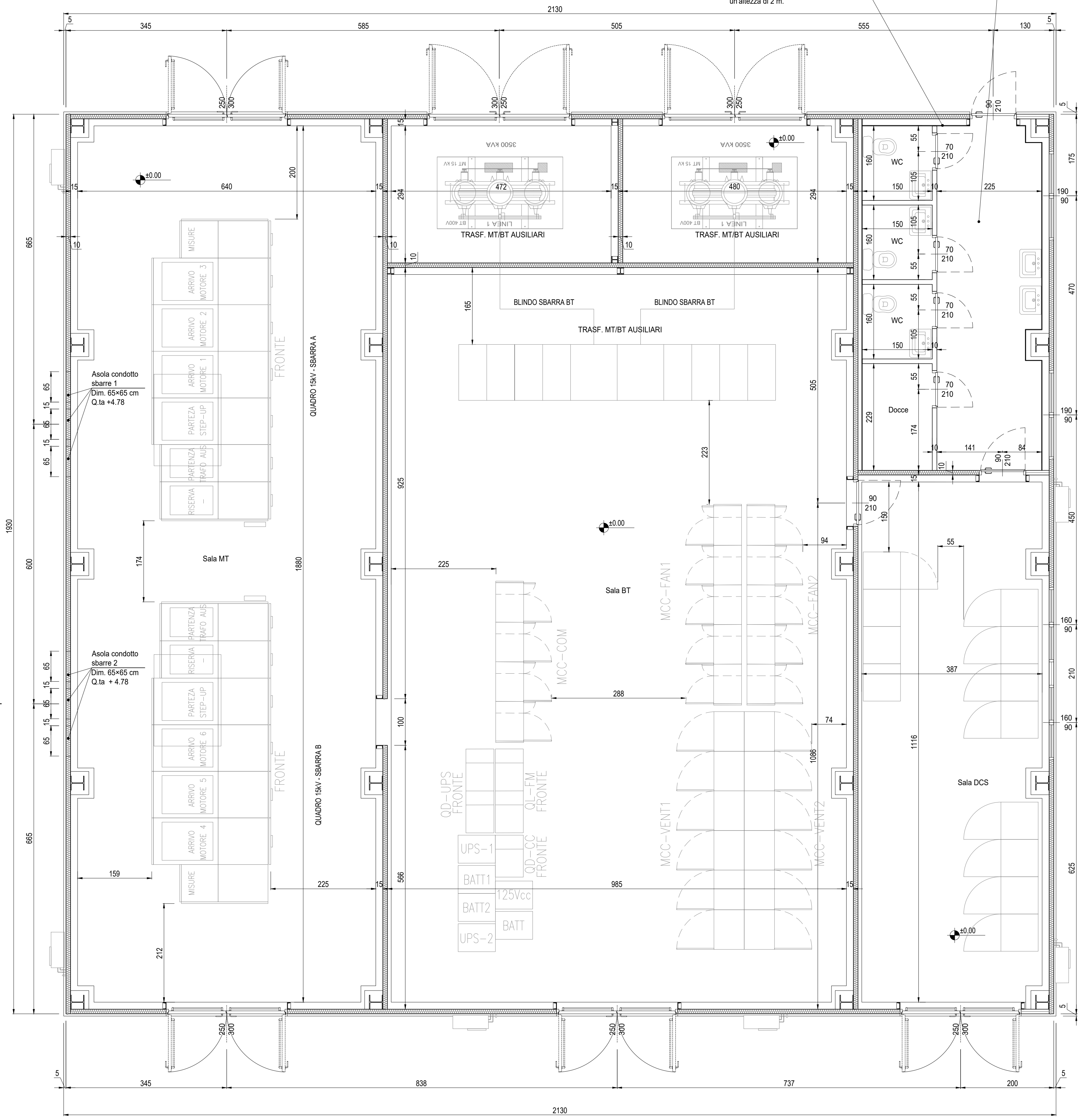
PIANTA Q.TA ±0.00 m Scala: 1:50
