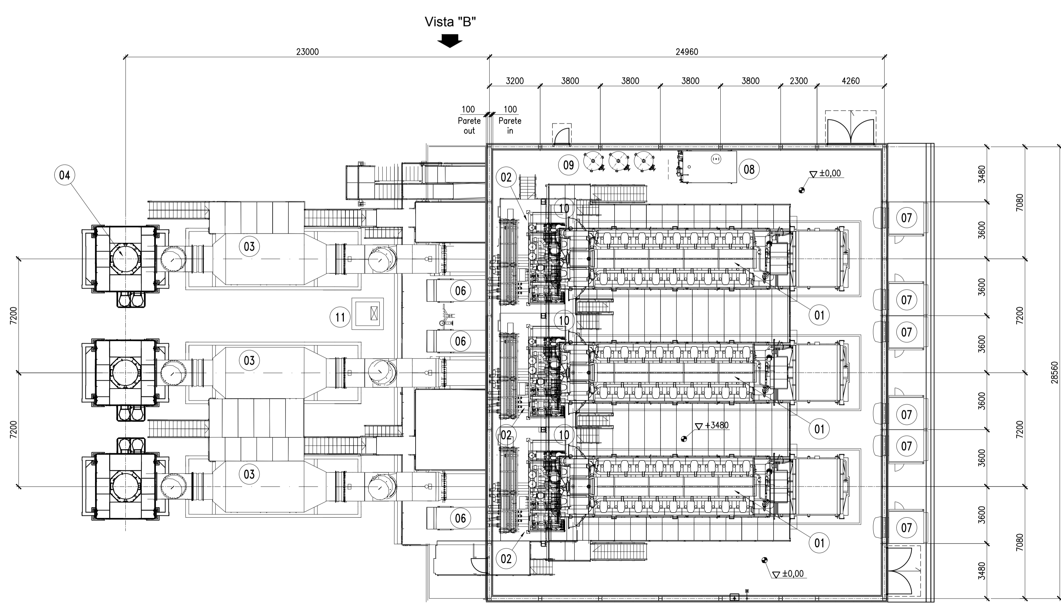
PLANIMETRIA SALA MACCHINE
