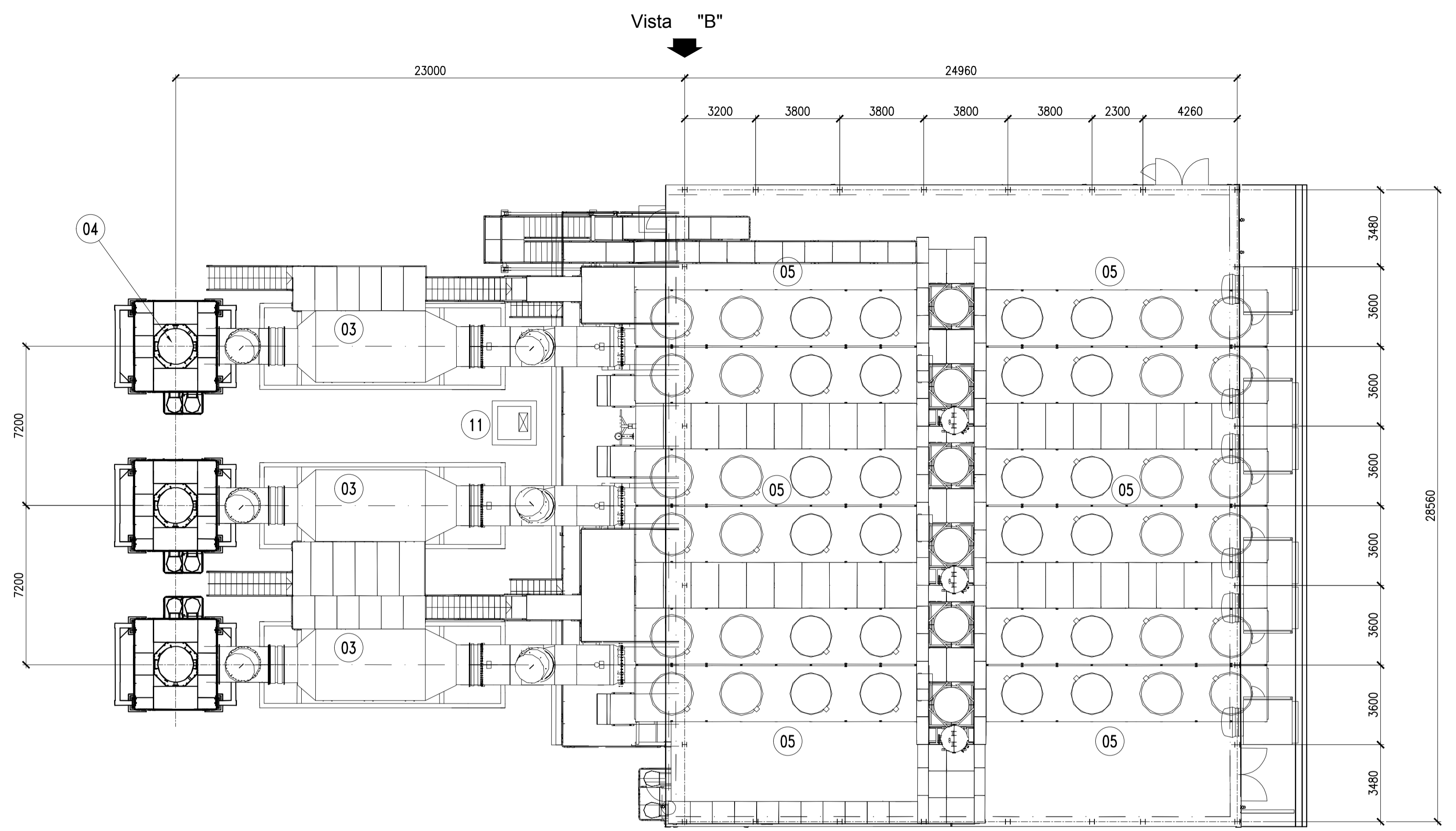
PLANIMETRIA QUOTA TETTO
