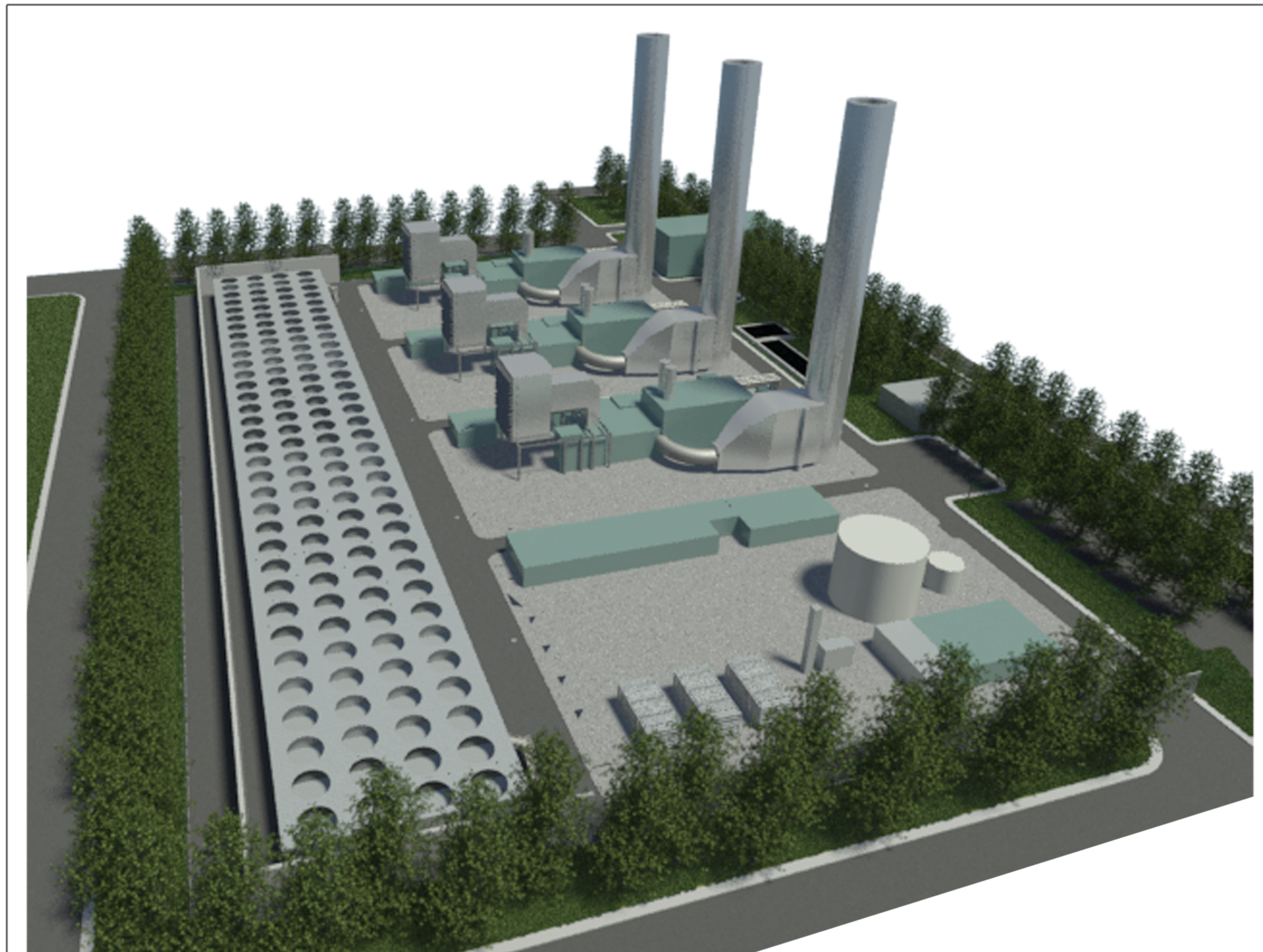
Modello 3D dell'impianto in progetto
