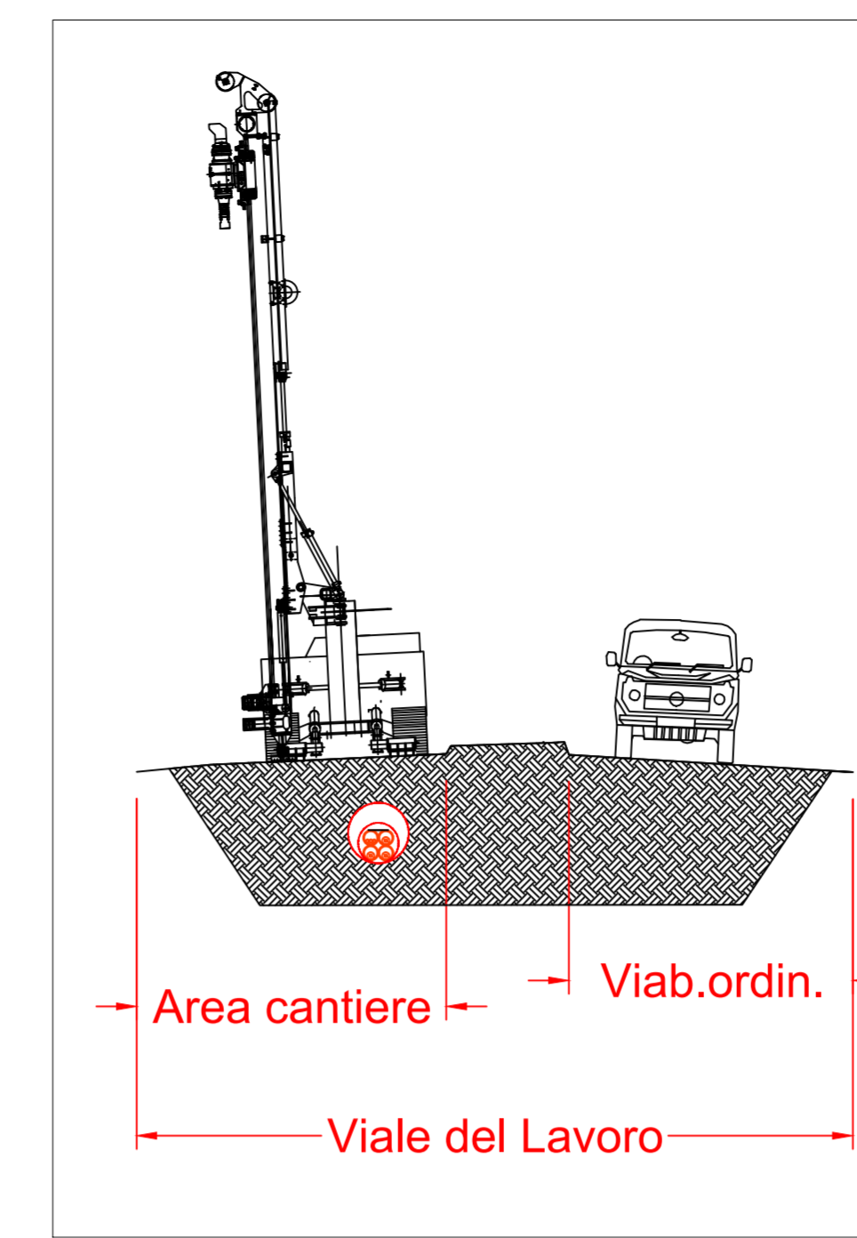
Sezioni Tipo
