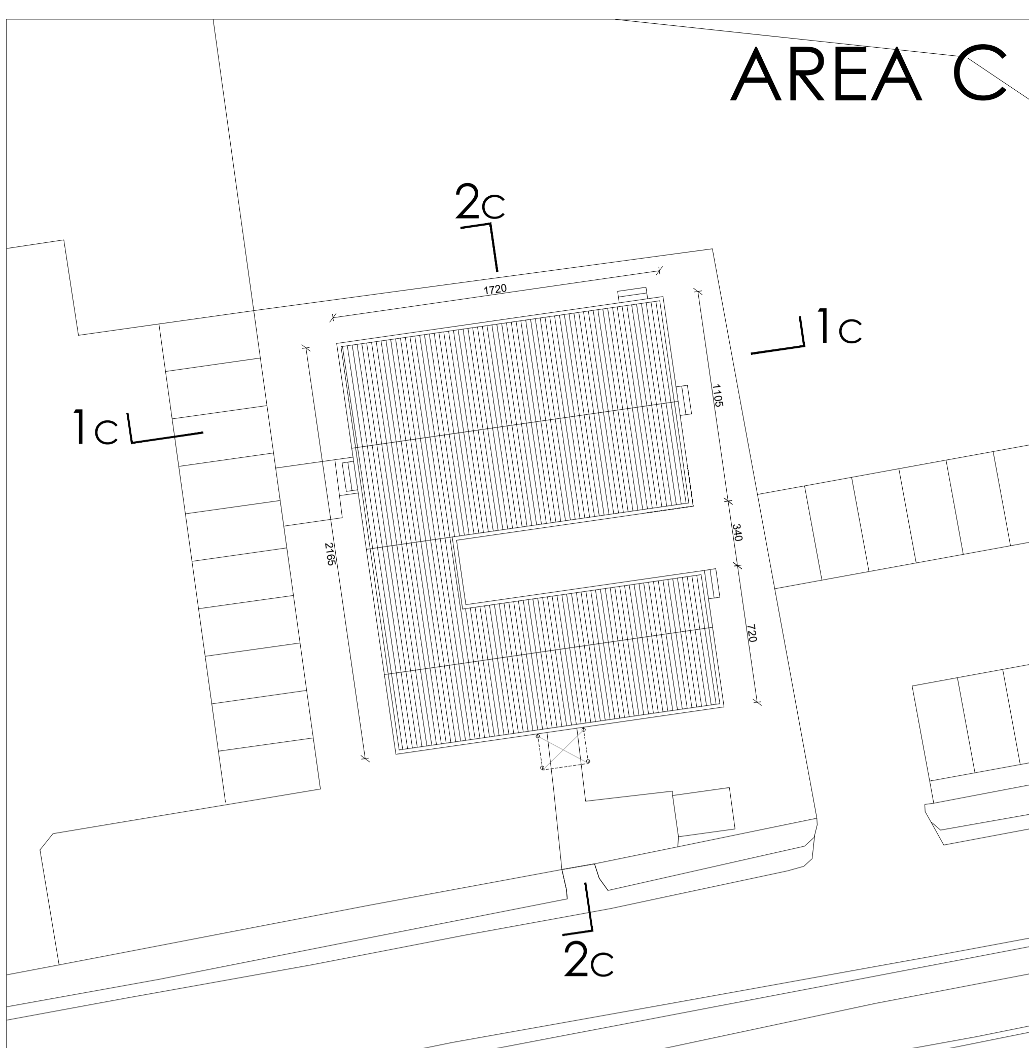
PIANTA COPERTURA 1:200
