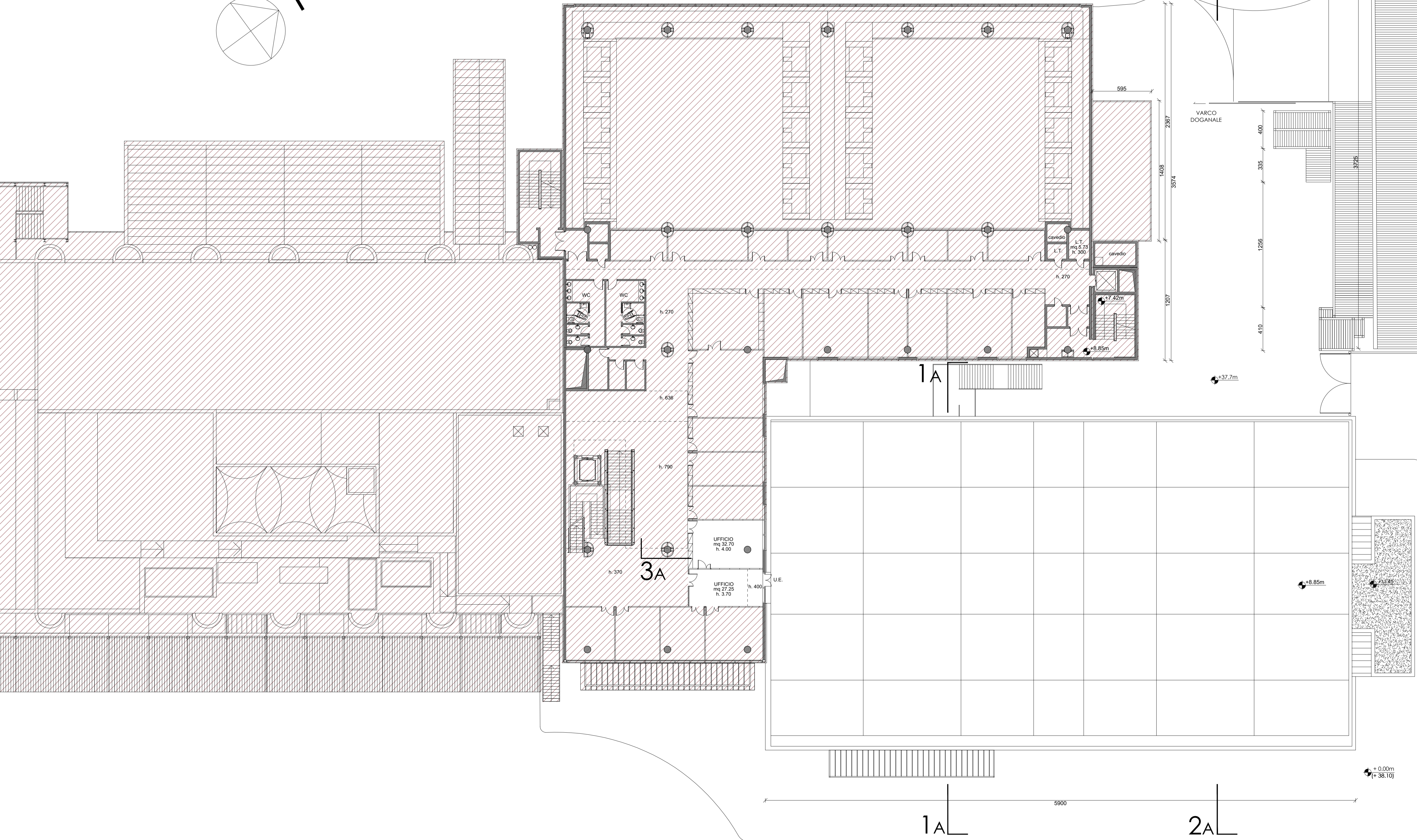
PIANTA PIANO SECONDO 1:200
