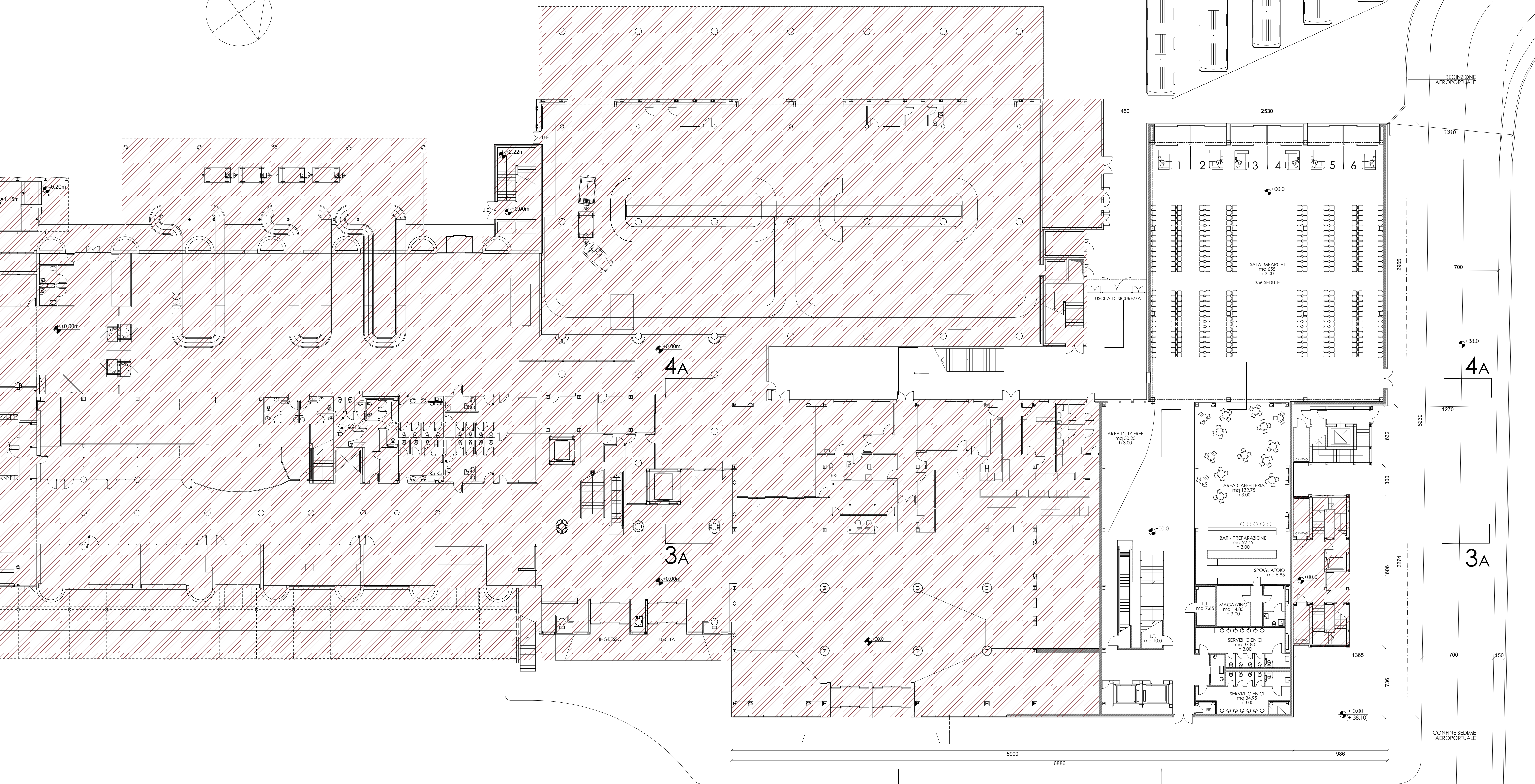
PIANTA PIANO TERRA 1:200
